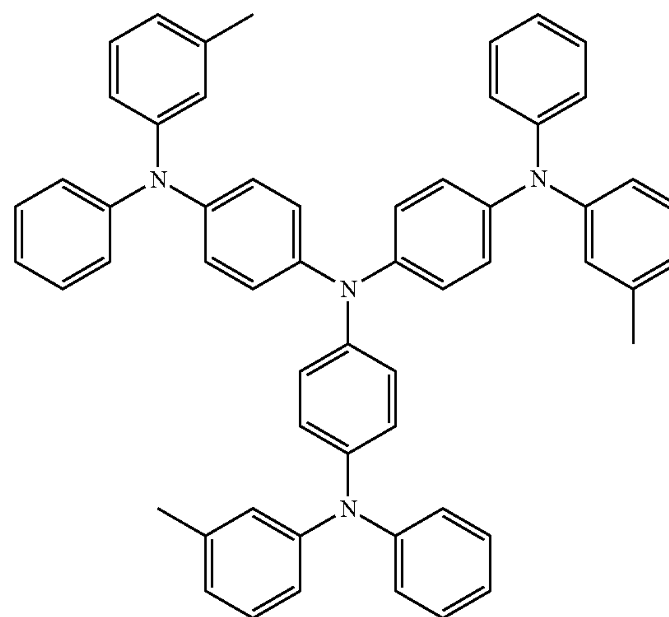
[n-TDATA]
