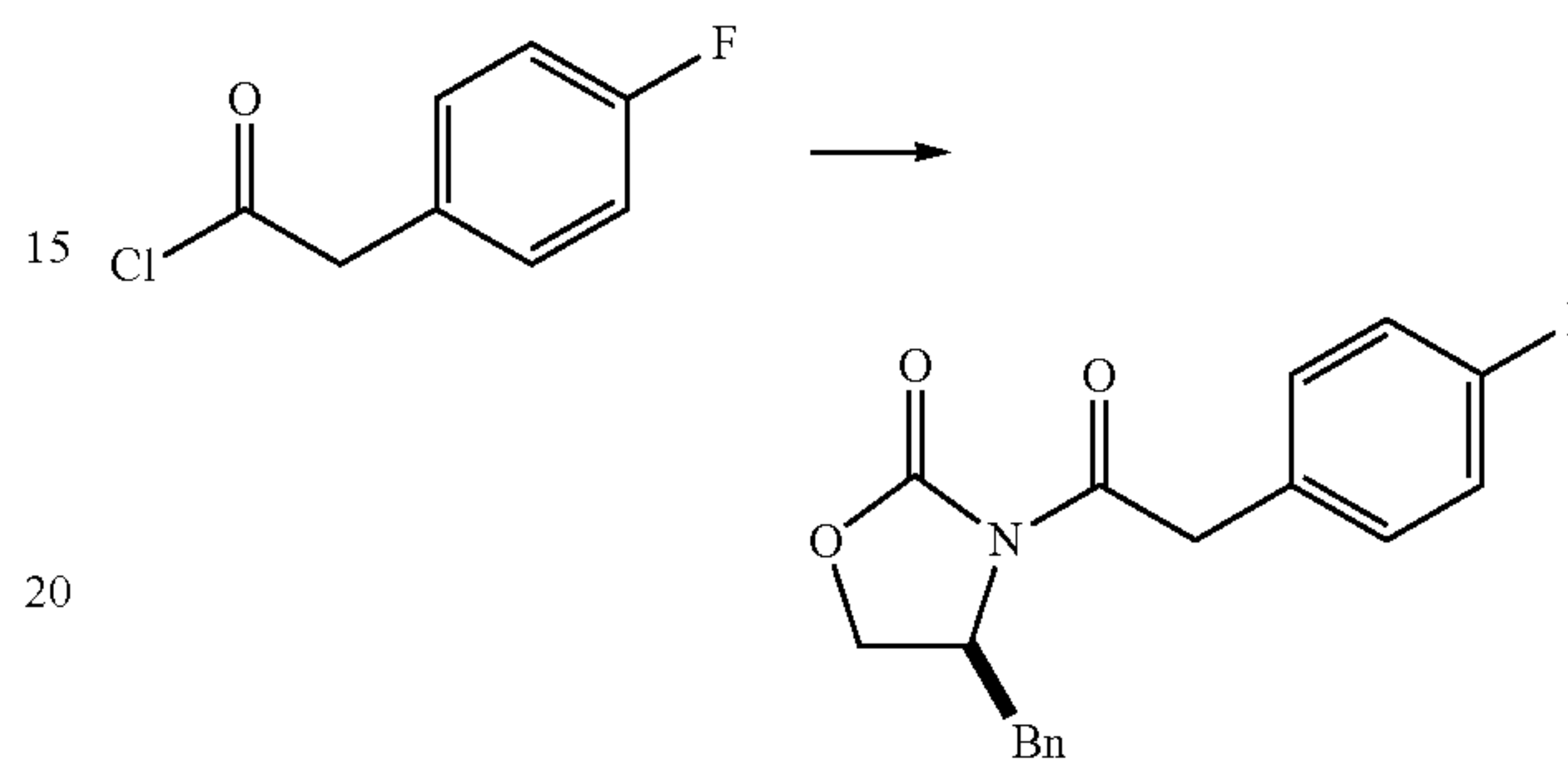
(S)-4-Benzyl-3-(2-(4-fluorophenyl)acetyl)oxazolidin-2-one
