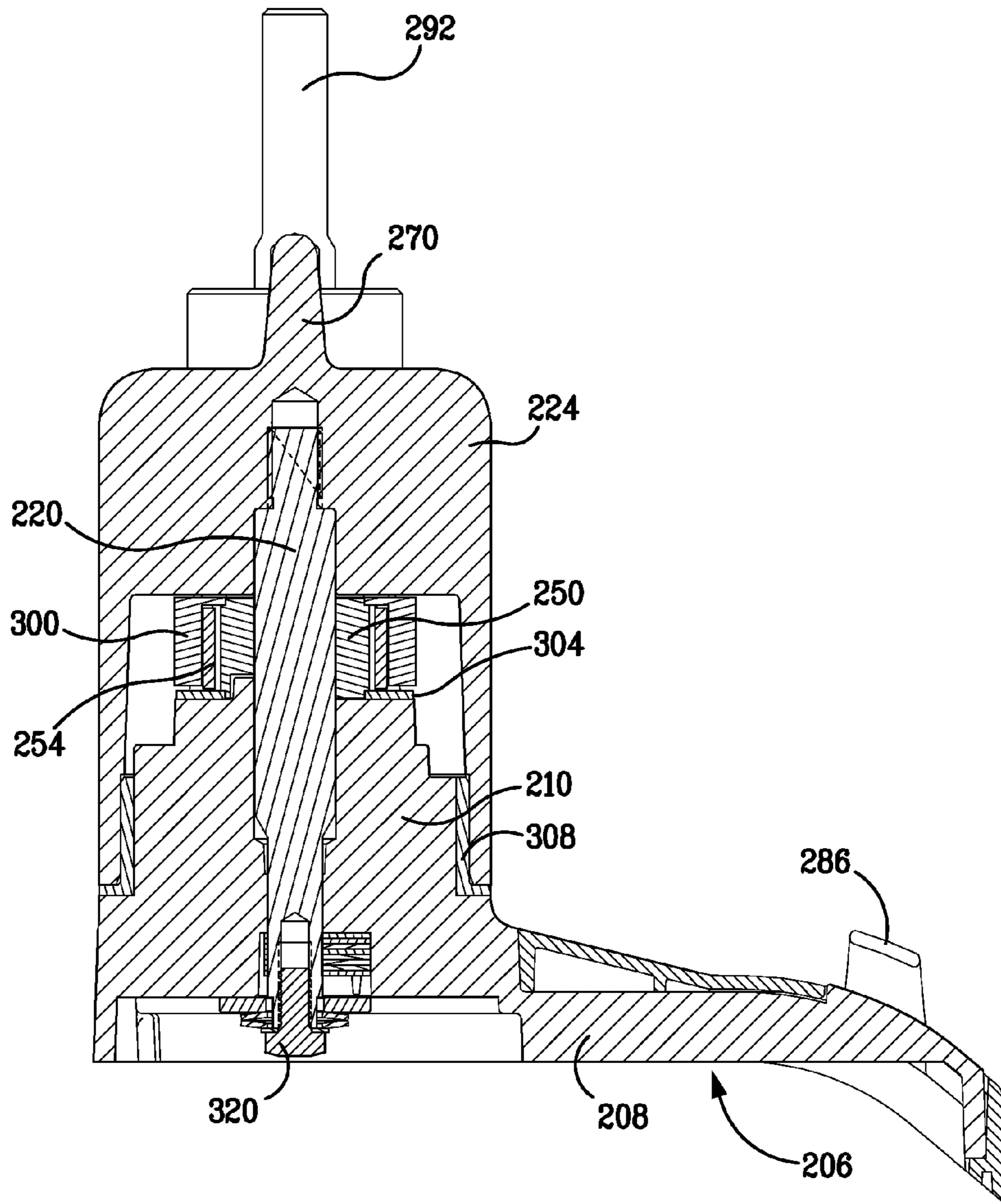
Section B-B FIG. 9
