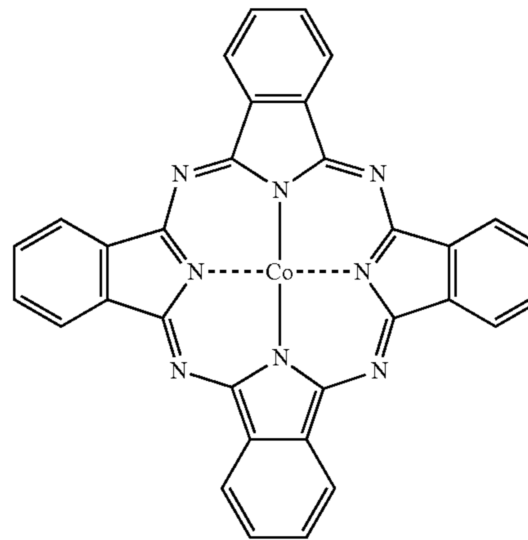
CoPc
