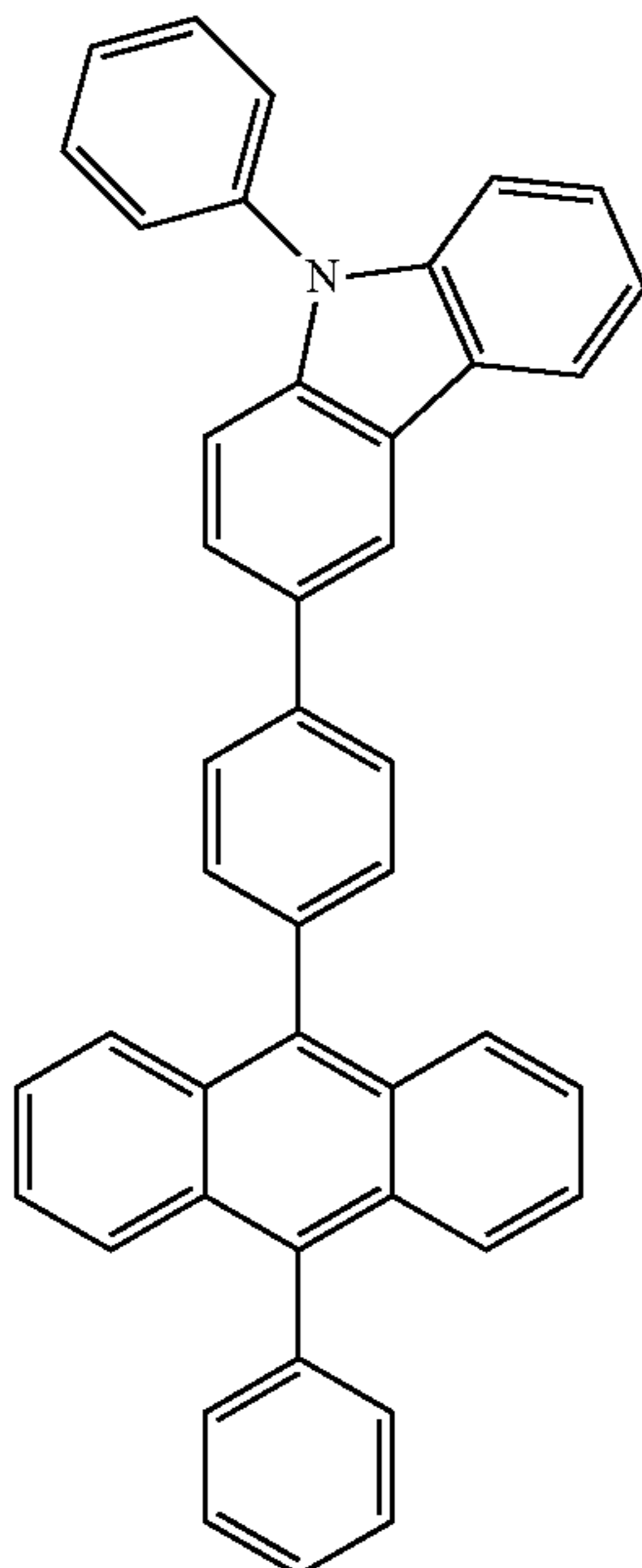
PCzPA
