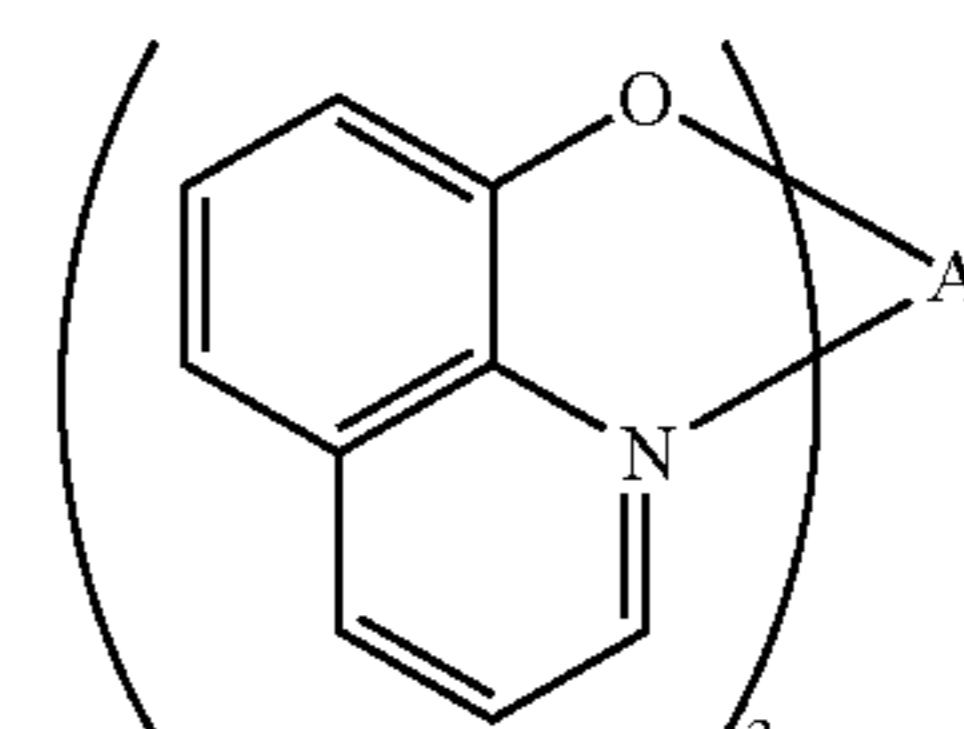
Alq
