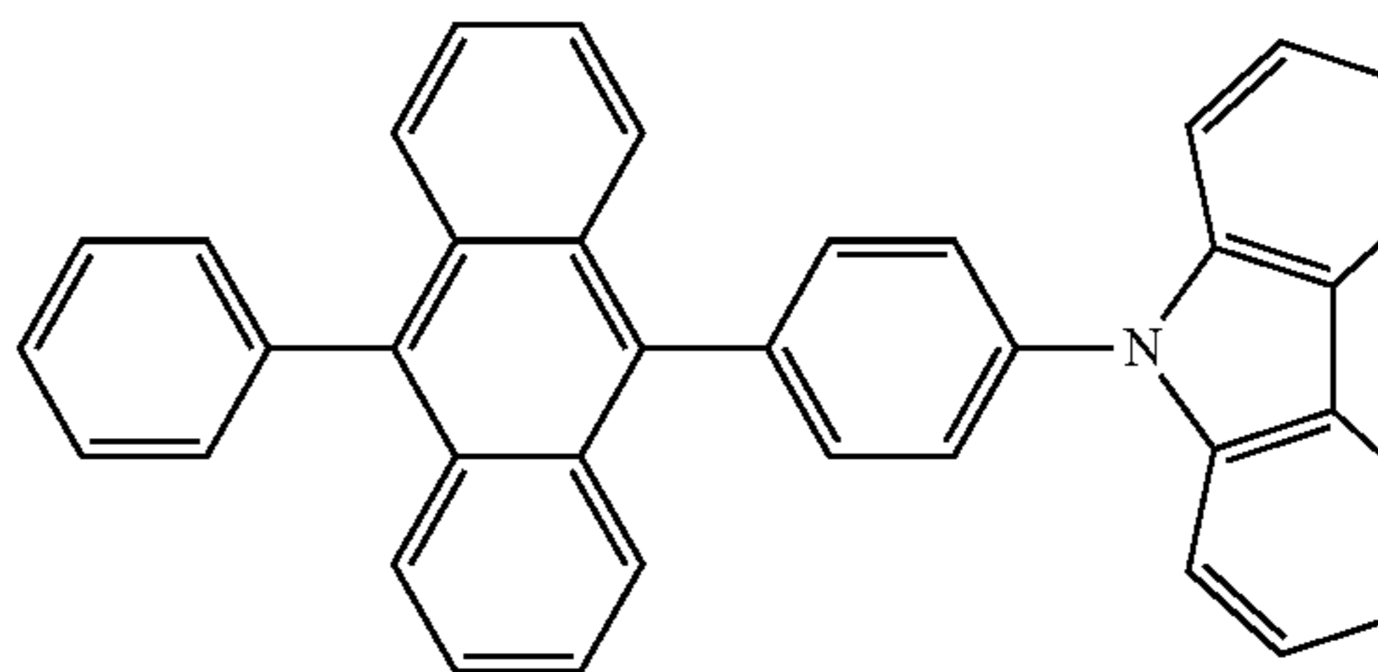
CzPA
