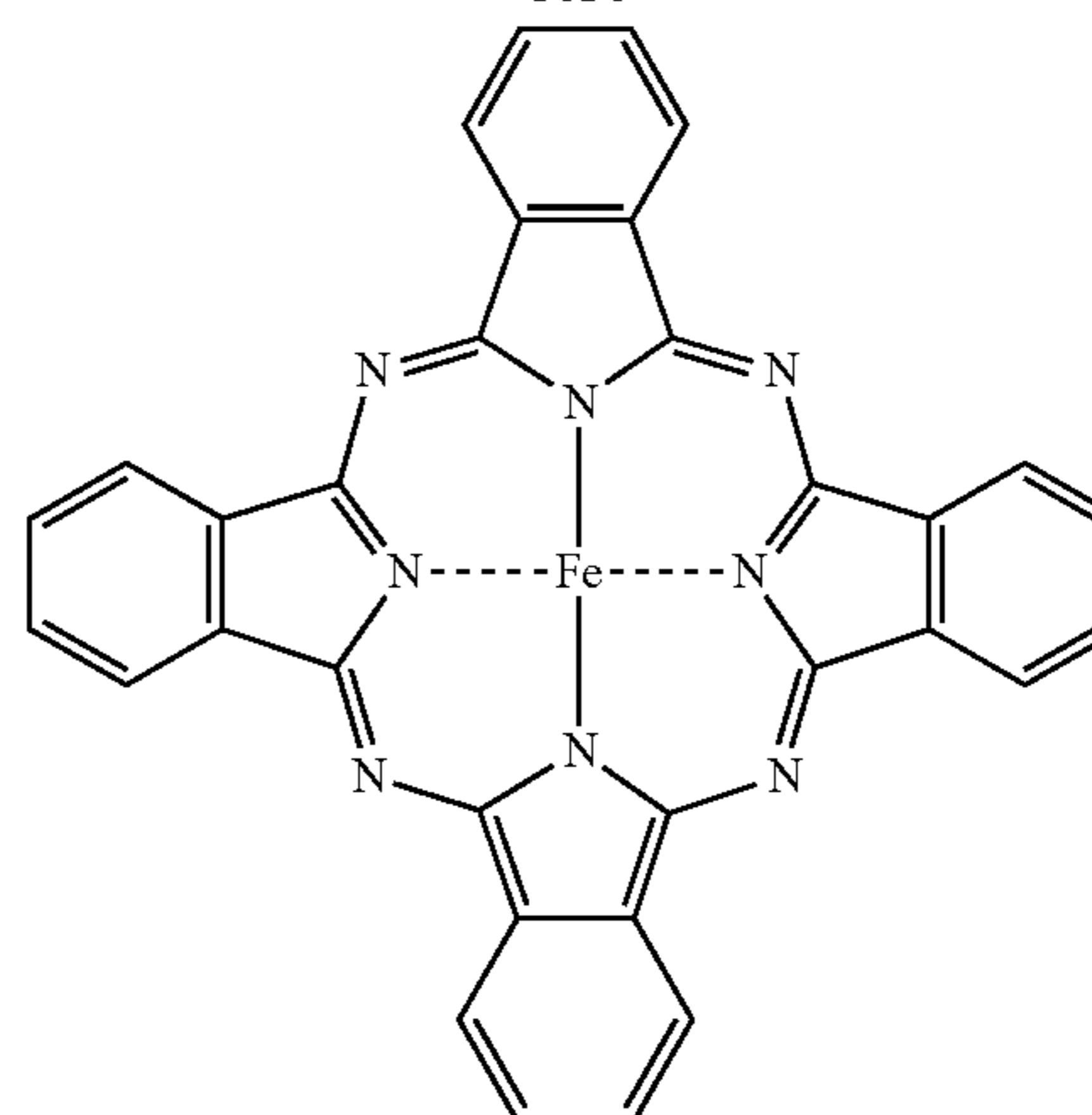
FePc
