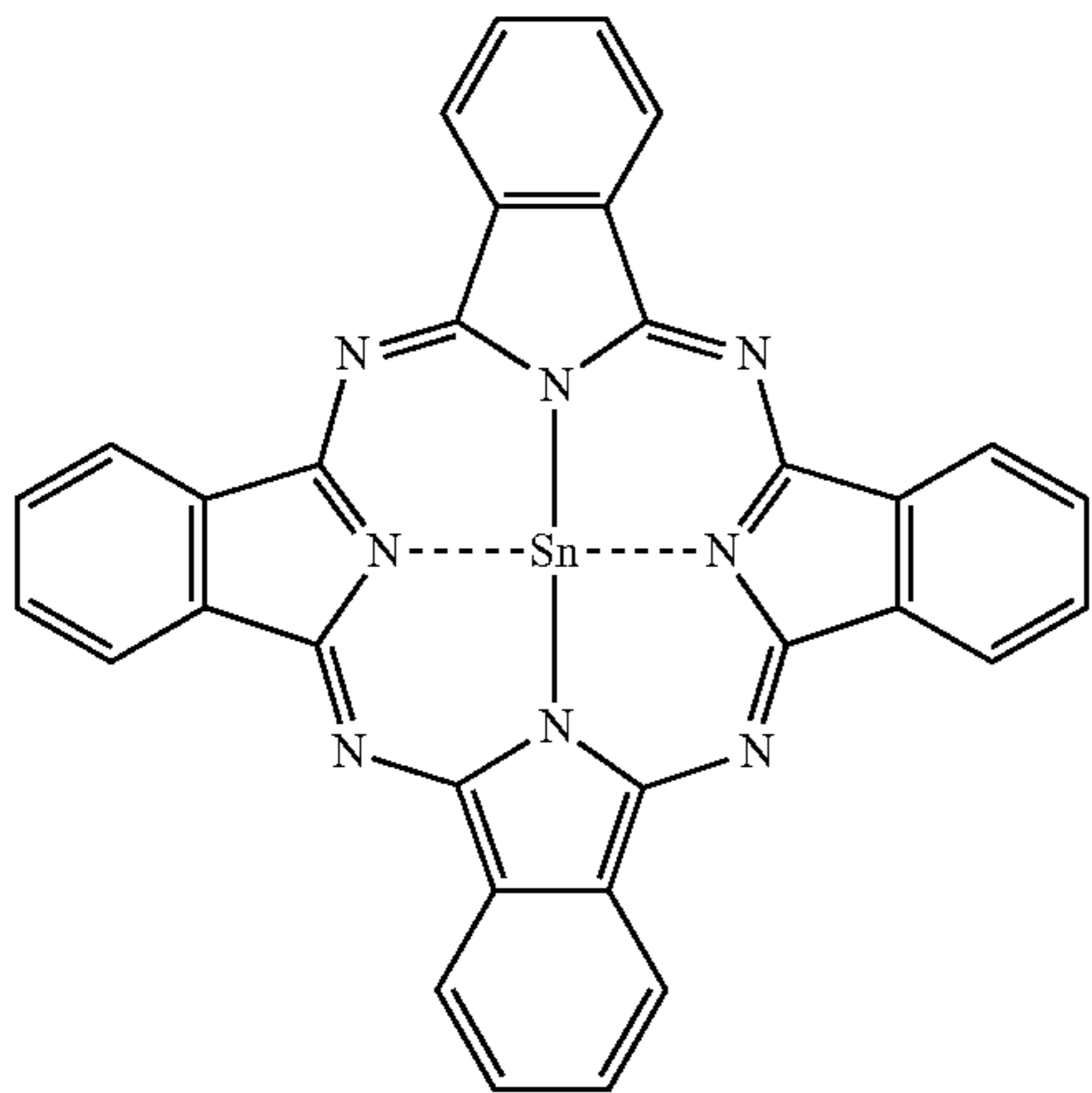
SnPc
