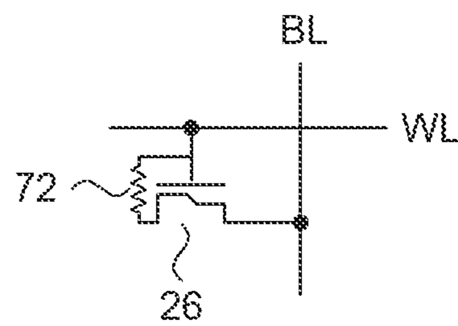
FIG. 8
