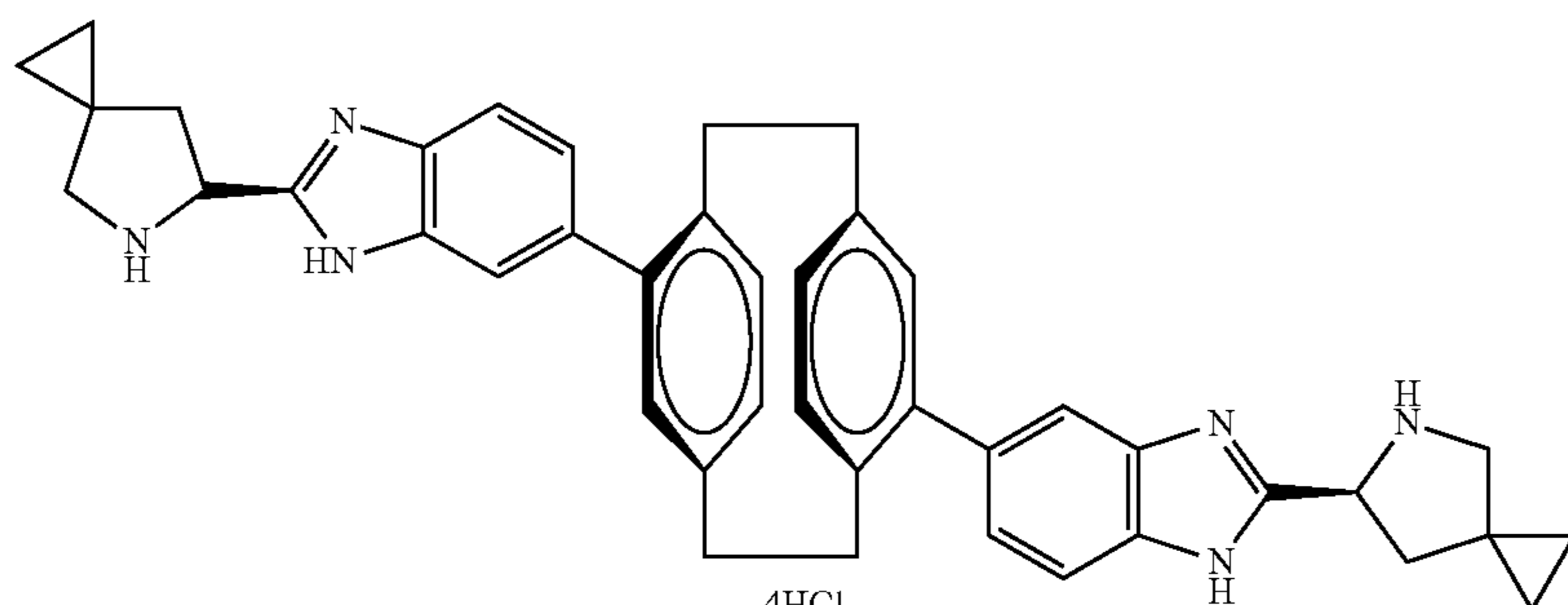
30 4HCl
