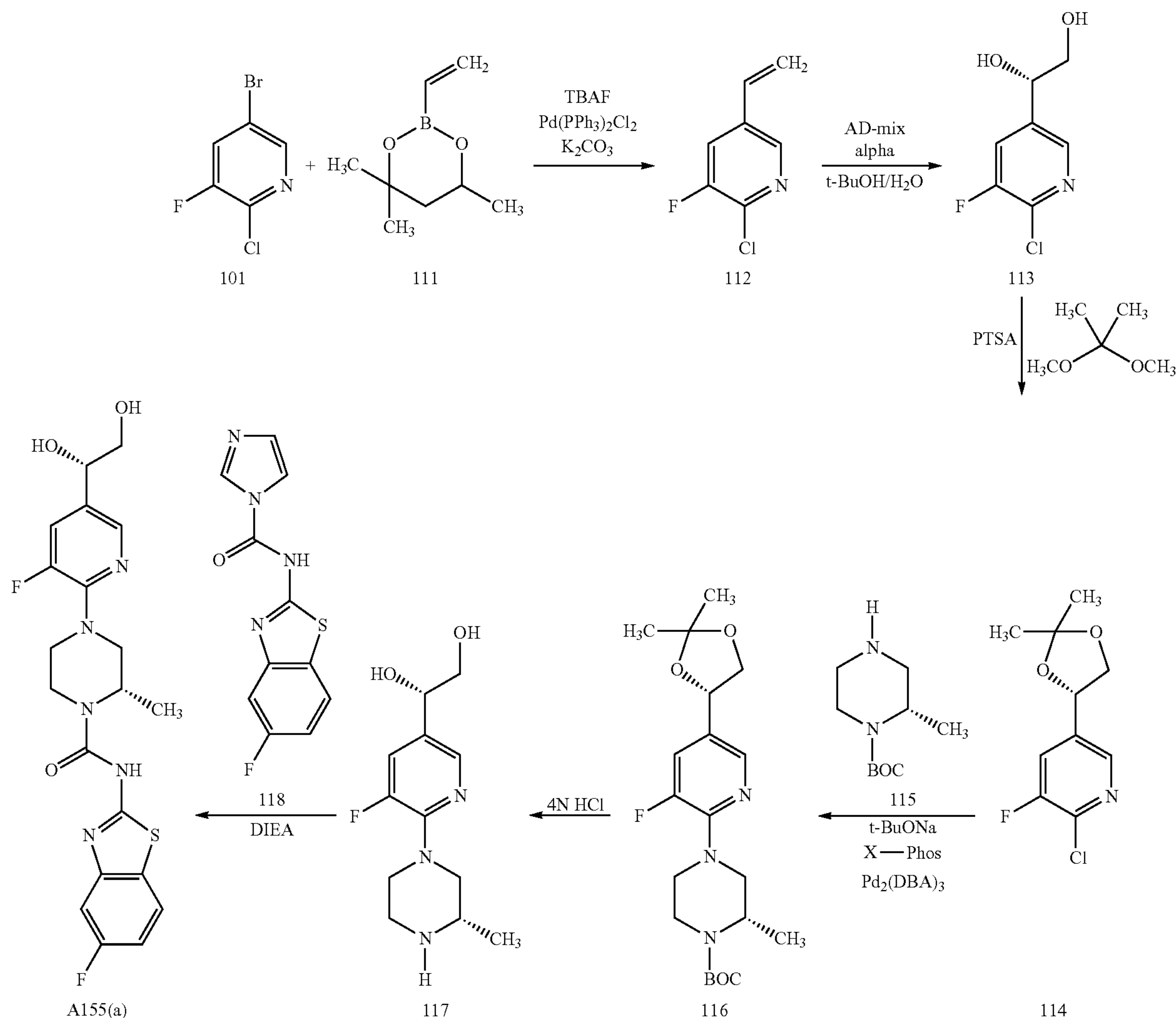
2-Chloro-3-fluoro-5-vinylpyridine (112)
