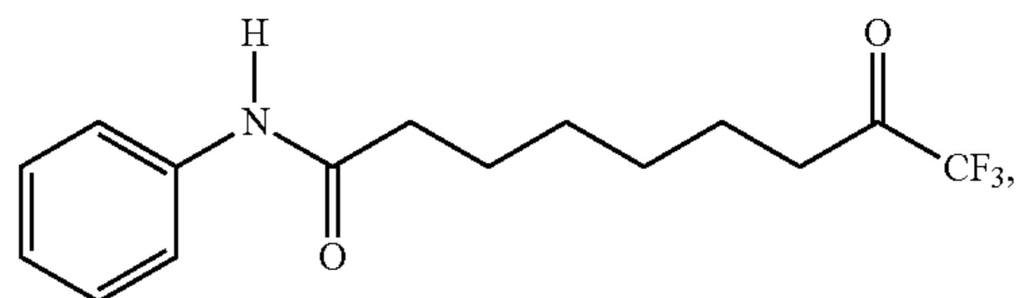
Trifluorométhyl cétone
