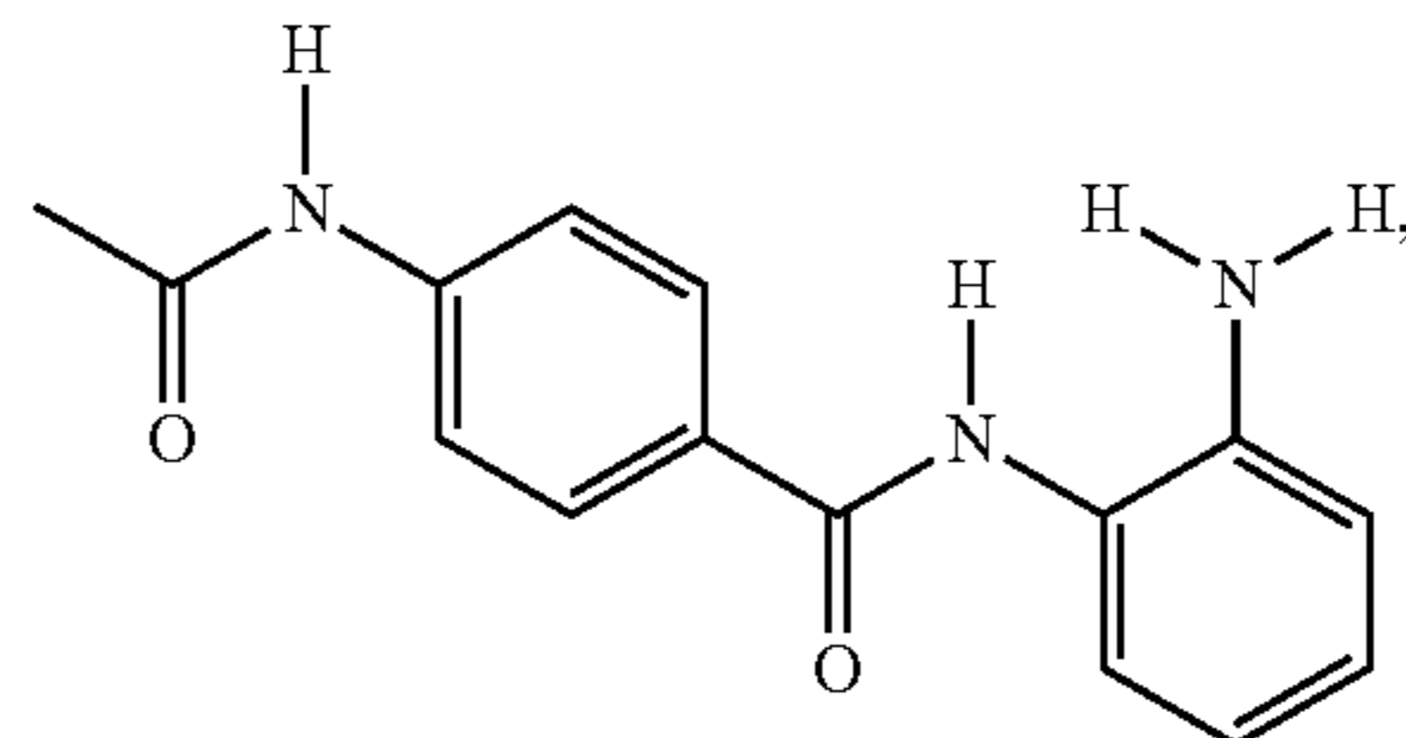
CI-994
