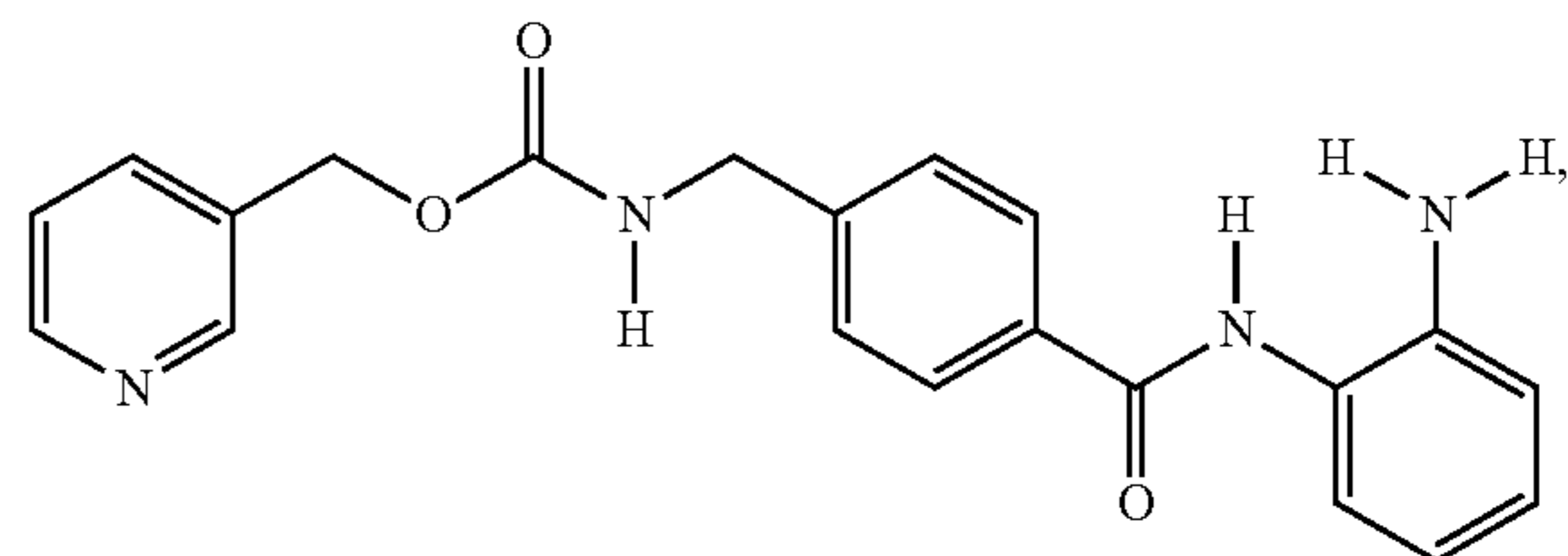
MS-275
