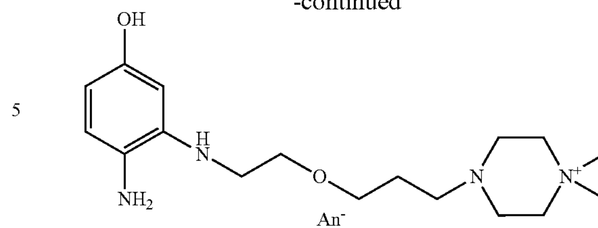
4-(3-{2-[(2-amino-5-hydroxyphenyl)amino]ethoxy}propyl)-1,1-dimethylpiperazin-1-ium, An -
