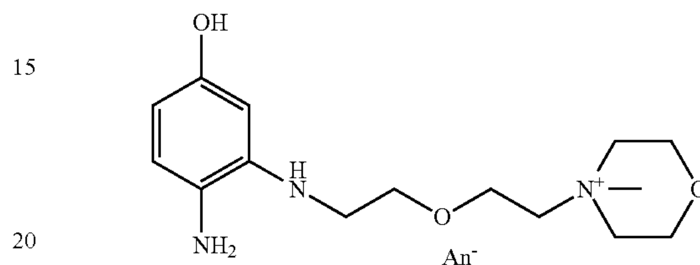
4-(3-{2-[(2-amino-5-hydroxyphenyl)amino]ethoxy}propyl)-1,1-dimethylpiperazin-1-ium, An -
