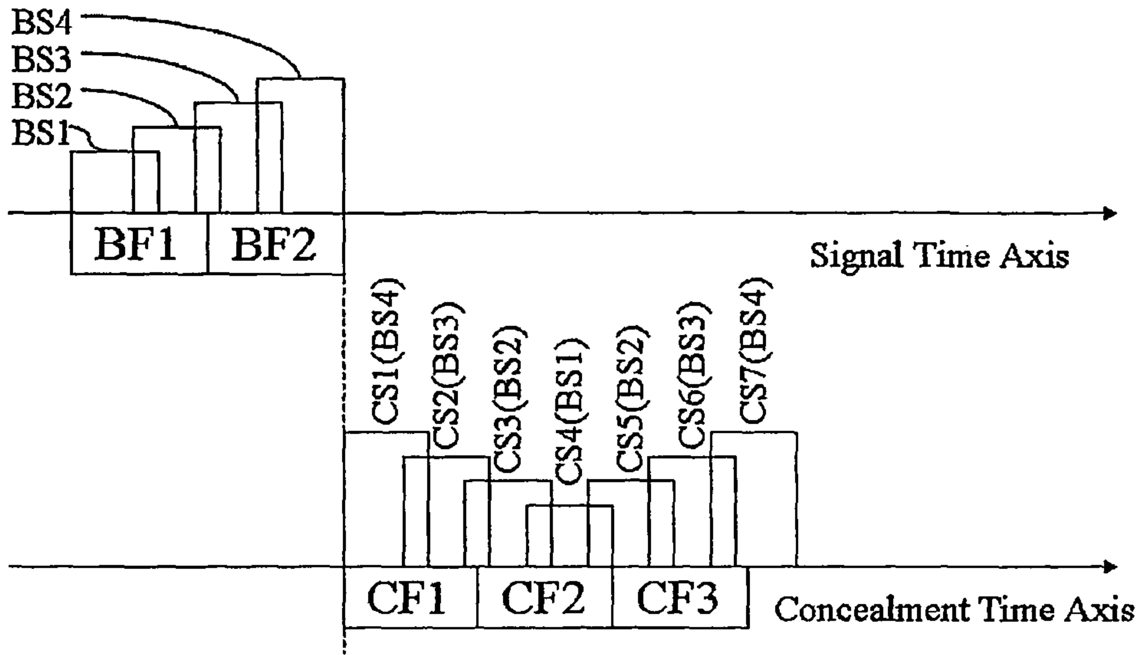
Fig. 5A
