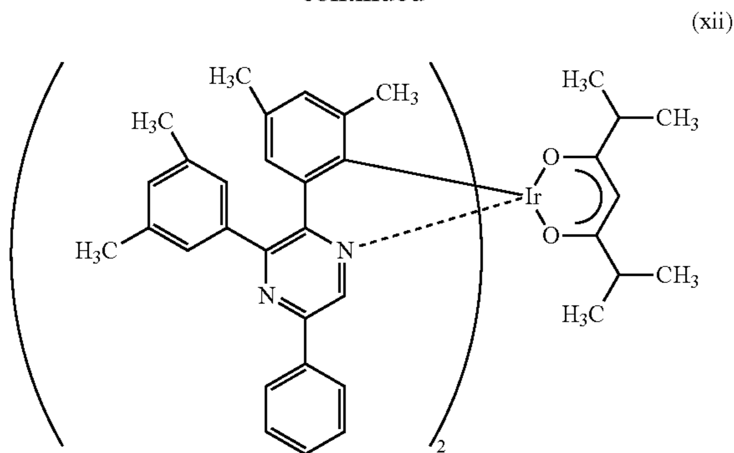
Ir(dmdppr-P) 2 (dibm)
