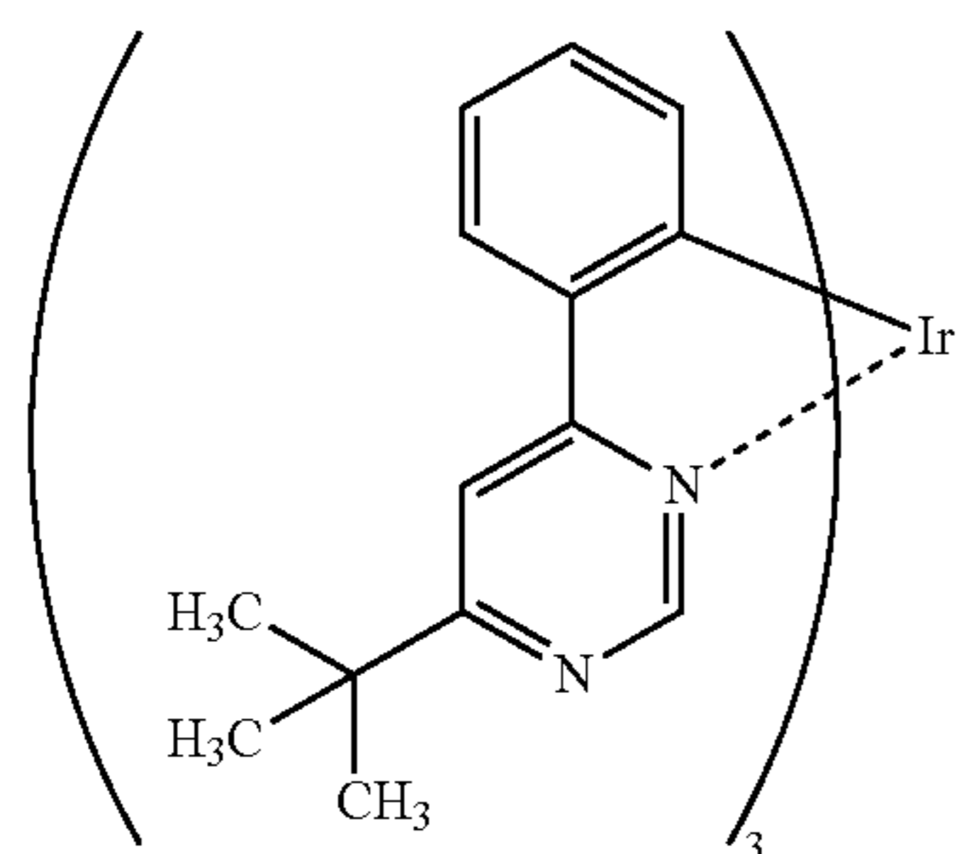
Ir(tBuppm) 3
