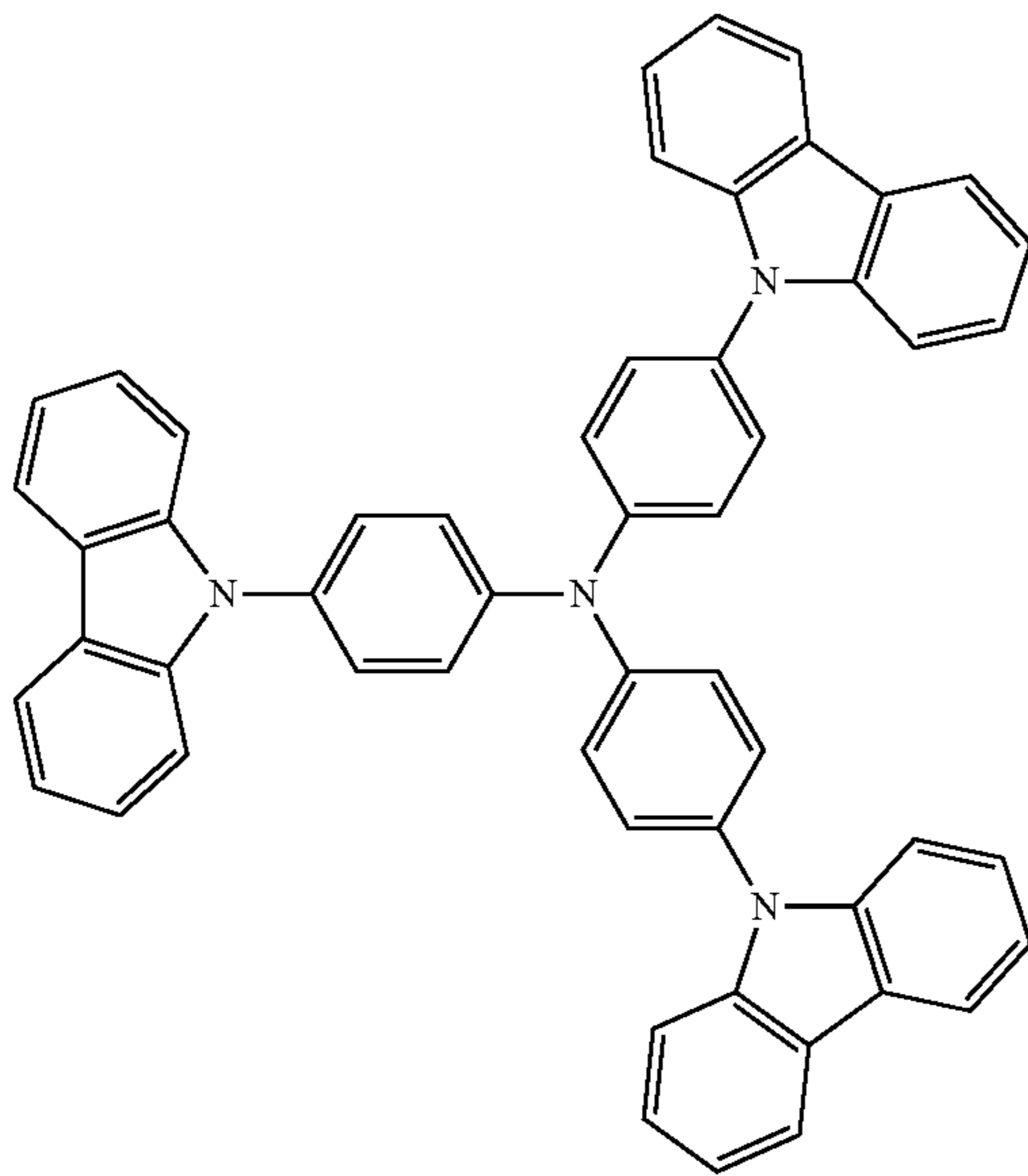
TCTA
