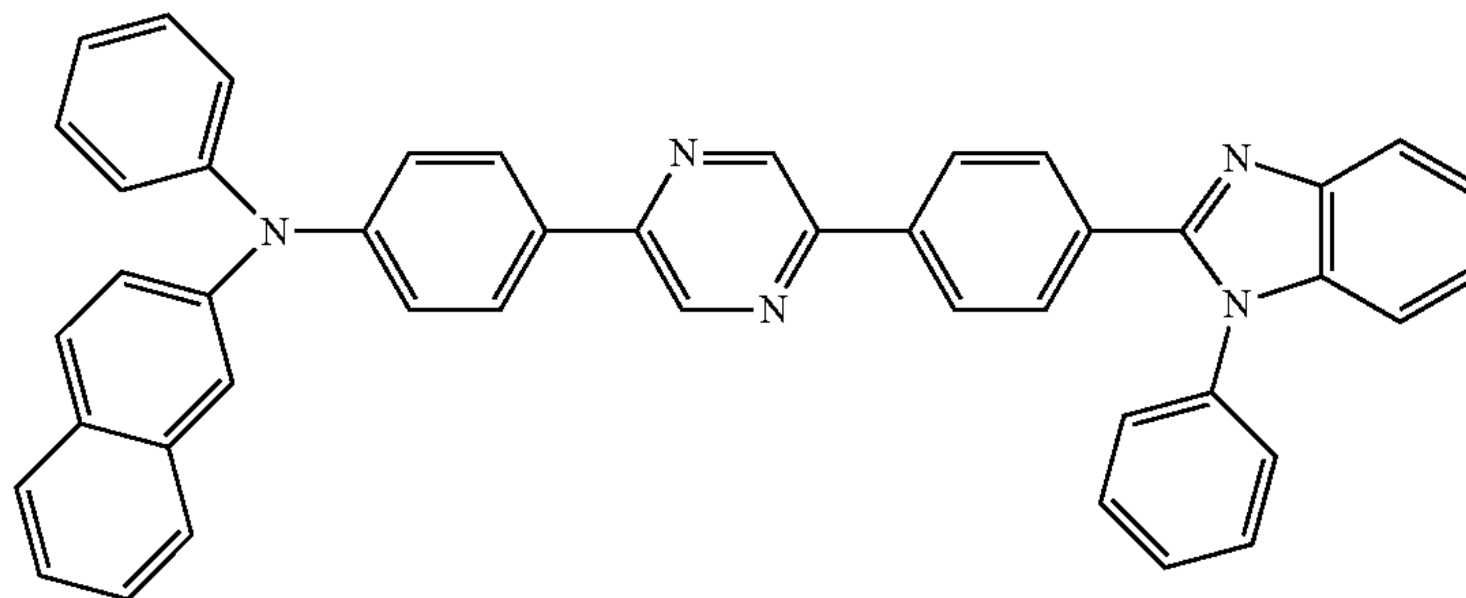
N-phenyl-N-(4-(5-(4-(1-phenyl-1H-benzo[d]imidazol-2-yl)phenyl)pyrazin-2-yl)phenyl)naphthalen-2-amine
