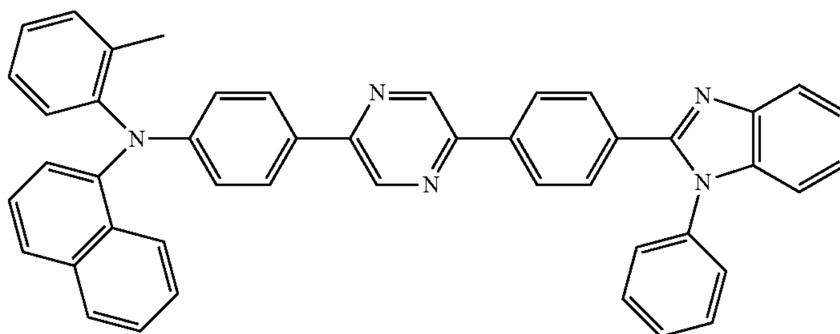
N-(4-(5-(4-(1-phenyl-1H-benzo[d]imidazol-2-yl)phenyl)pyrazin-2-yl)phenyl)-N-(o-tolyl)naphthalen-1-amine
