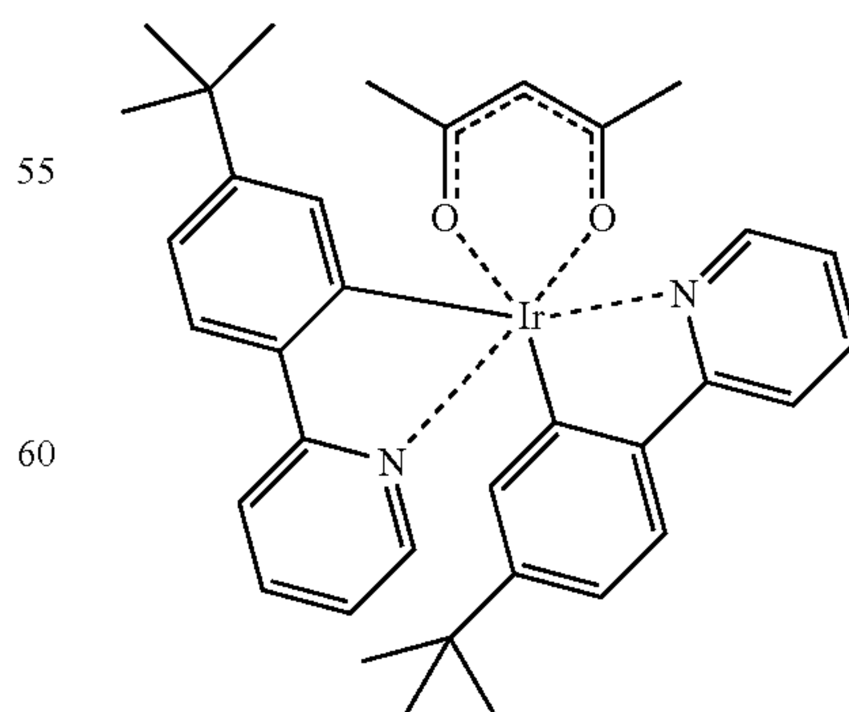
Ir(t-Buppy) 2 (acac)
