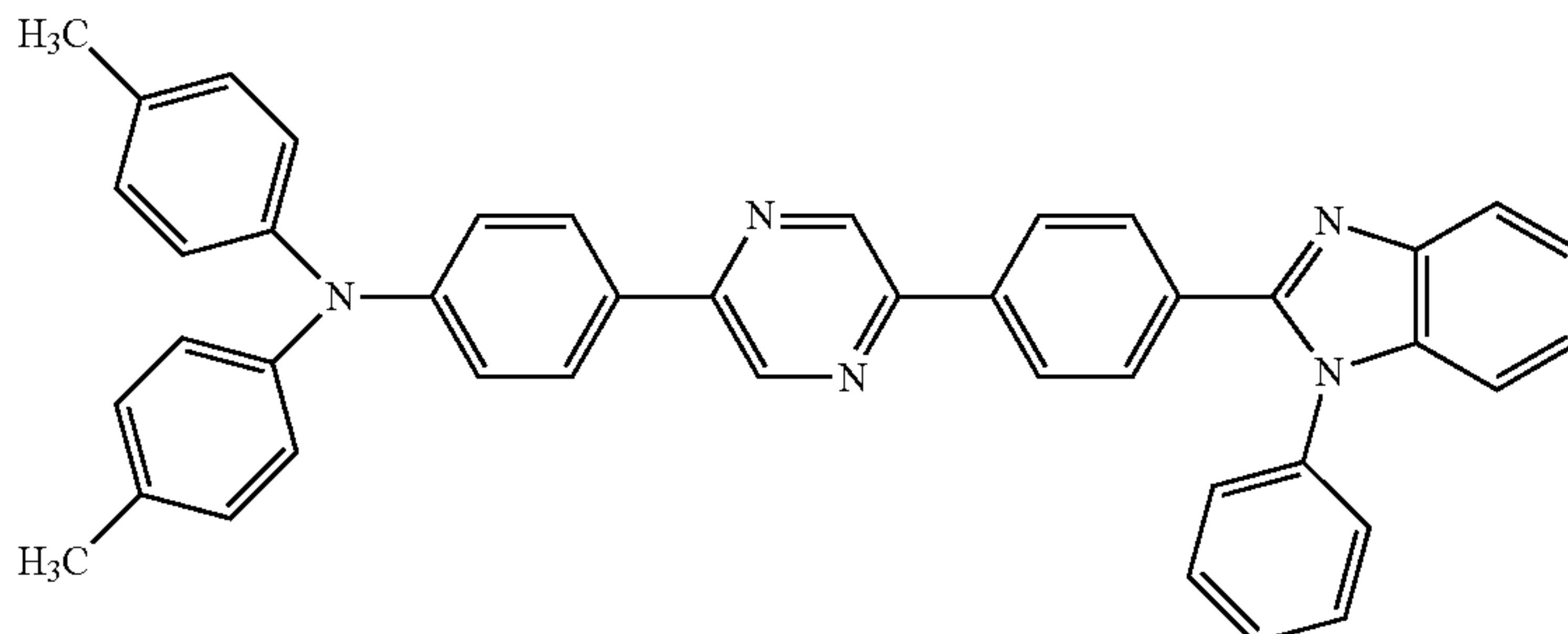
4-methyl-N-(4-(5-(4-(1-phenyl-1H-benzo[d]imidazol-2-yl)phenyl)pyrazin-2-yl)phenyl)-N-(p-tolyl)aniline
