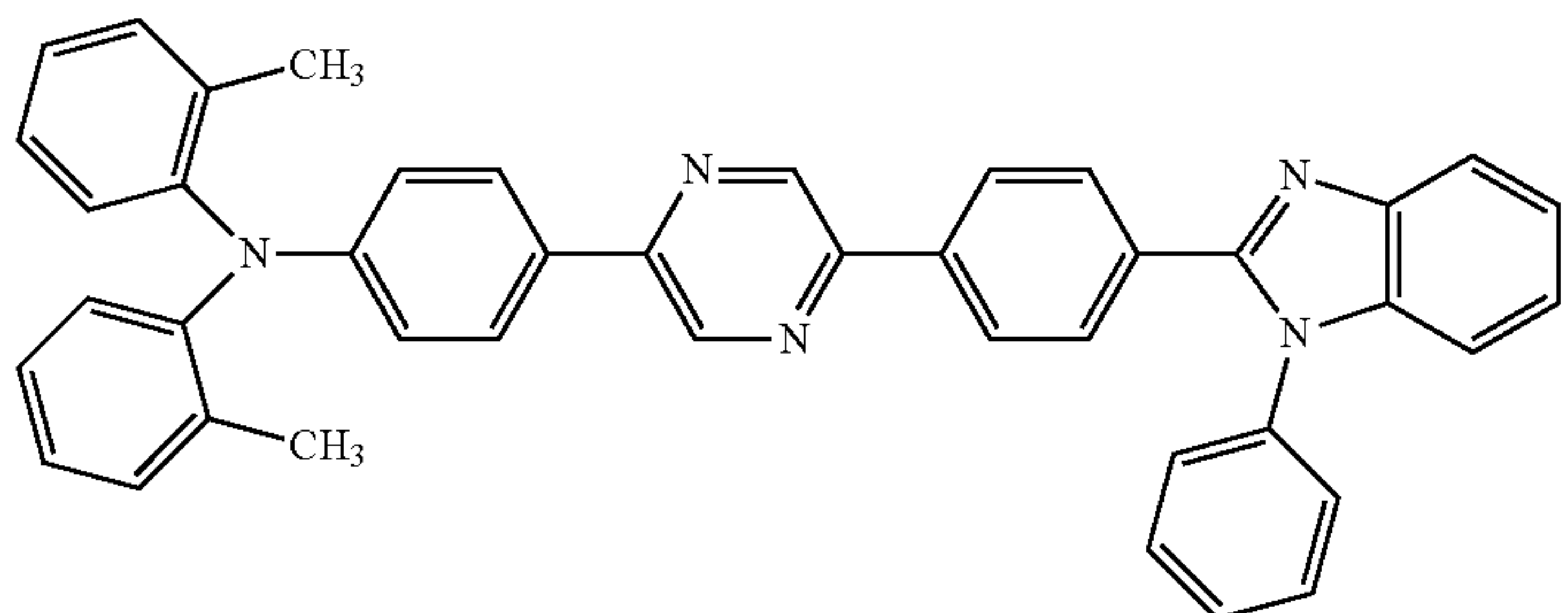
2-methyl-N-(4-(5-(4-(1-phenyl-1H-benzo[d]imidazol-2-yl)phenyl)pyrazin-2-yl)phenyl)-N-(o-tolyl)aniline
