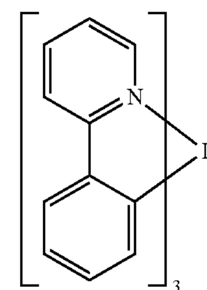
Ir(ppy) 3
