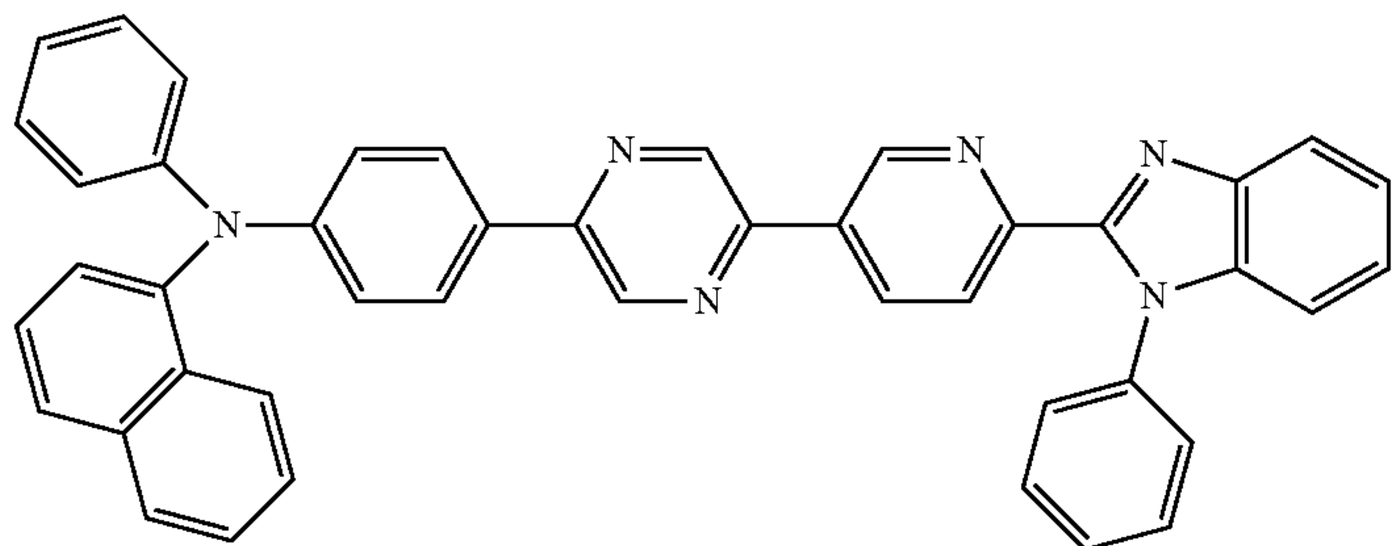
N-phenyl-N-(4-(5-(6-(1-phenyl-1H-benzo[d]imidazol-2-yl)pyridin-3-yl)pyrazine-2-yl)phenyl)naphthalen-1-amine
