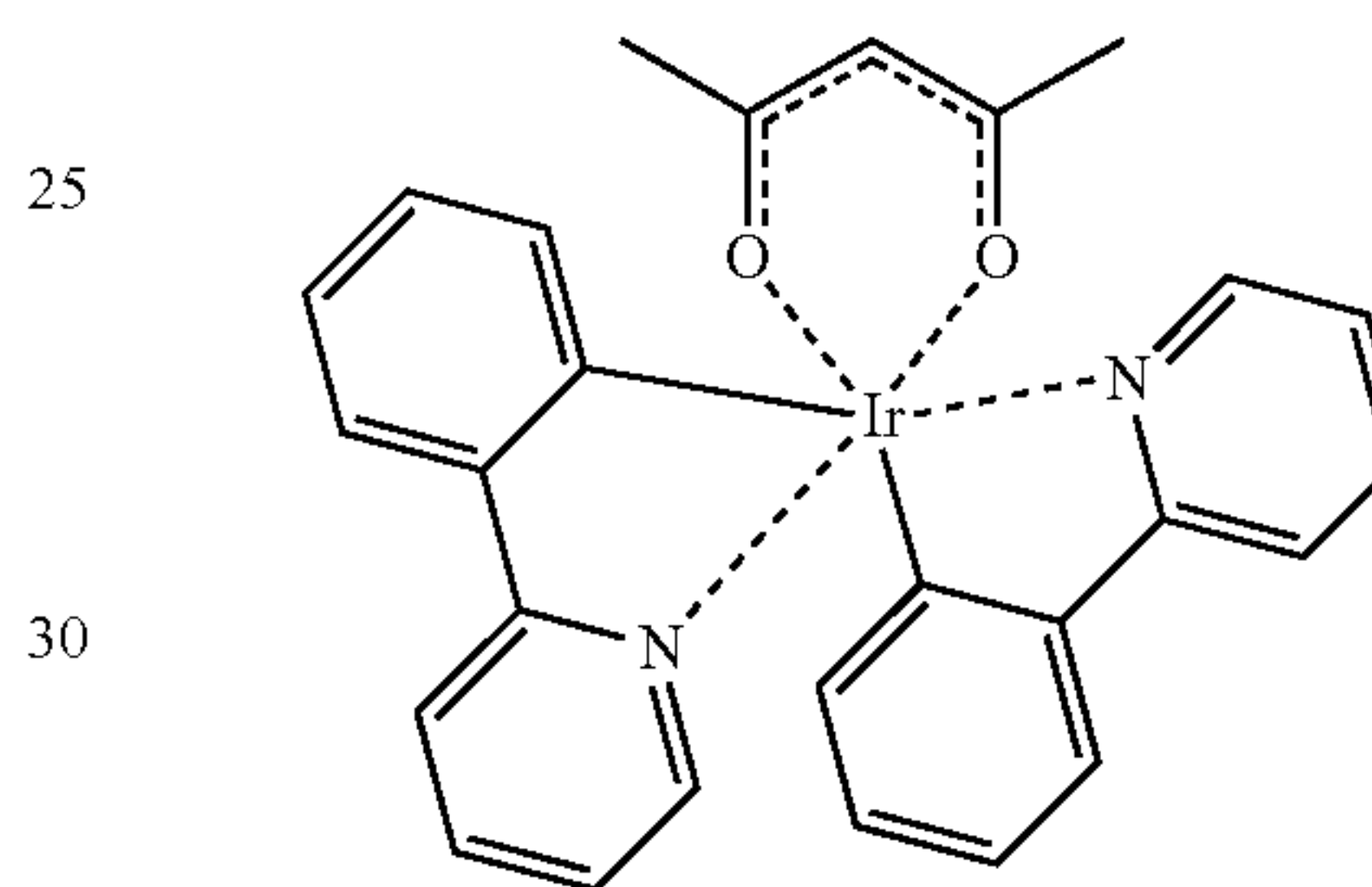
Ir(ppy) 2 (acac)
