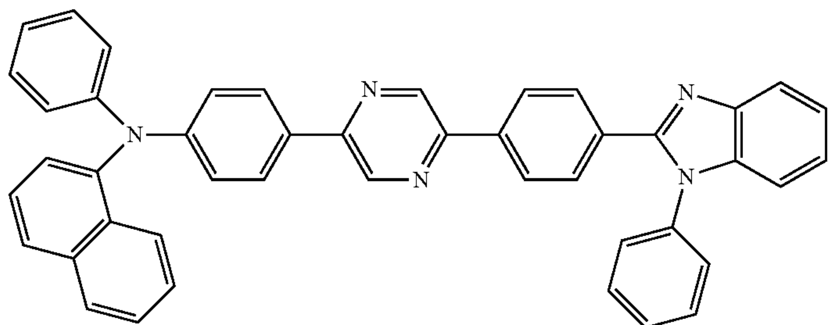
N-phenyl-N-(4-(5-(6-(1-phenyl-1H-benzo[d]imidazol-2-yl)phenyl)pyrazine-2-yl)phenyl)naphthalen-1-amine
