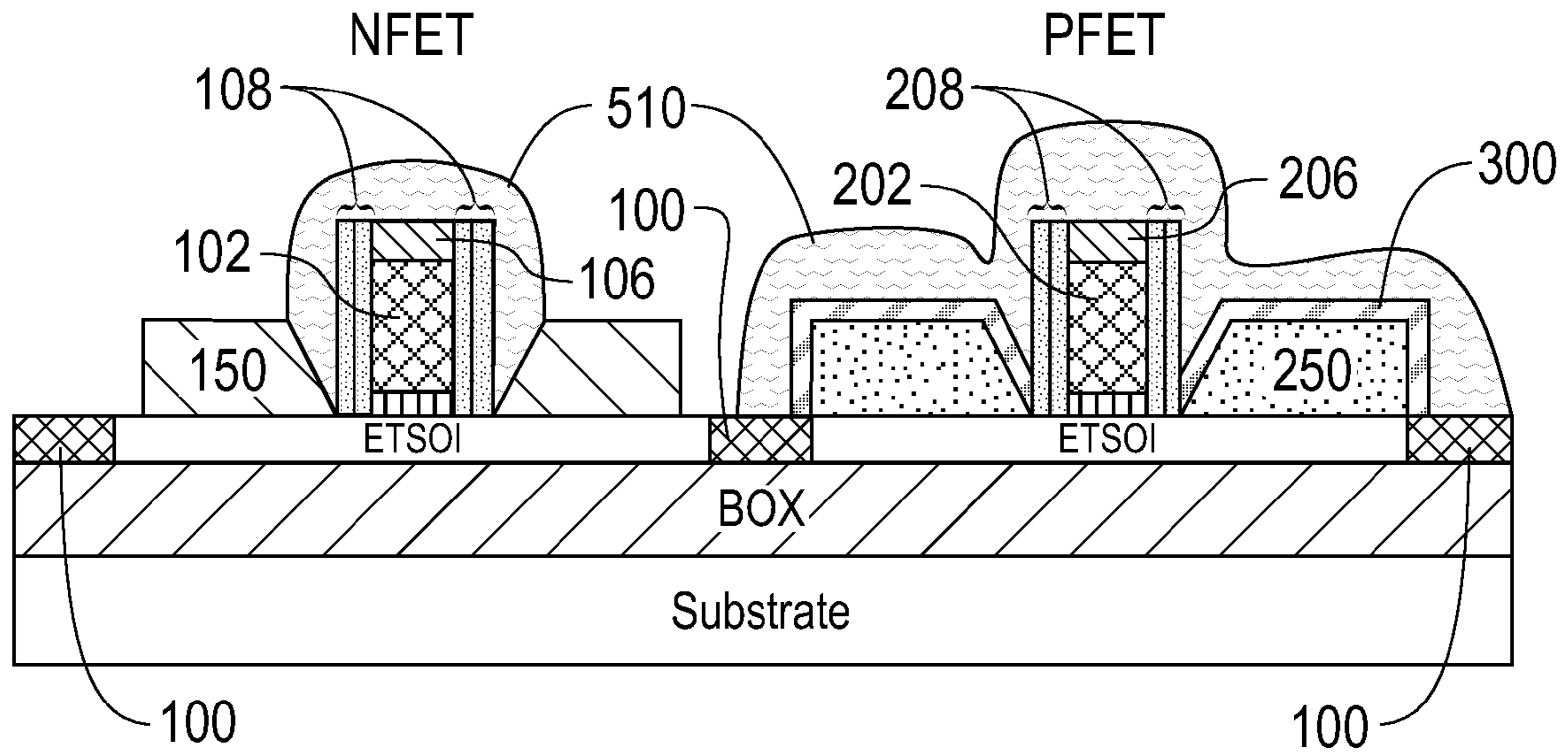
FIG. 5C
