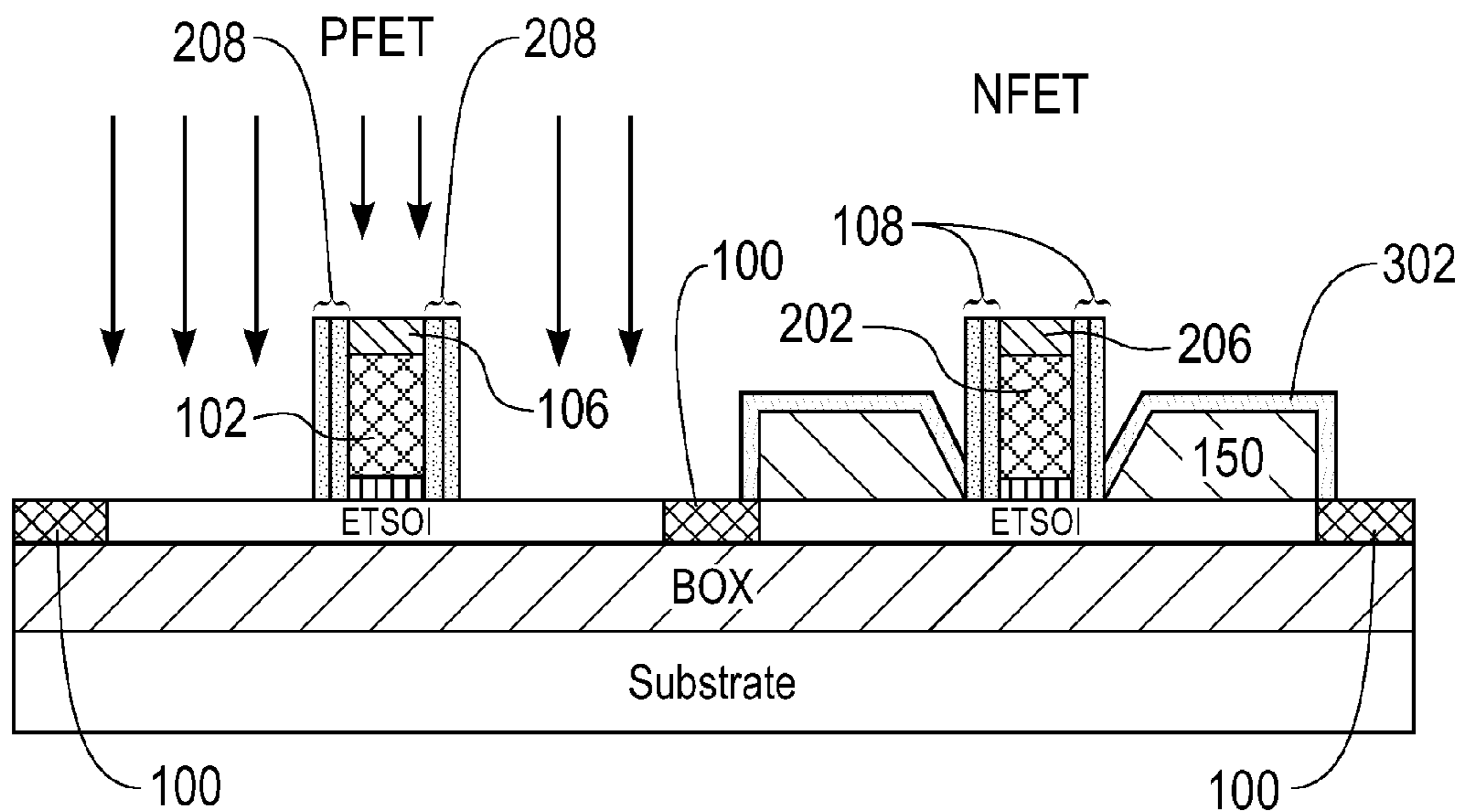
FIG. 4C
