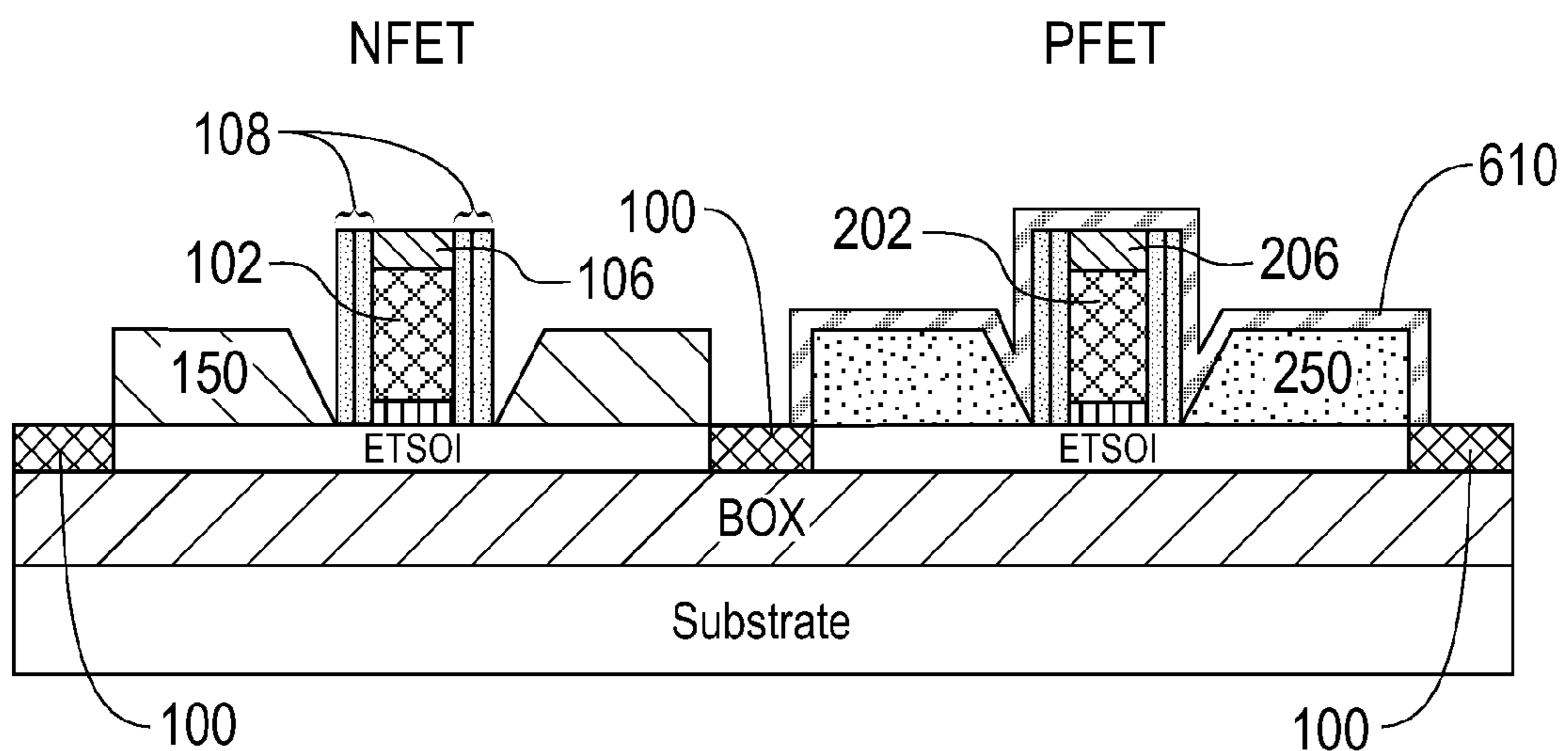
FIG. 6D
