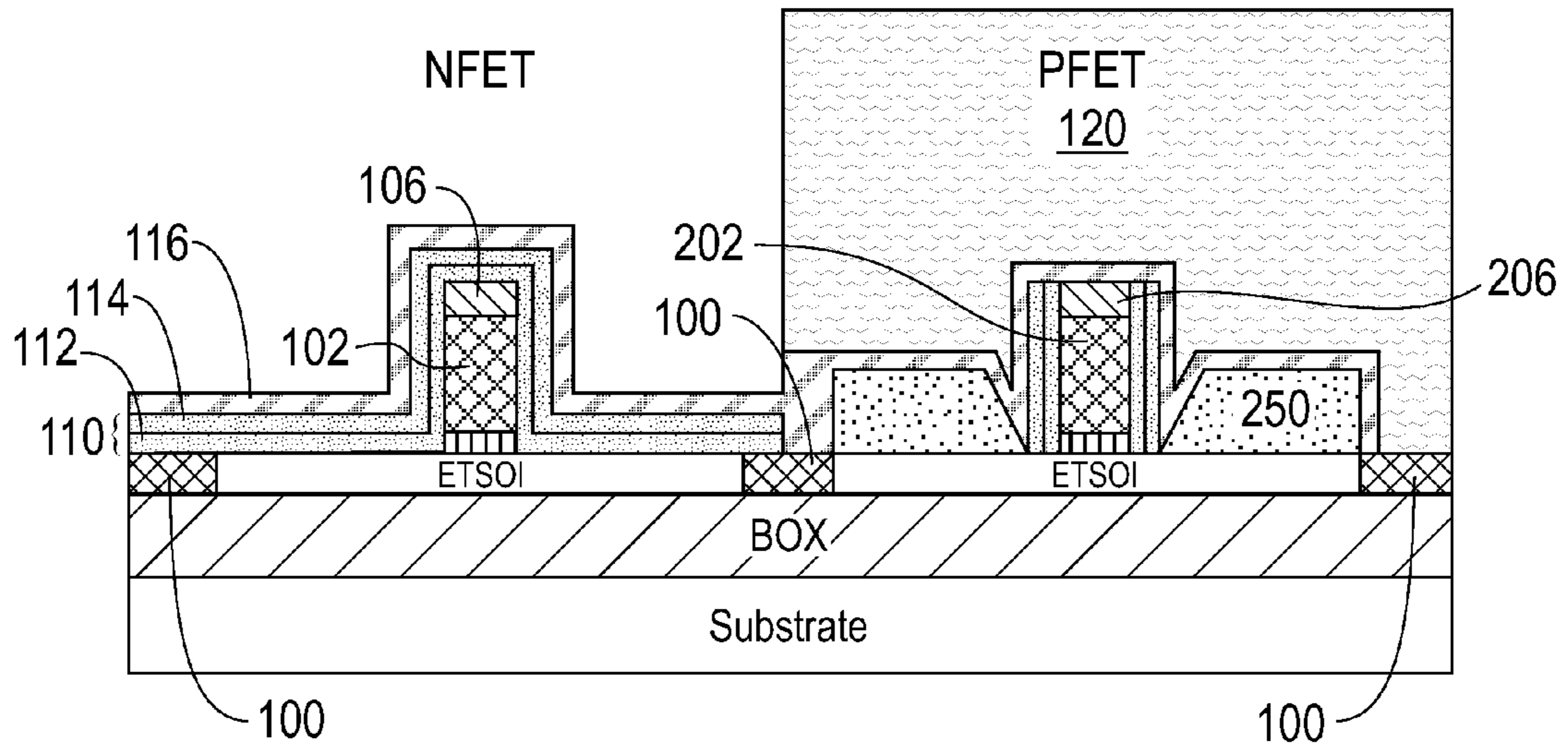
FIG. 3A
