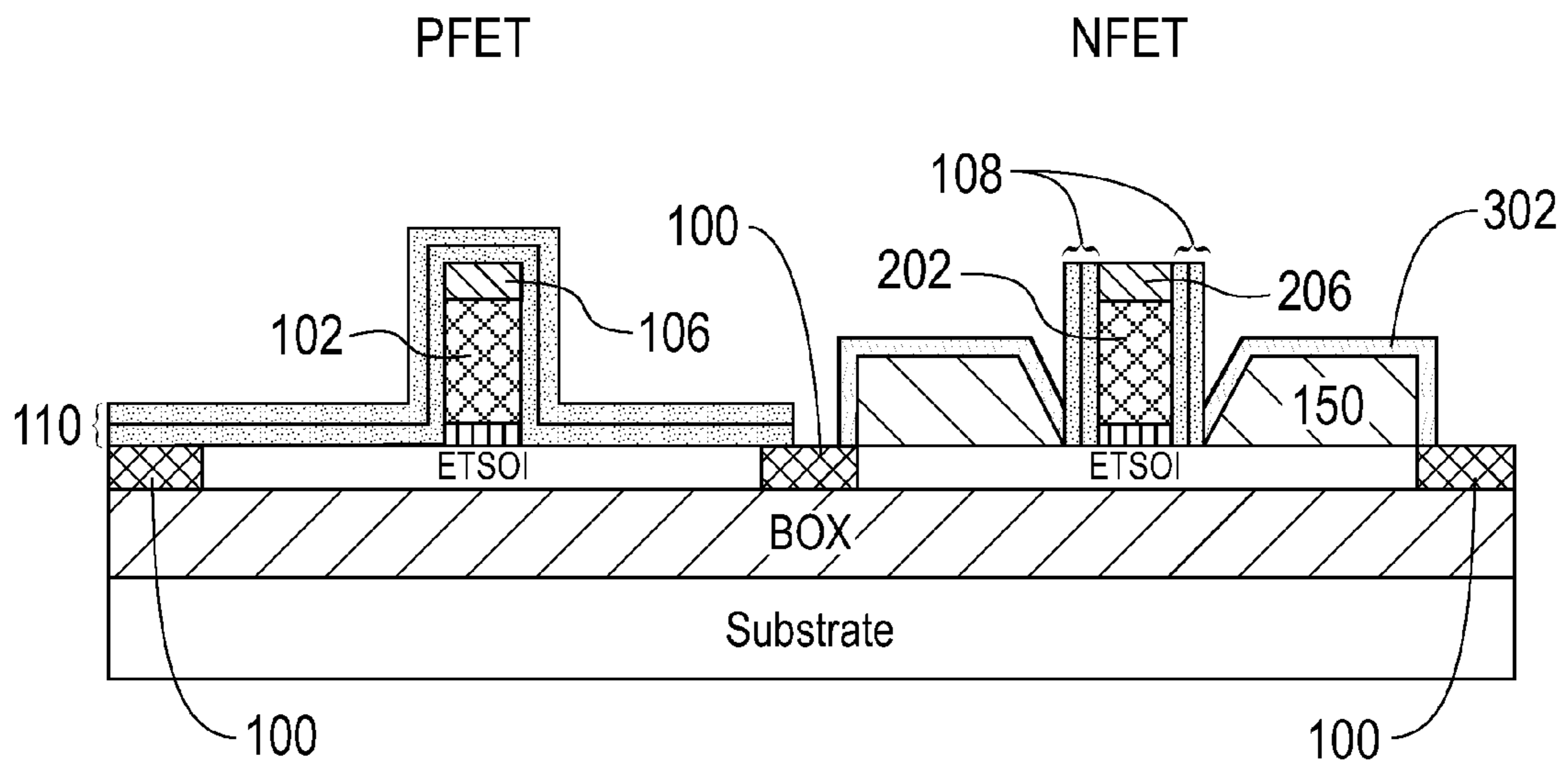
FIG. 4B
