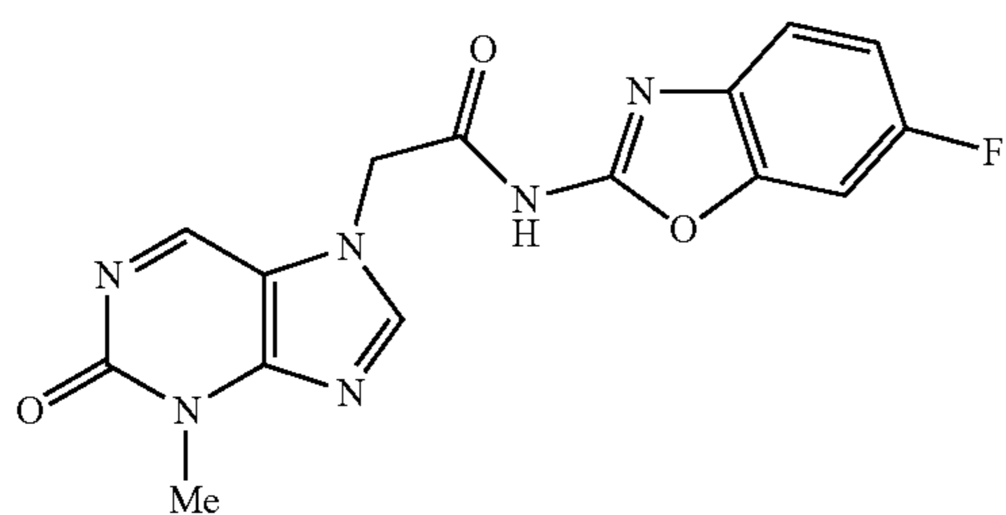
N-(6-fluorobenzo[d]oxazol-2-yl)-2-(3-methyl-2-oxo-2,3-dihydropurin-7-yl)acetamide
