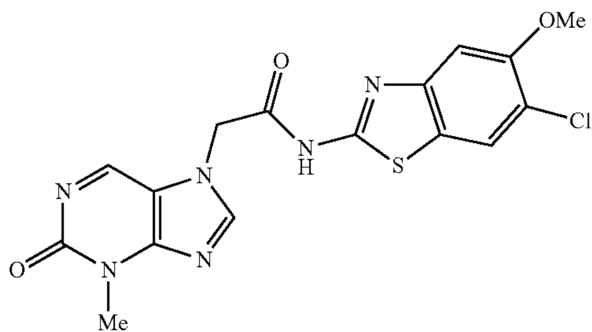
N-(6-chloro-5-methoxybenzo[d]thiazol-2-yl)-2-(3-methyl-2-oxo-2,3-dihydropurin-7-yl)acetamide
