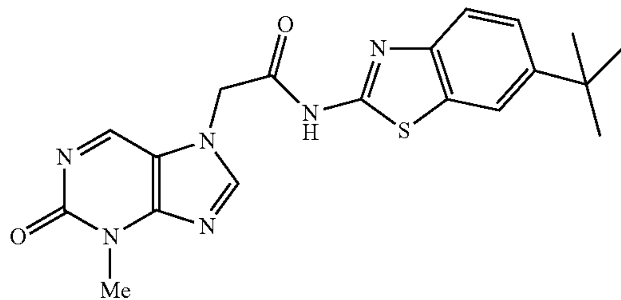
N-(6-tert-butylbenzo[d]thiazol-2-yl)-2-(3-methyl-2-oxo-2,3-dihydropurin-7-yl)acetamide
