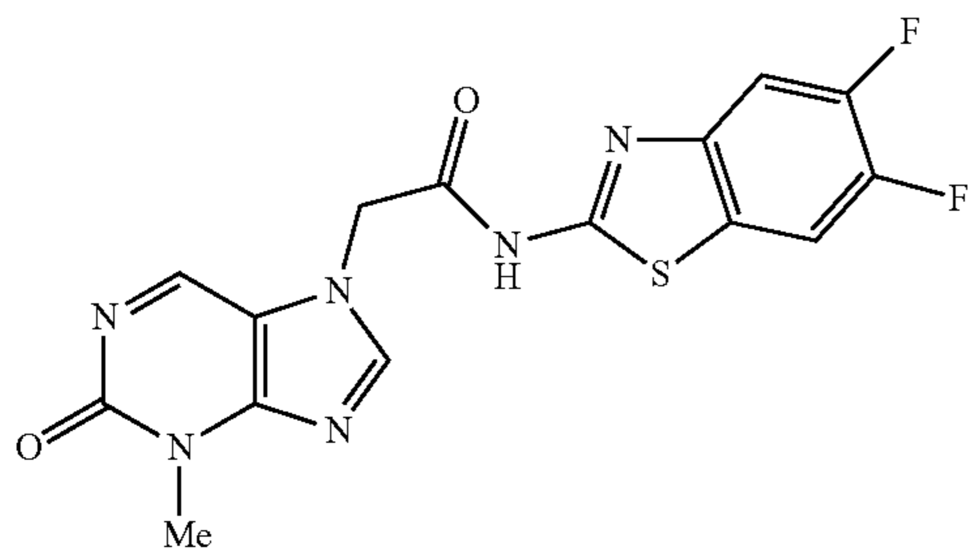
N-(5,6-difluorobenzo[d]thiazol-2-yl)-2-(3-methyl-2-oxo-2,3-dihydropurin-7-yl)acetamide
