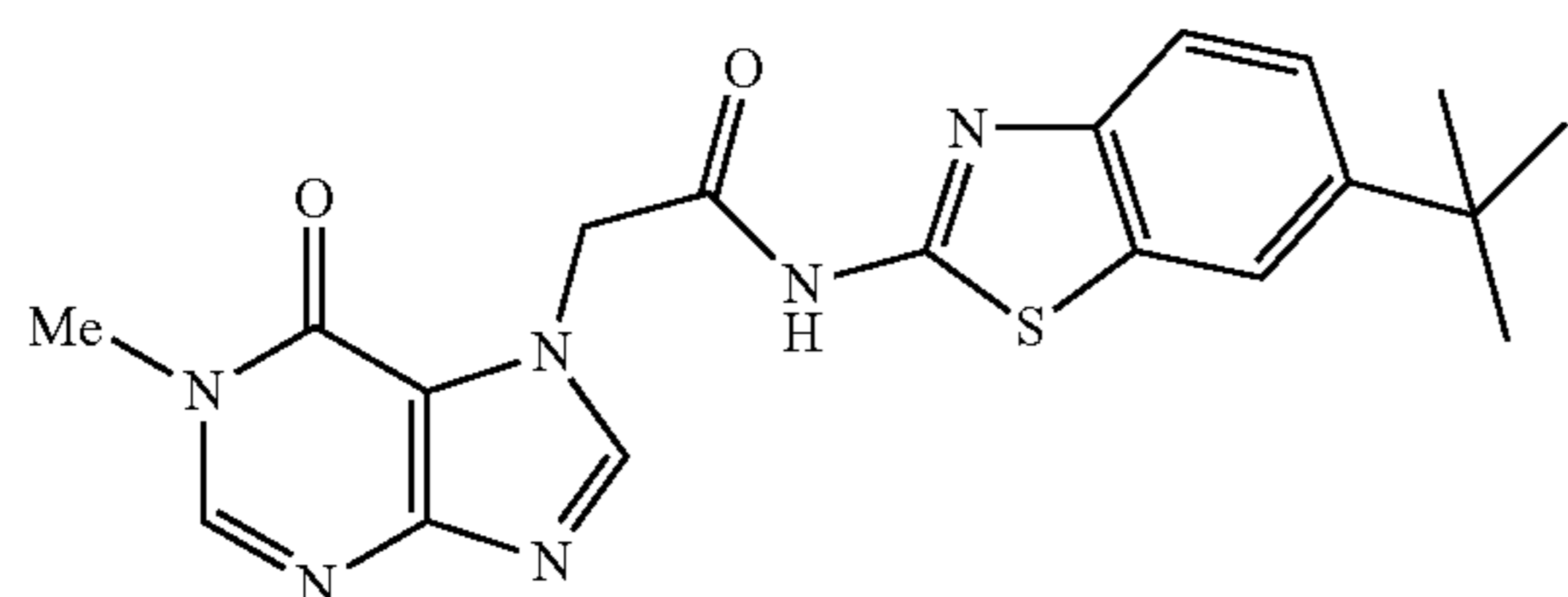
N-(6-tert-butylbenzo[d]thiazol-2-yl)-2-(1-methyl-6-oxo-1H-purin-7(6H)-yl)acetamide
