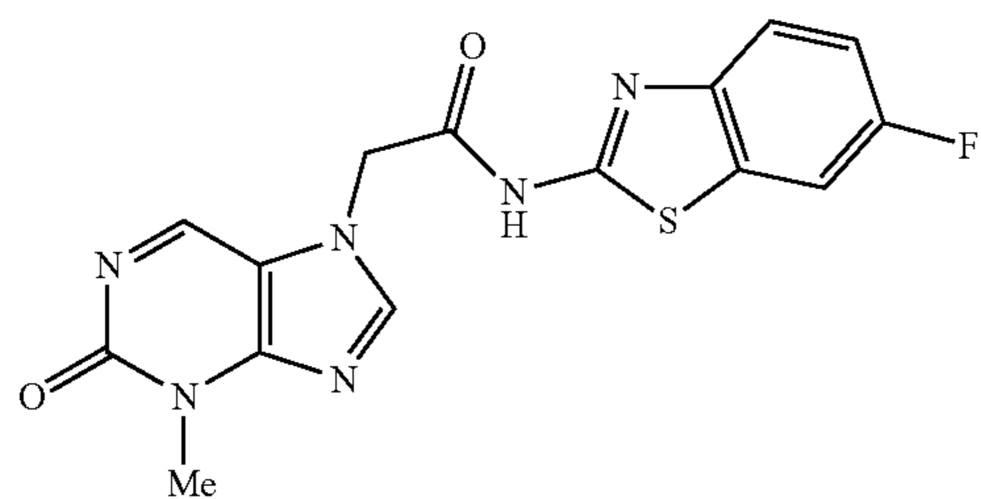
N-(6-fluorobenzo[d]thiazol-2-yl)-2-(3-methyl-2-oxo-2,3-dihydropurin-7-yl)acetamide
