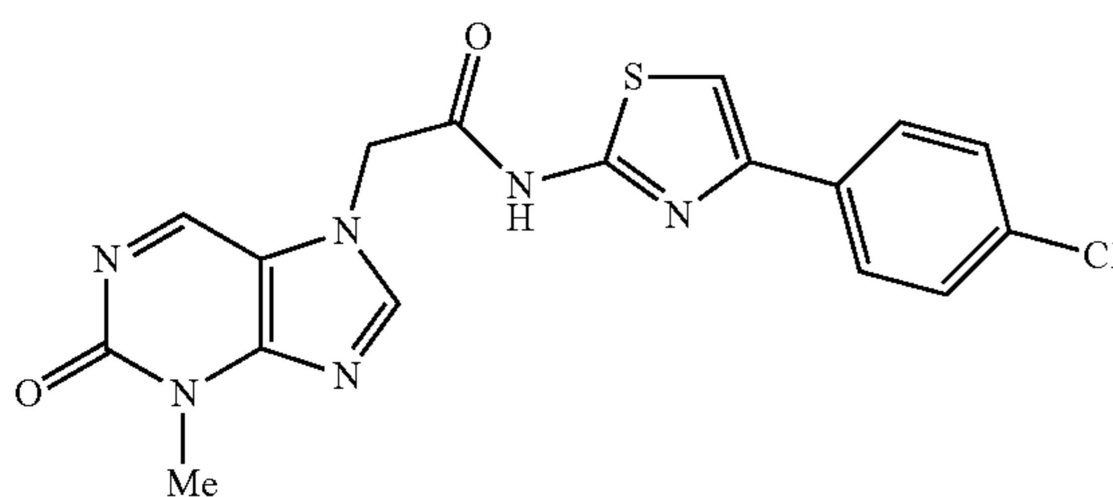
N-(4-(4-chlorophenyl)thiazol-2-yl)-2-(3-methyl-2-oxo-2,3-dihydropurin-7-yl)acetamide
