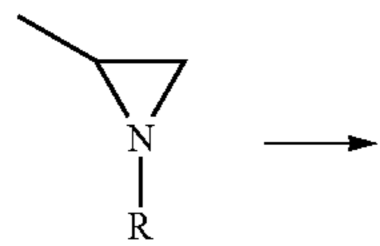
Tri-Aziridine (PZ-28)
