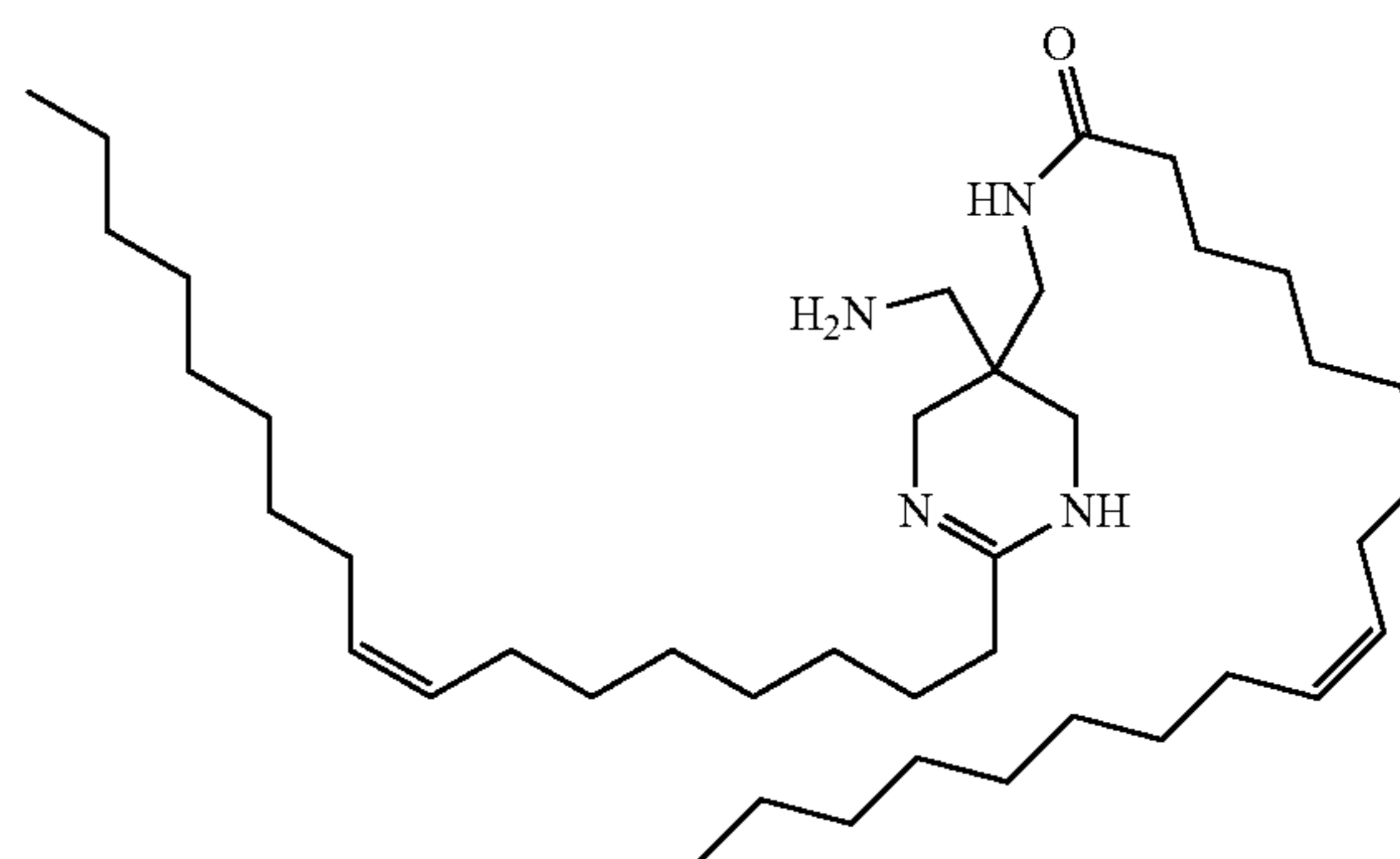
MS 643.6 [M + 1]
