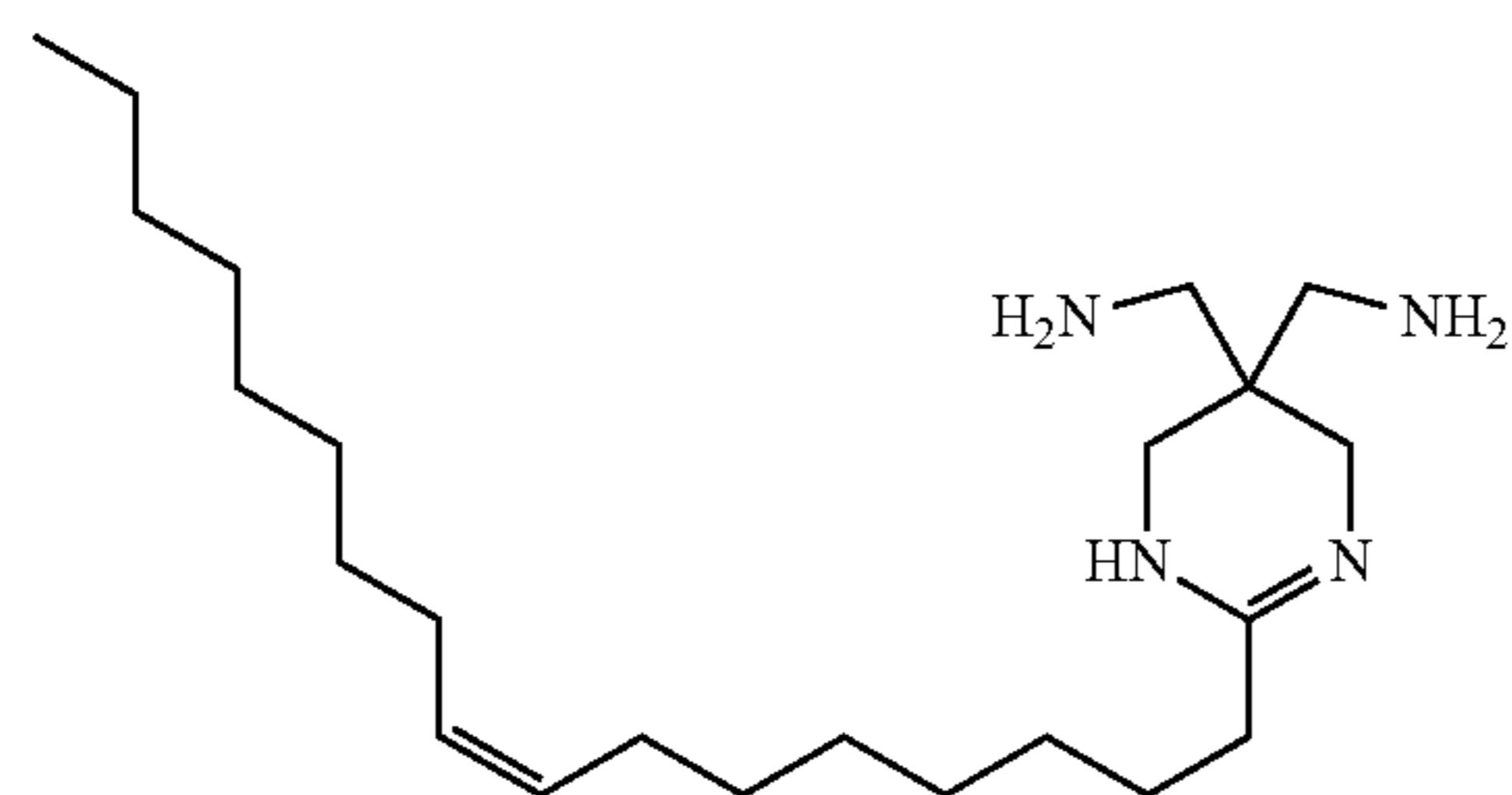
MS 379.4 [M + 1]
