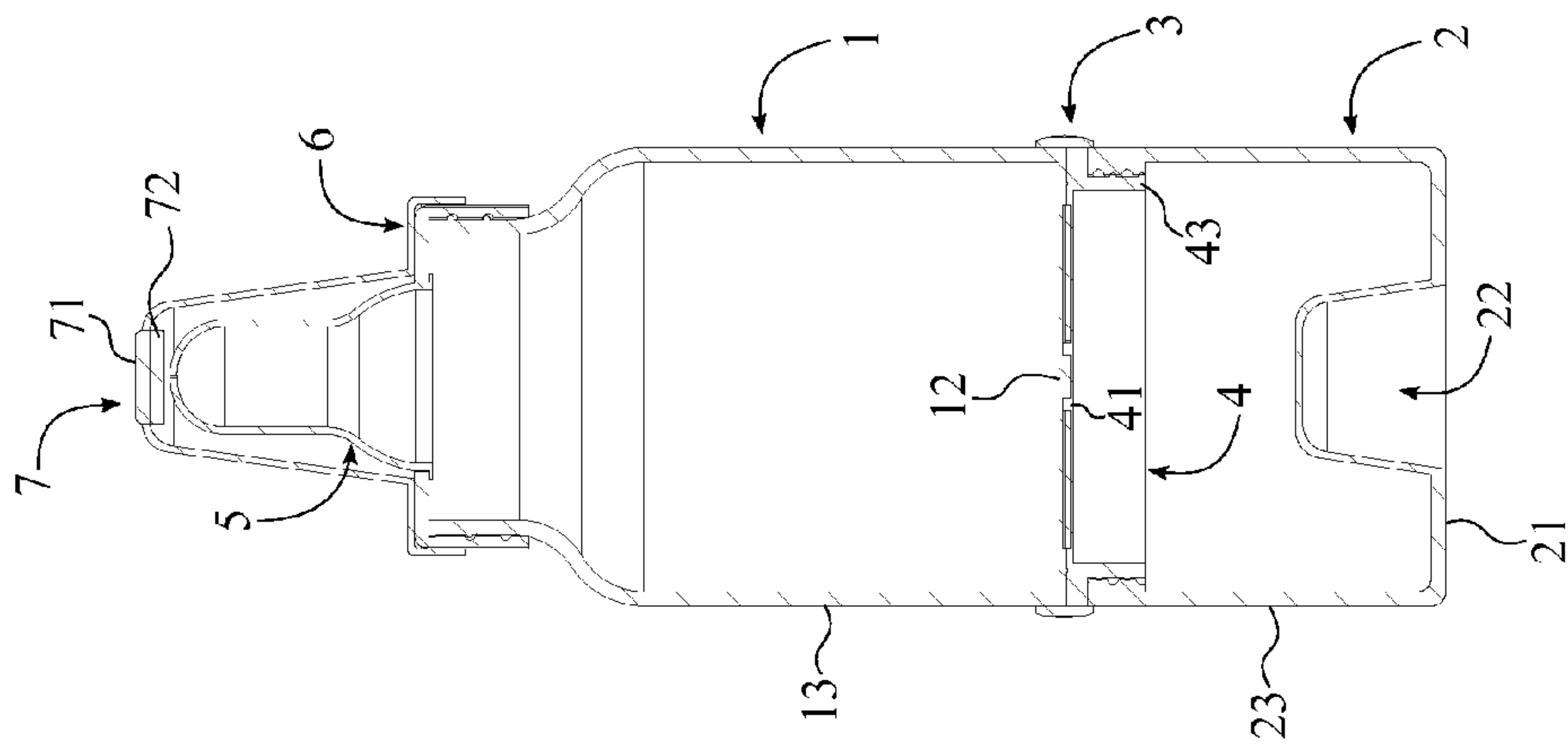
SECTION A-A
