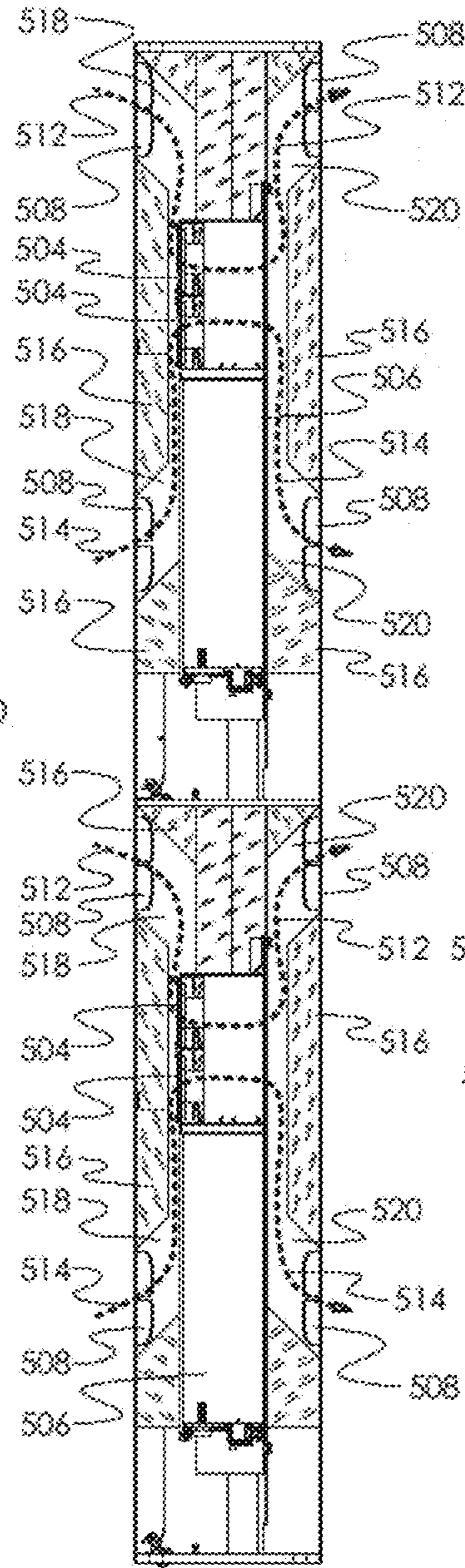
SECTION A-A FIG. 5B
