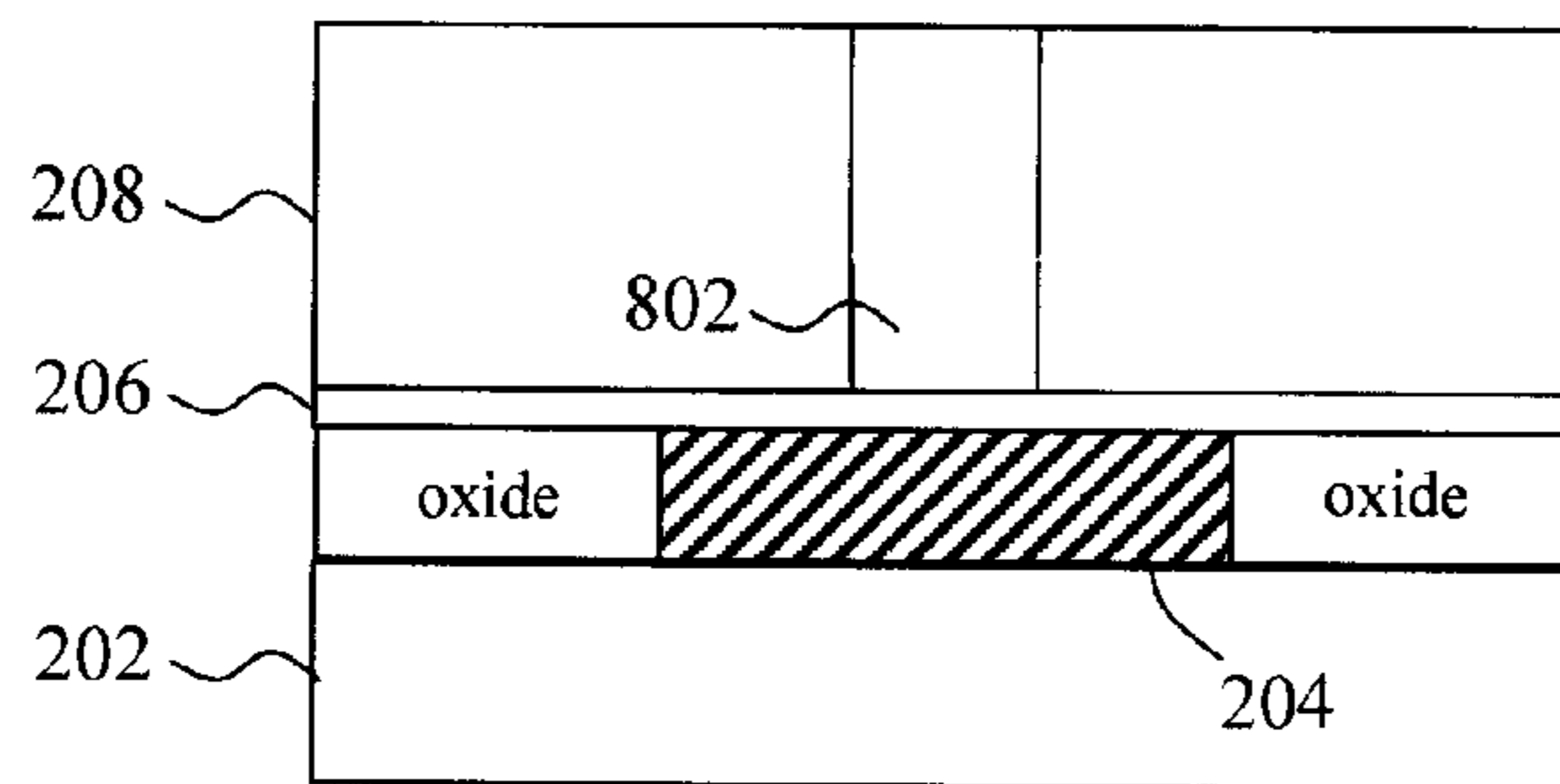
FIG. 8A
