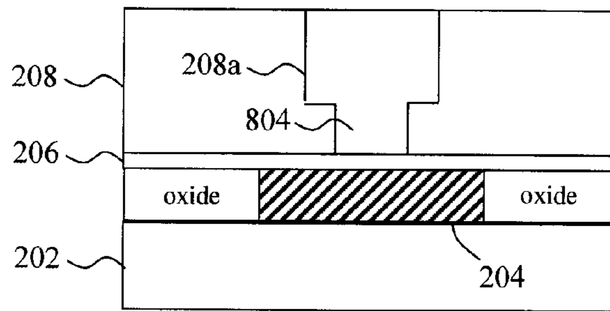
FIG. 8
