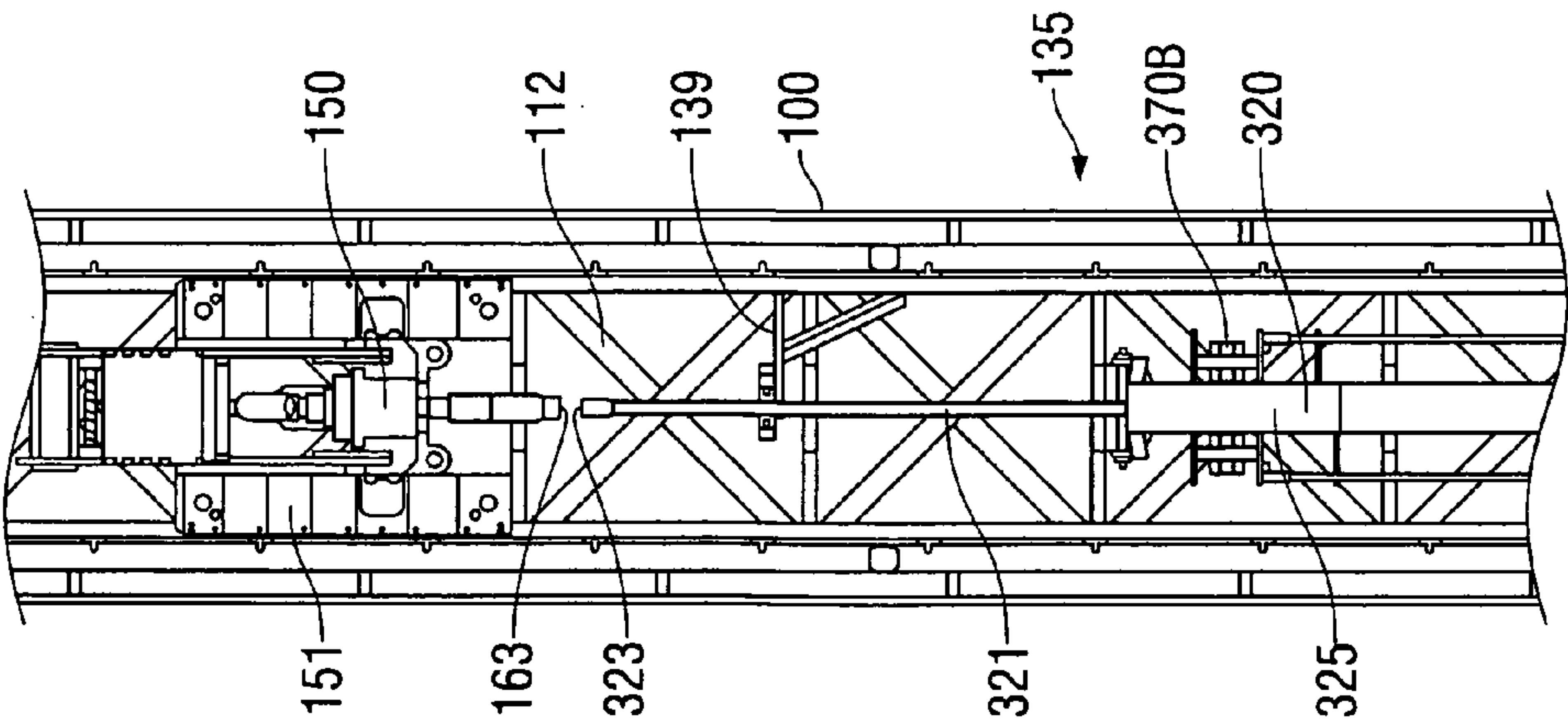
FIG. 7A-A
