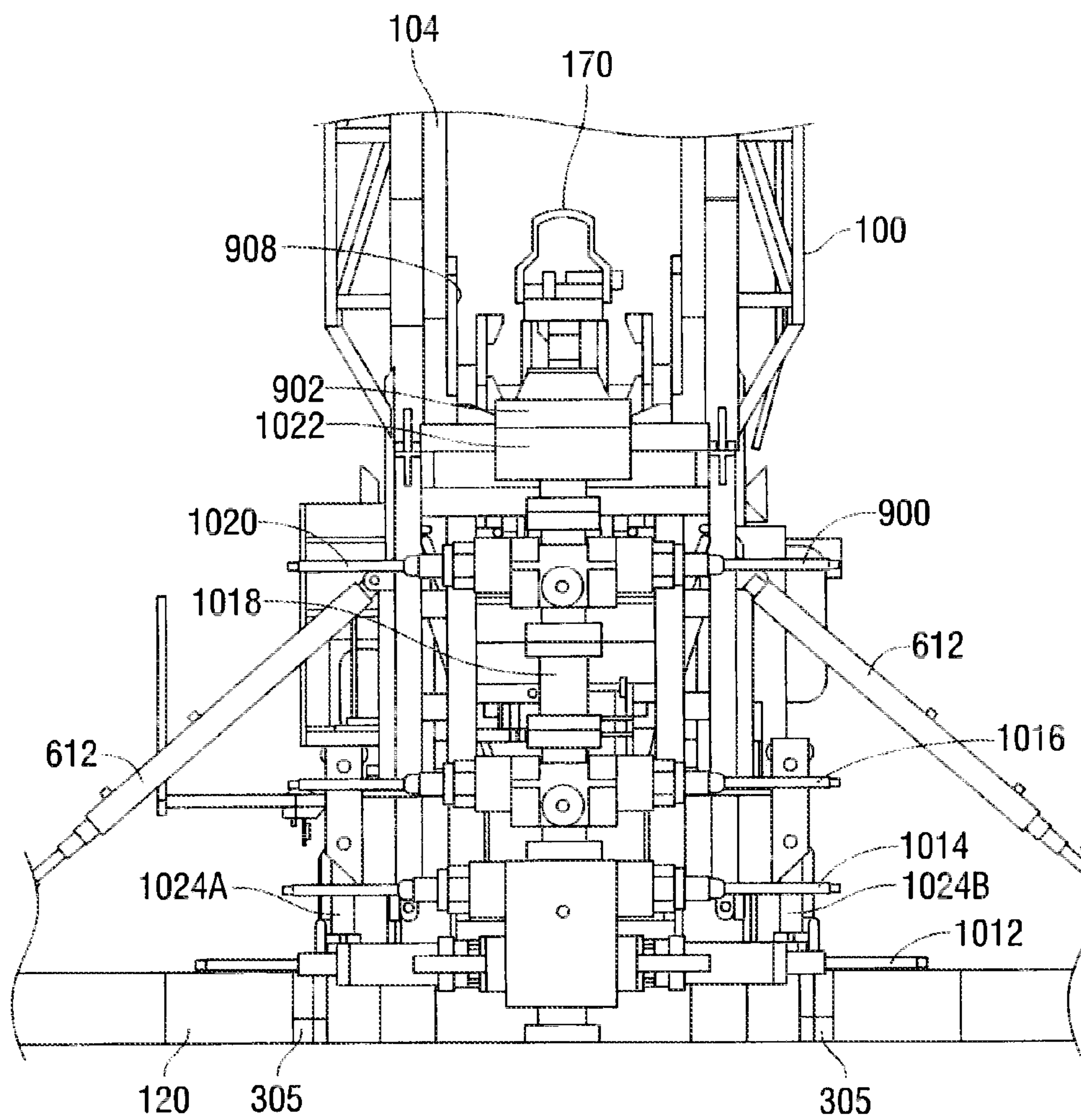
FIG. 9C-C
