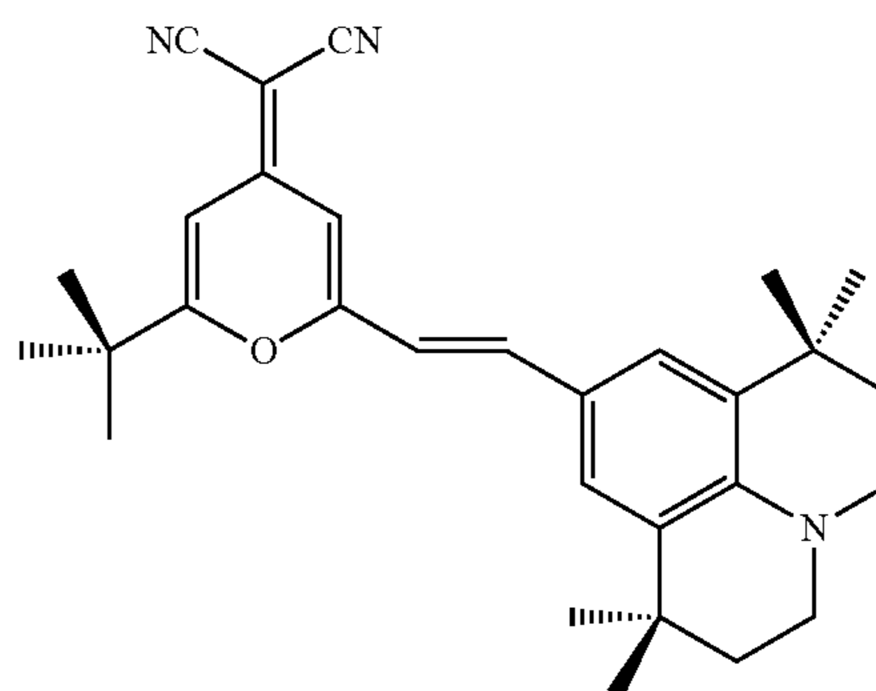
DCJTb
