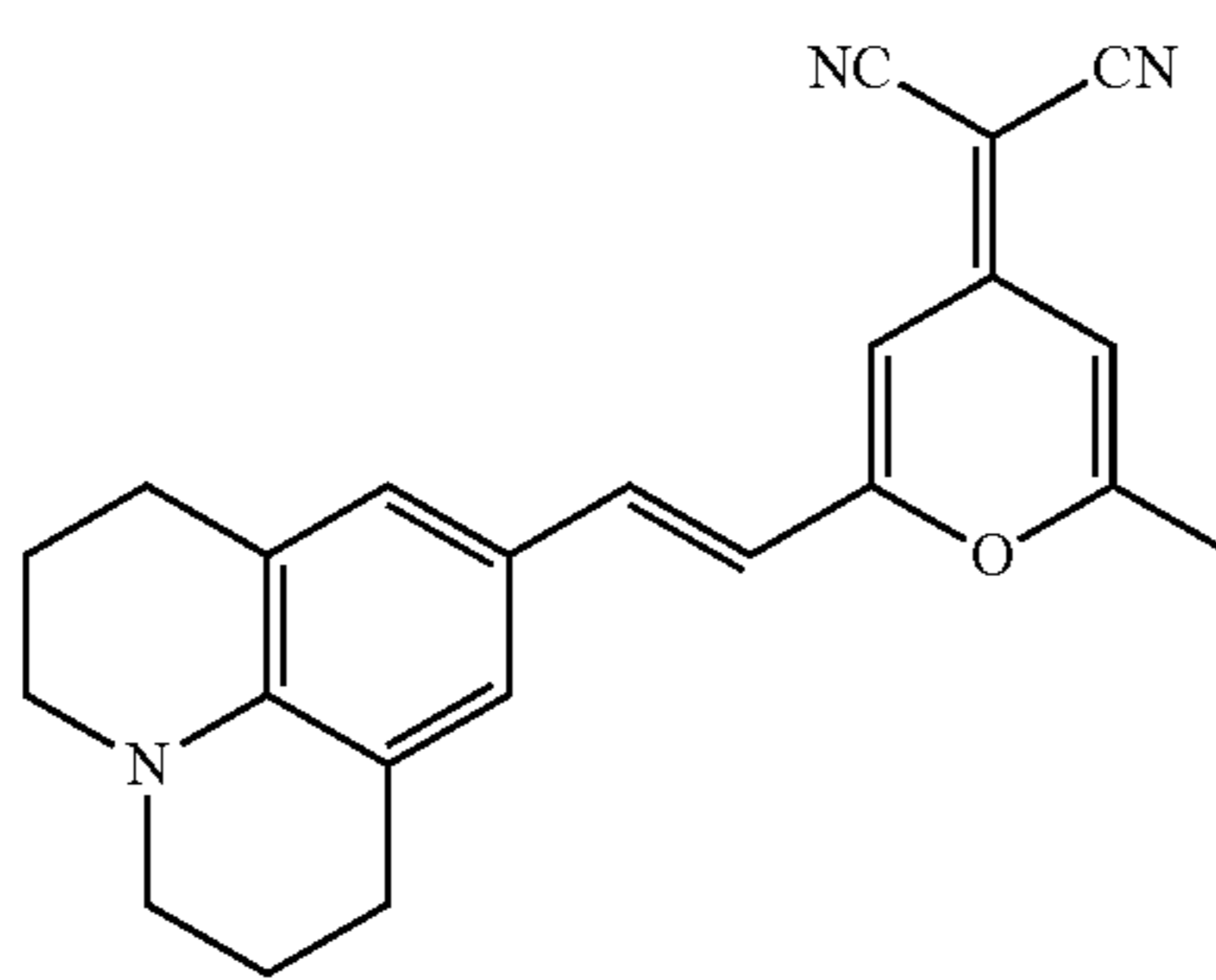
DCM
