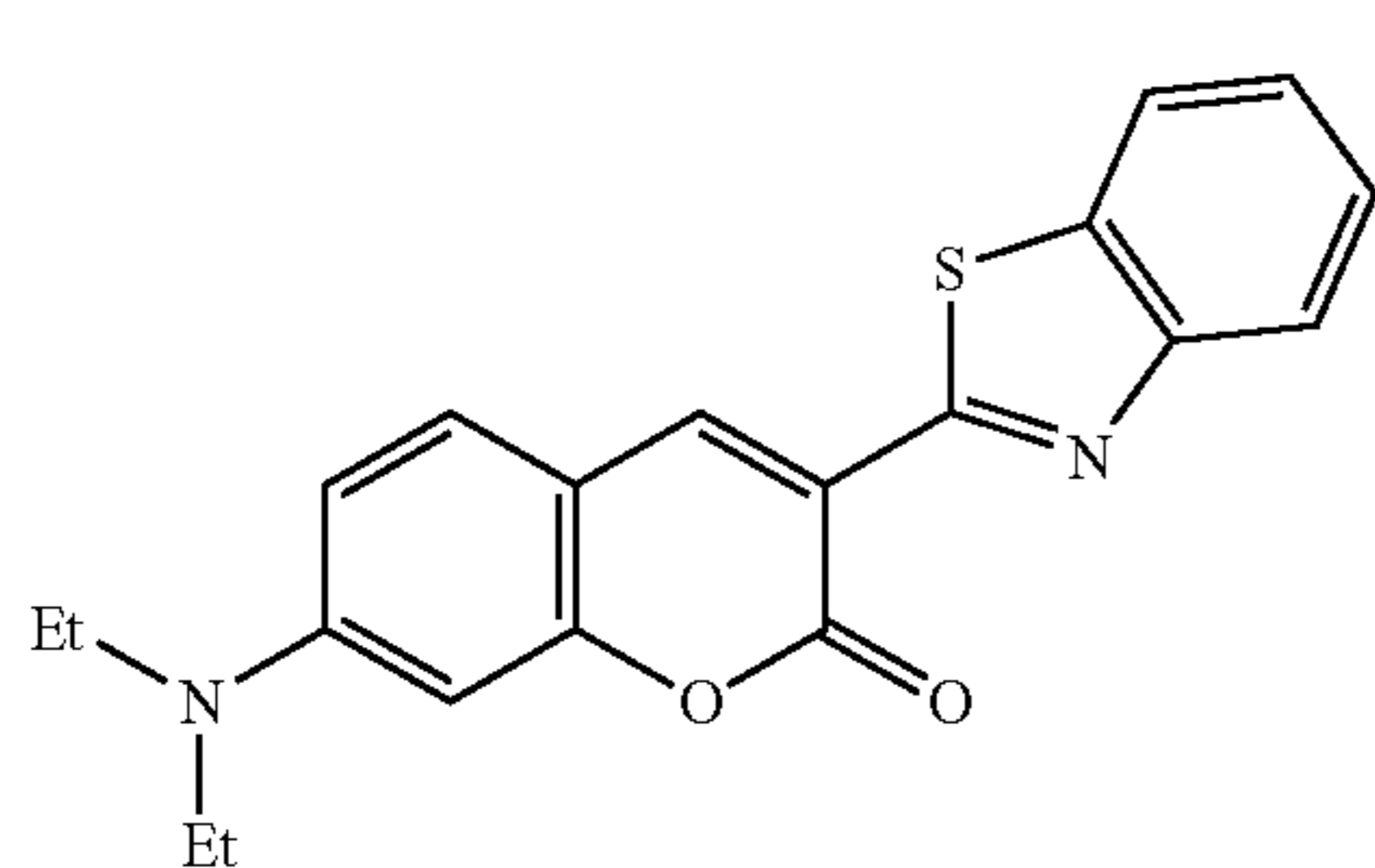
Coumarin 6
