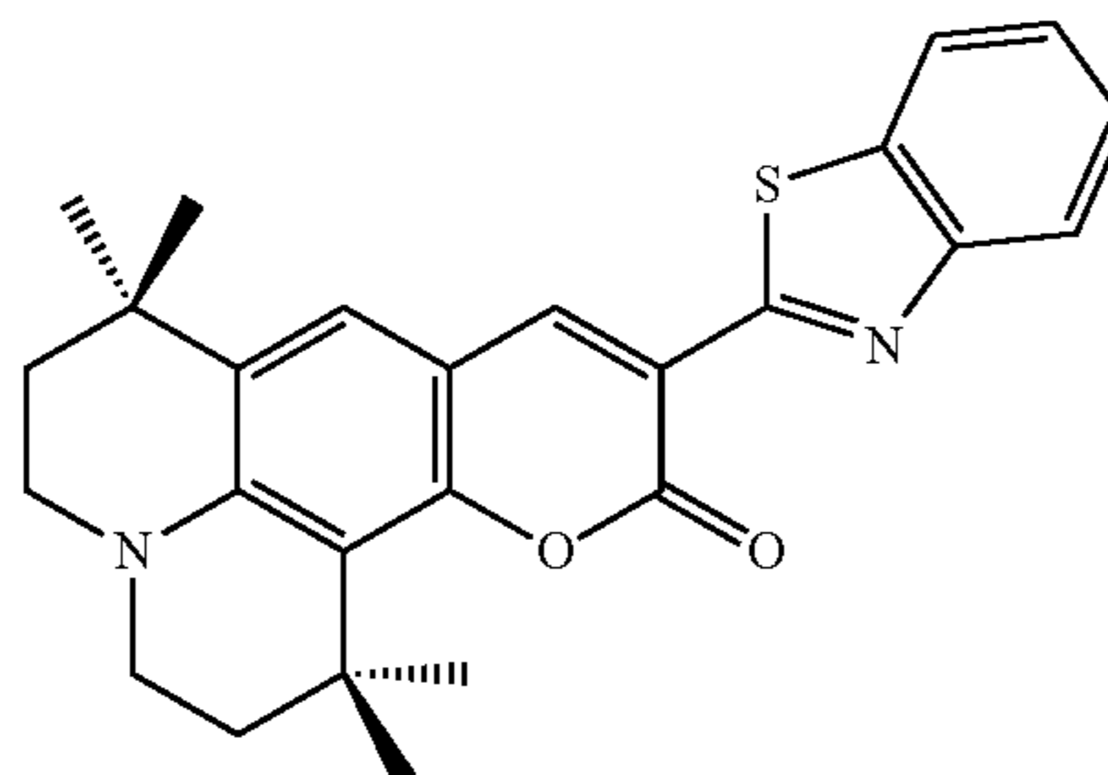
C545T
