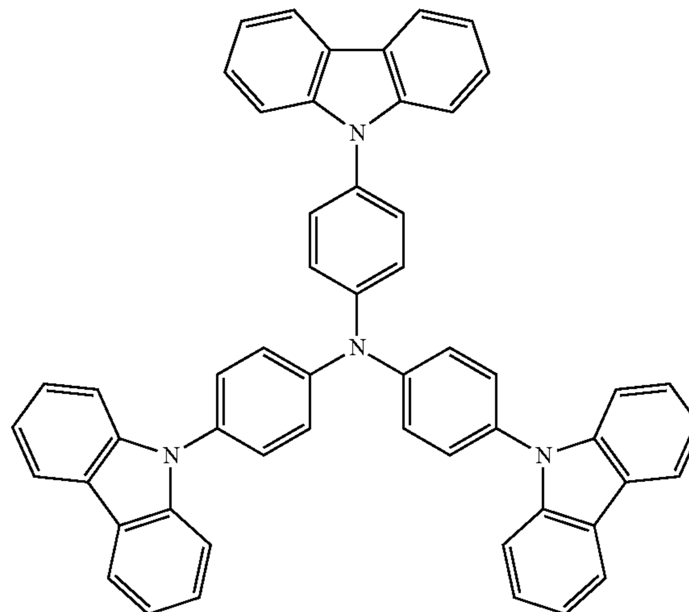
TCTA
