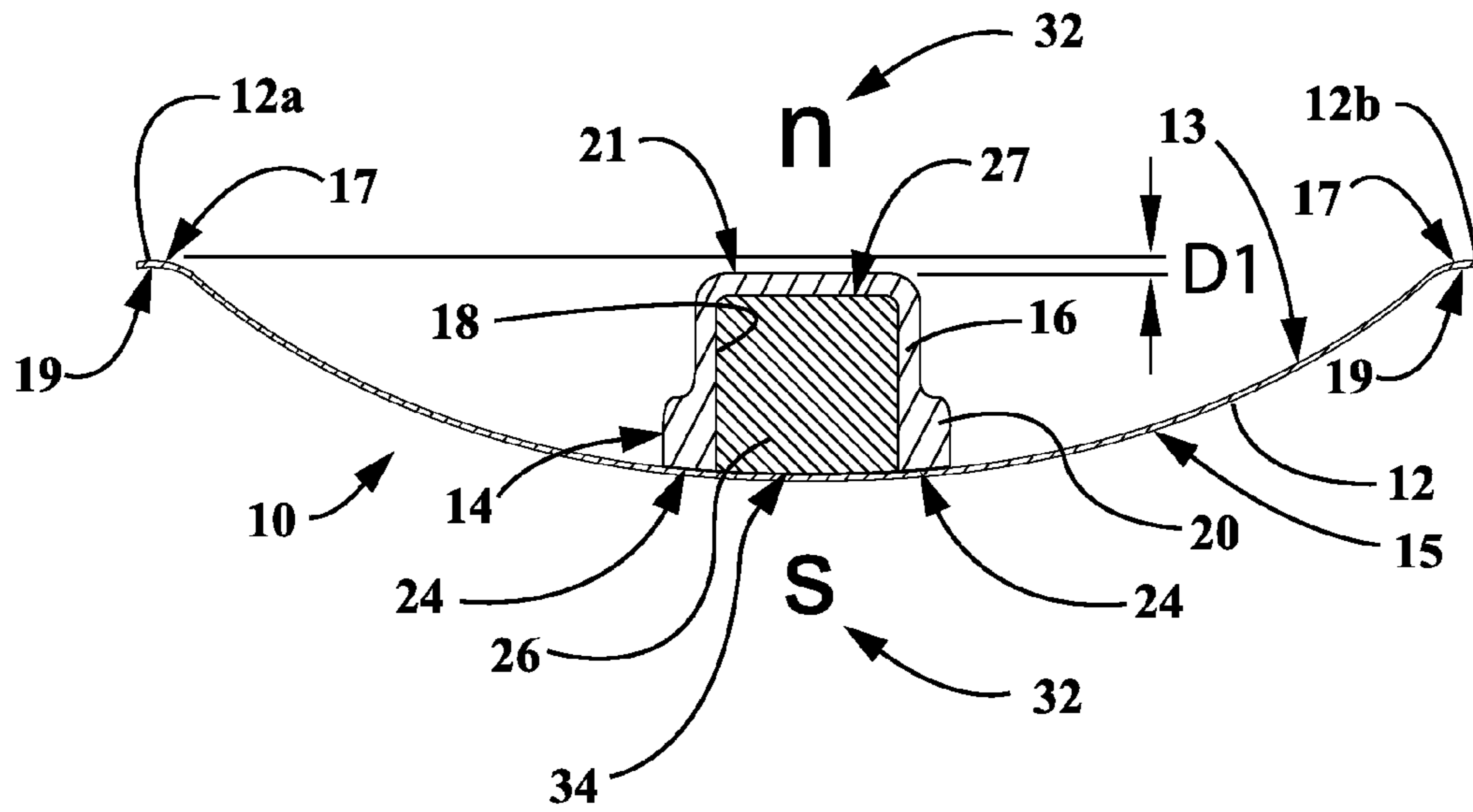
Section A-A
