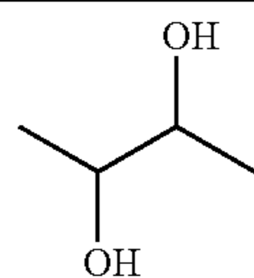
2,3-Butanediol
