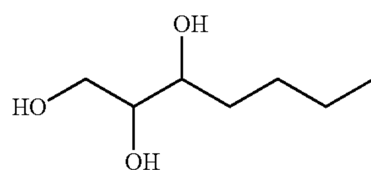
1,2,3-Heptanetriol
