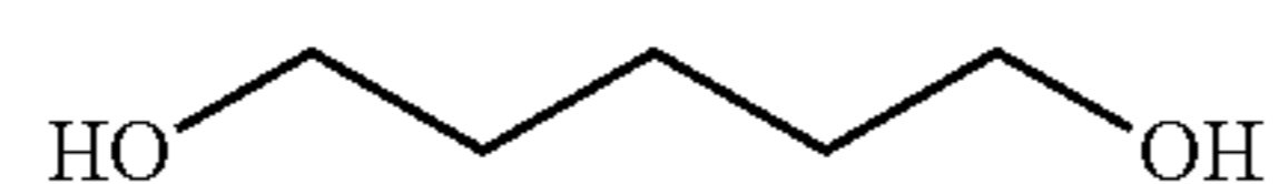
1,5-Pentanediol
