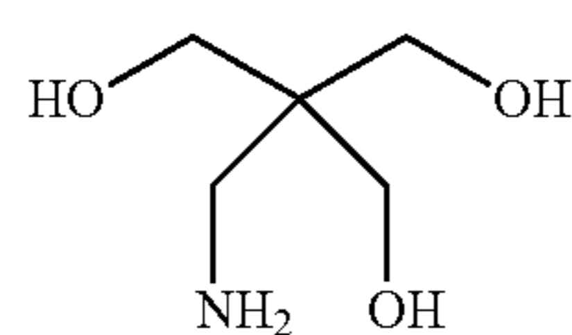
2-Amino-2-(hydroxymethyl)-1,3-propanediol
