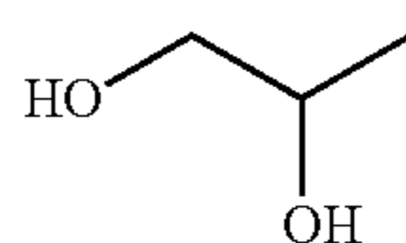
1,2-Propanediol
