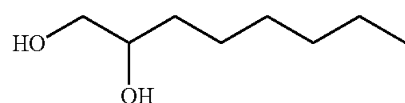
1,2-Octanediol
