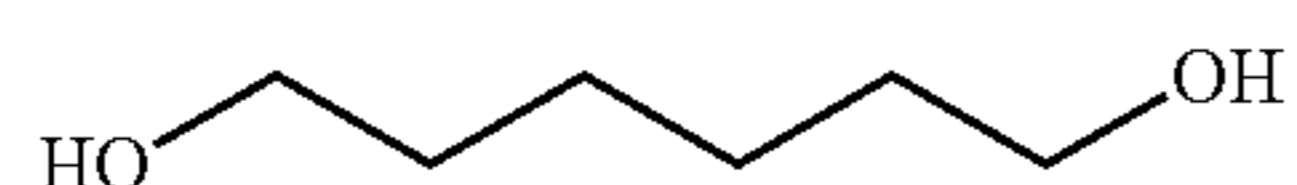
1,6-Hexanediol
