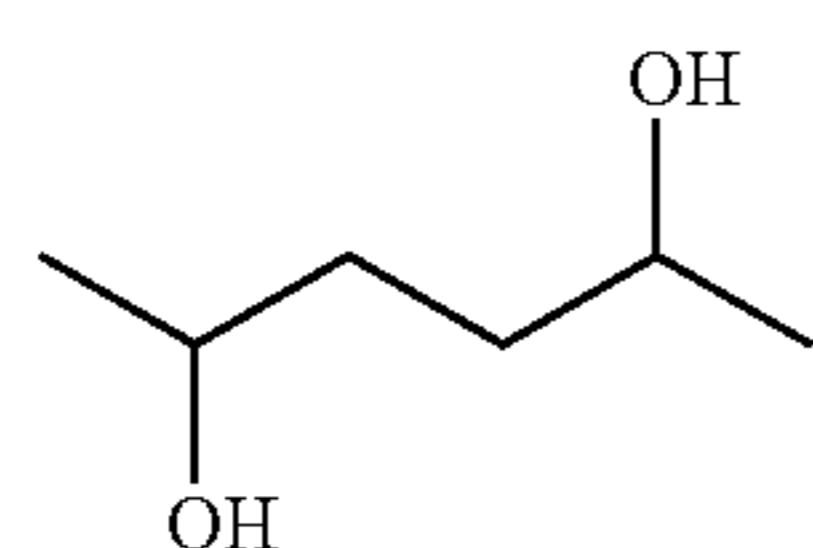
2,5-Hexanediol
