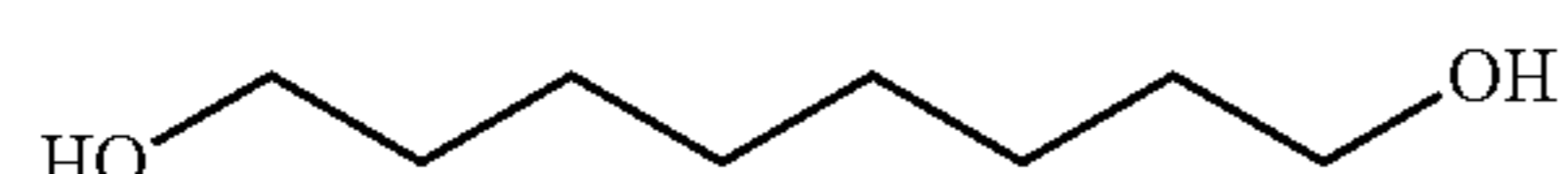
1,8-Octanediol
