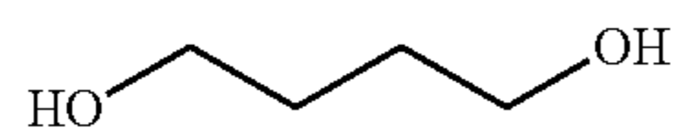
1,4-Butanediol
