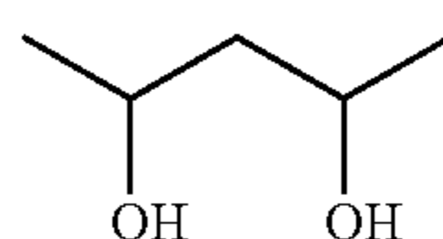
2,4-Pentanediol
