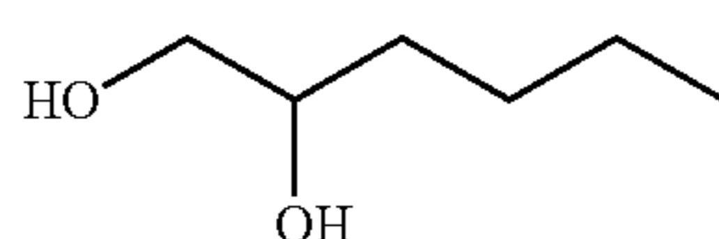
1,2-Hexanediol
