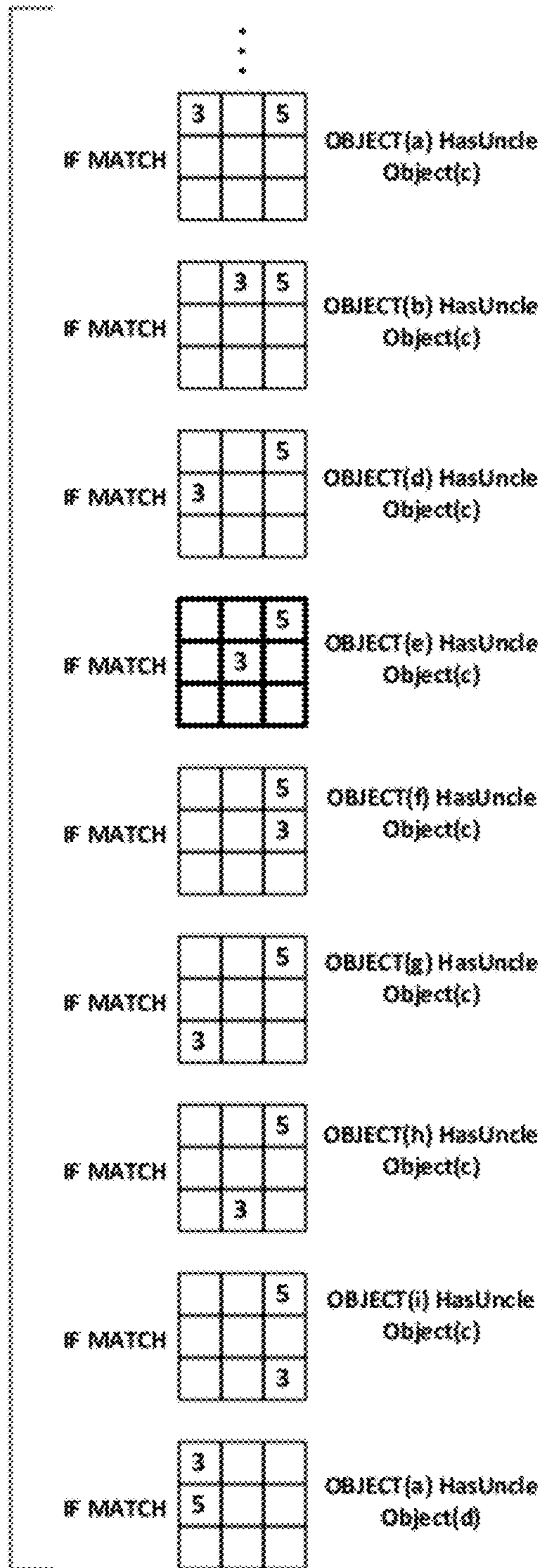
FIG. 26 – PREDICATE TEMPLATES
