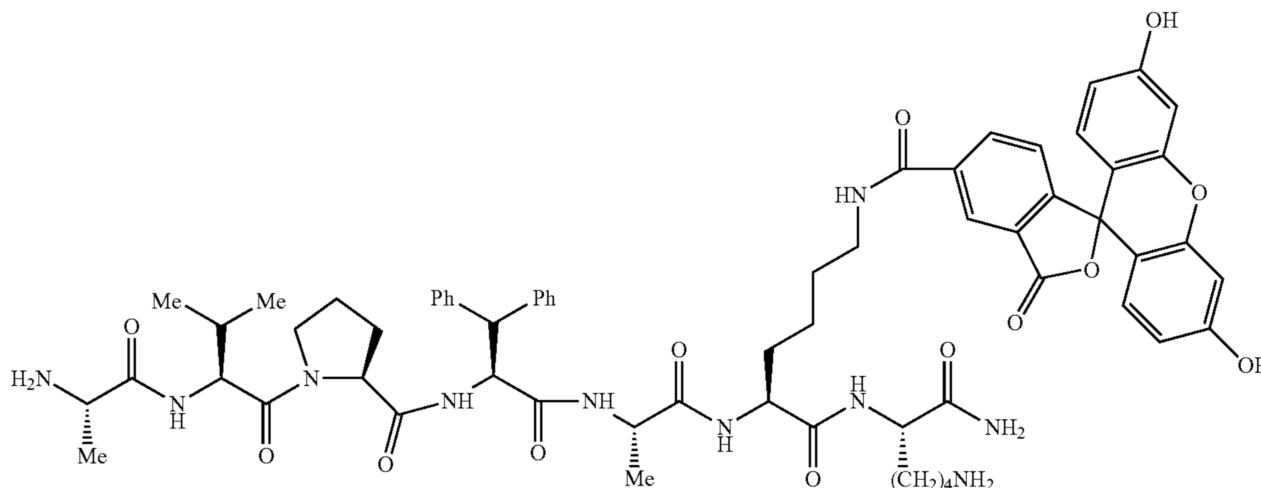
AVP-diPhe-FAM probe
