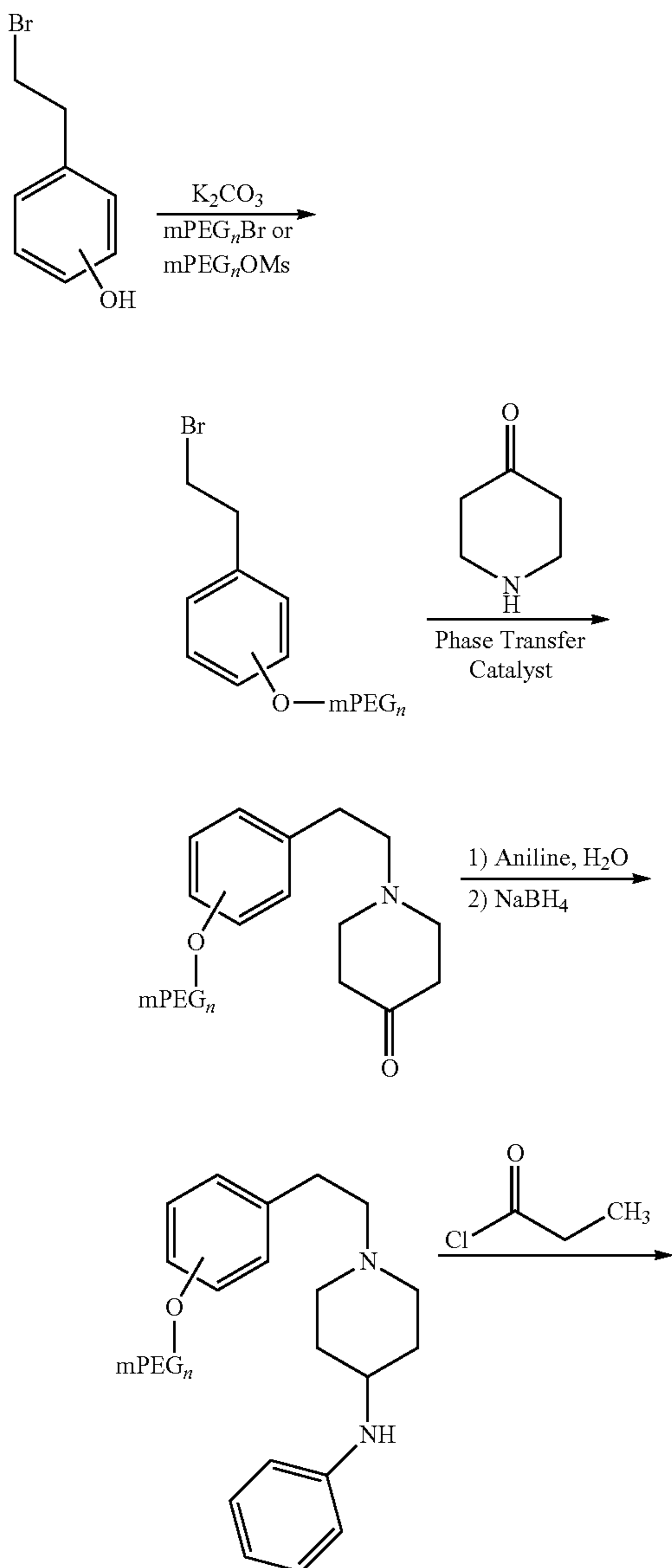
Scheme 11-A
