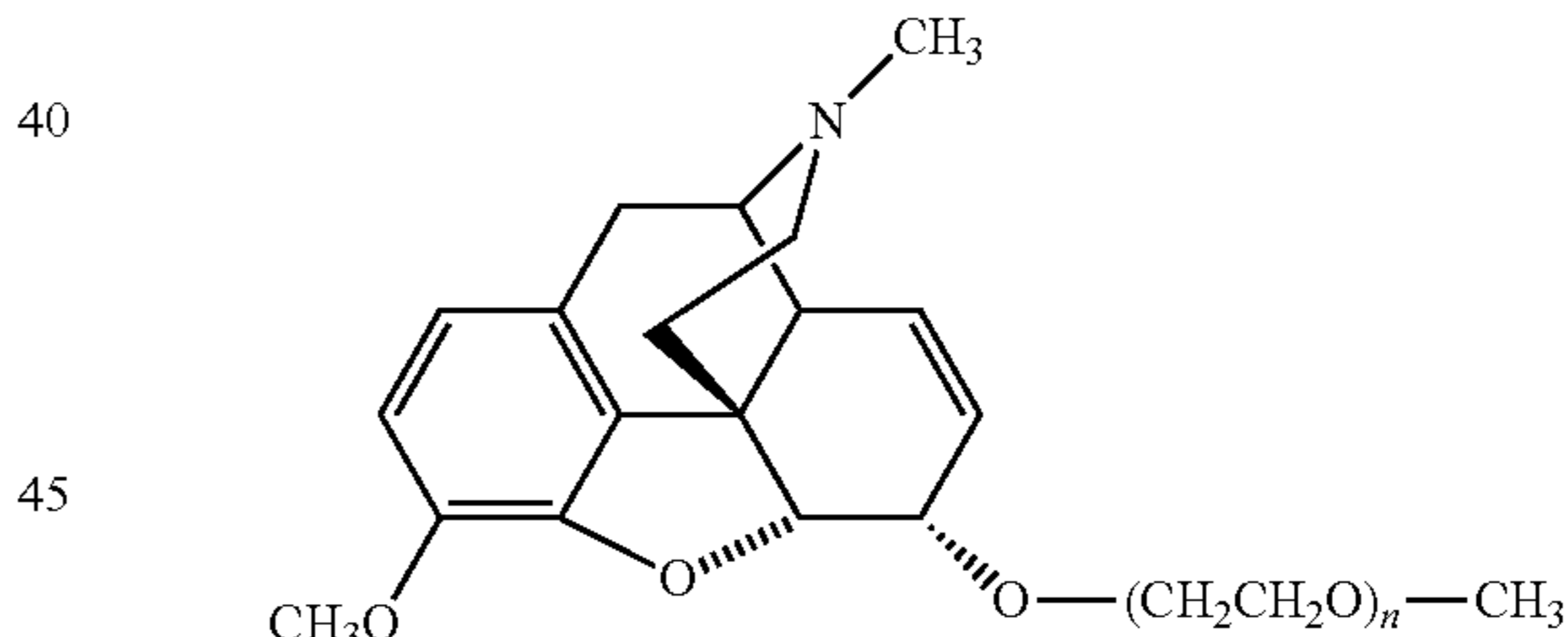
Formula I-Ce
