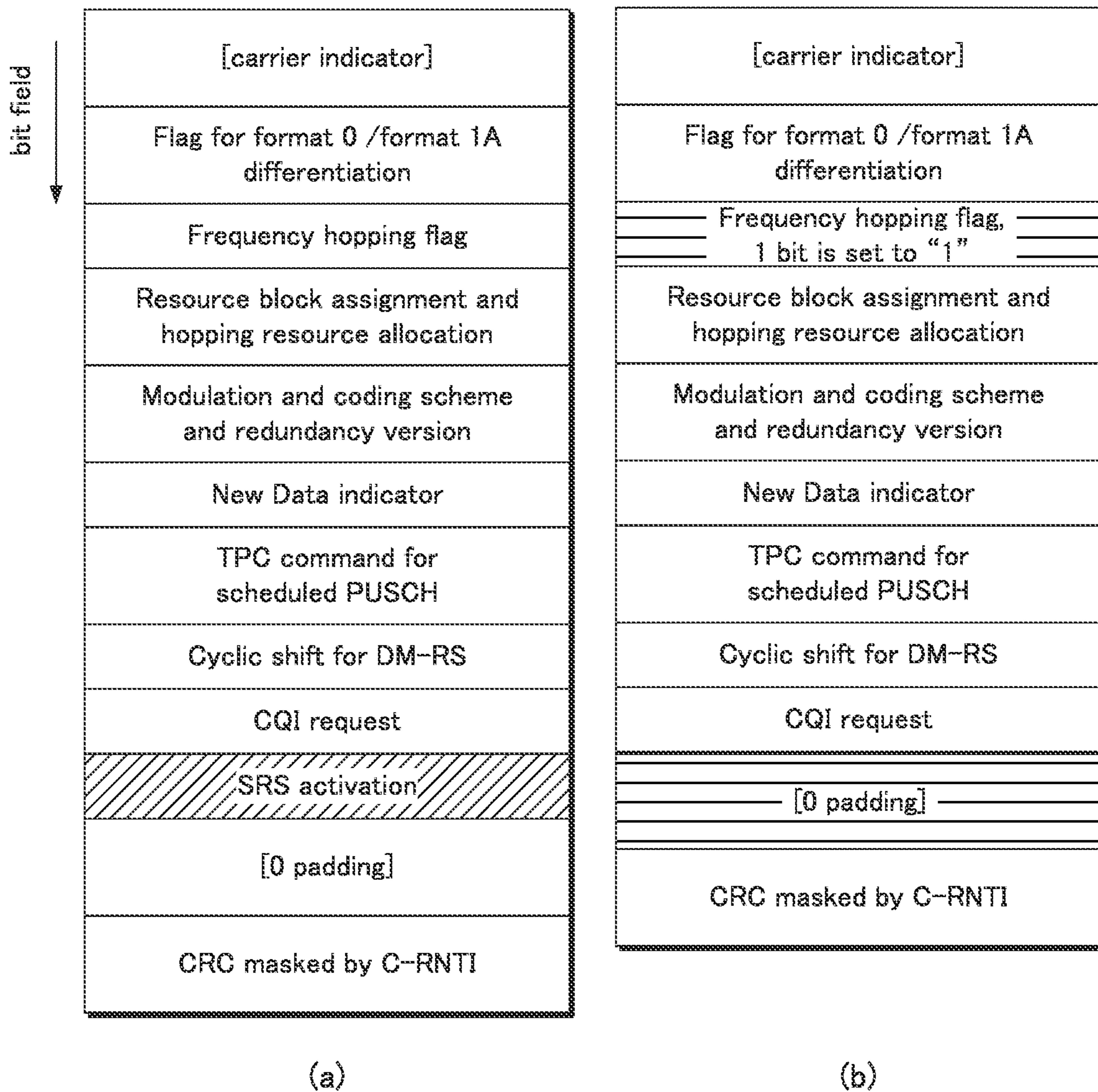
DCI format 0
