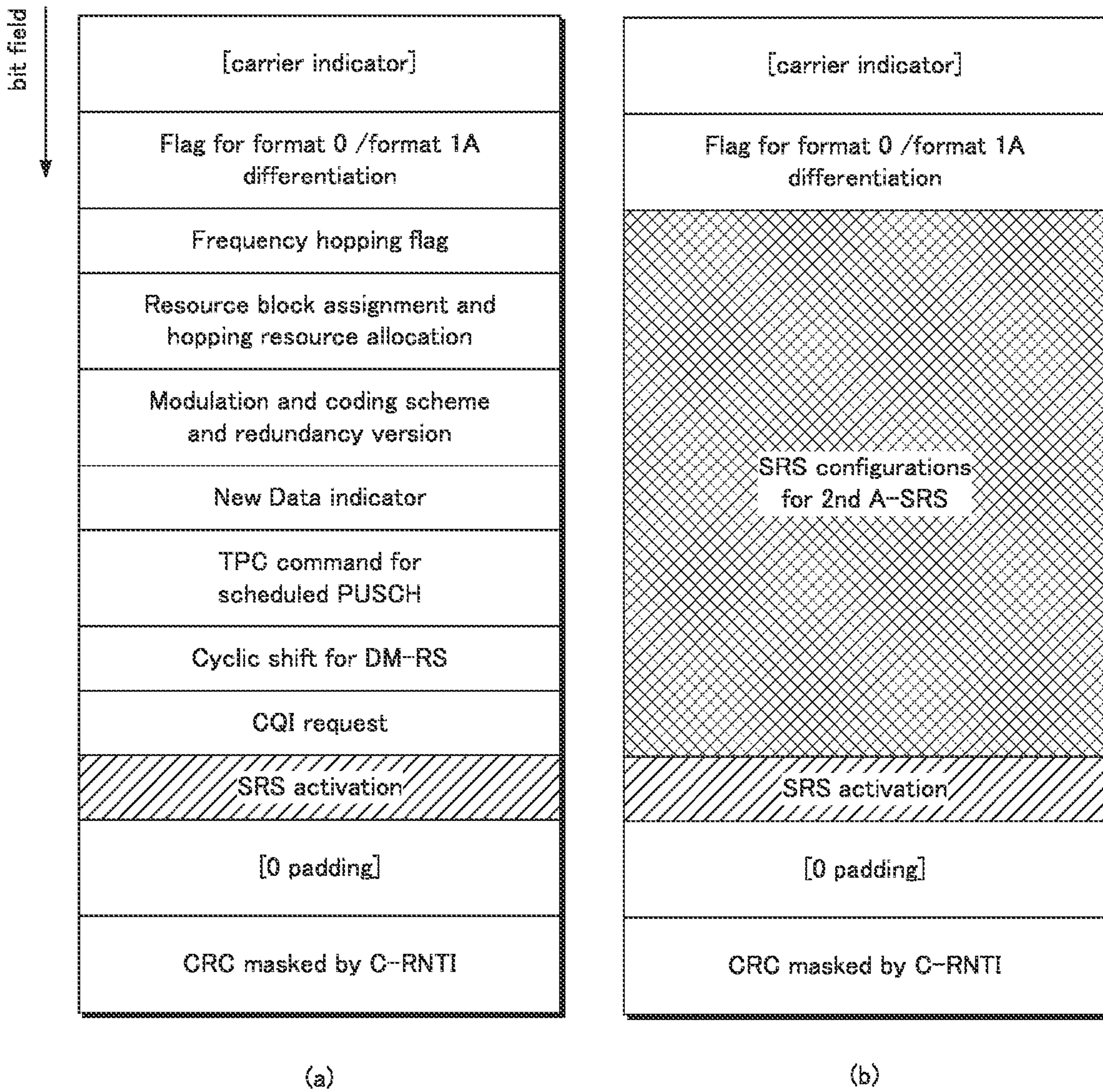
DCI format 0
