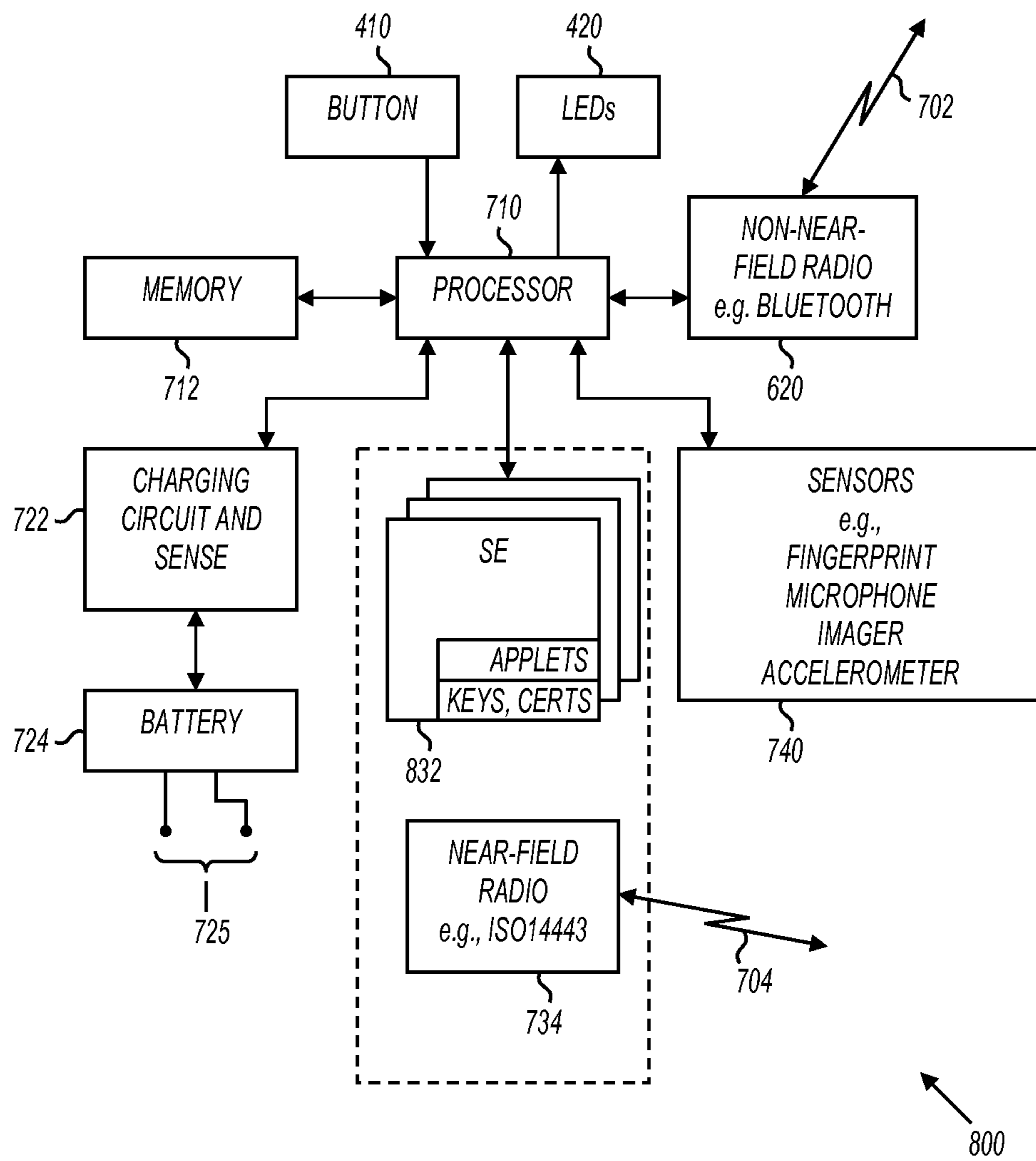
FIG. 8
