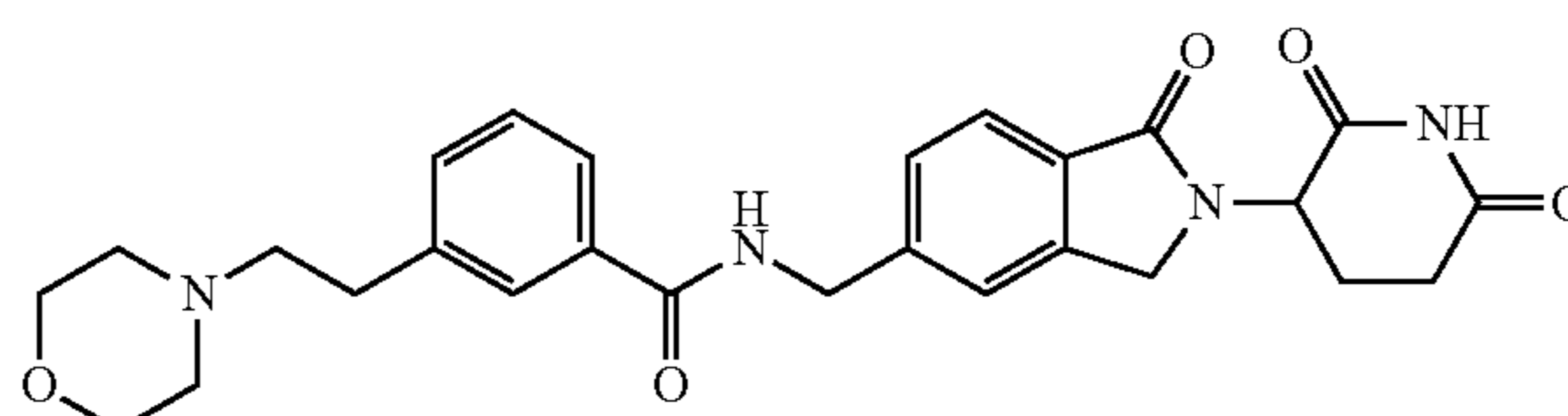
N-((2-(2,6-dioxopiperidin-3-yl)-1-oxoisindolin-5-yl)methyl)-3-morpholinoethylbenzamide;
