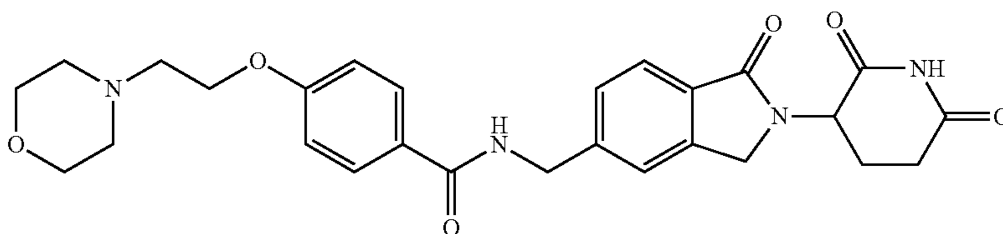
N-((2-(2,6-dioxopiperidin-3-yl)-1-oxoisindolin-5-yl)methyl)-4-(2-morpholinoethoxy)benzamide;
