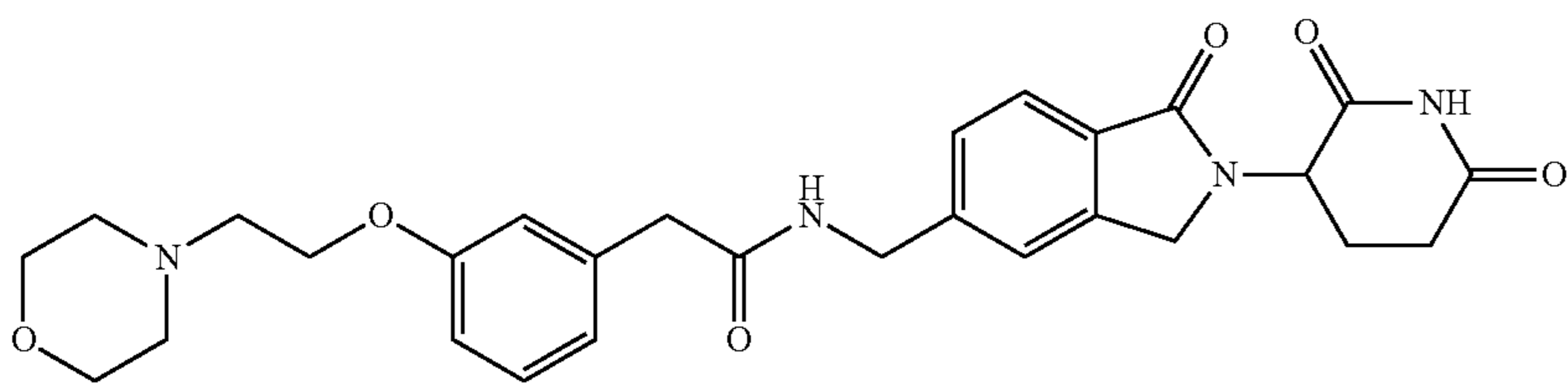
N-((2-(2,6-dioxopiperidin-3-yl)-1-oxoisindolin-5-yl)methyl)-2-(3-(2-morpholinoethoxy)phenyl)acetamide;
