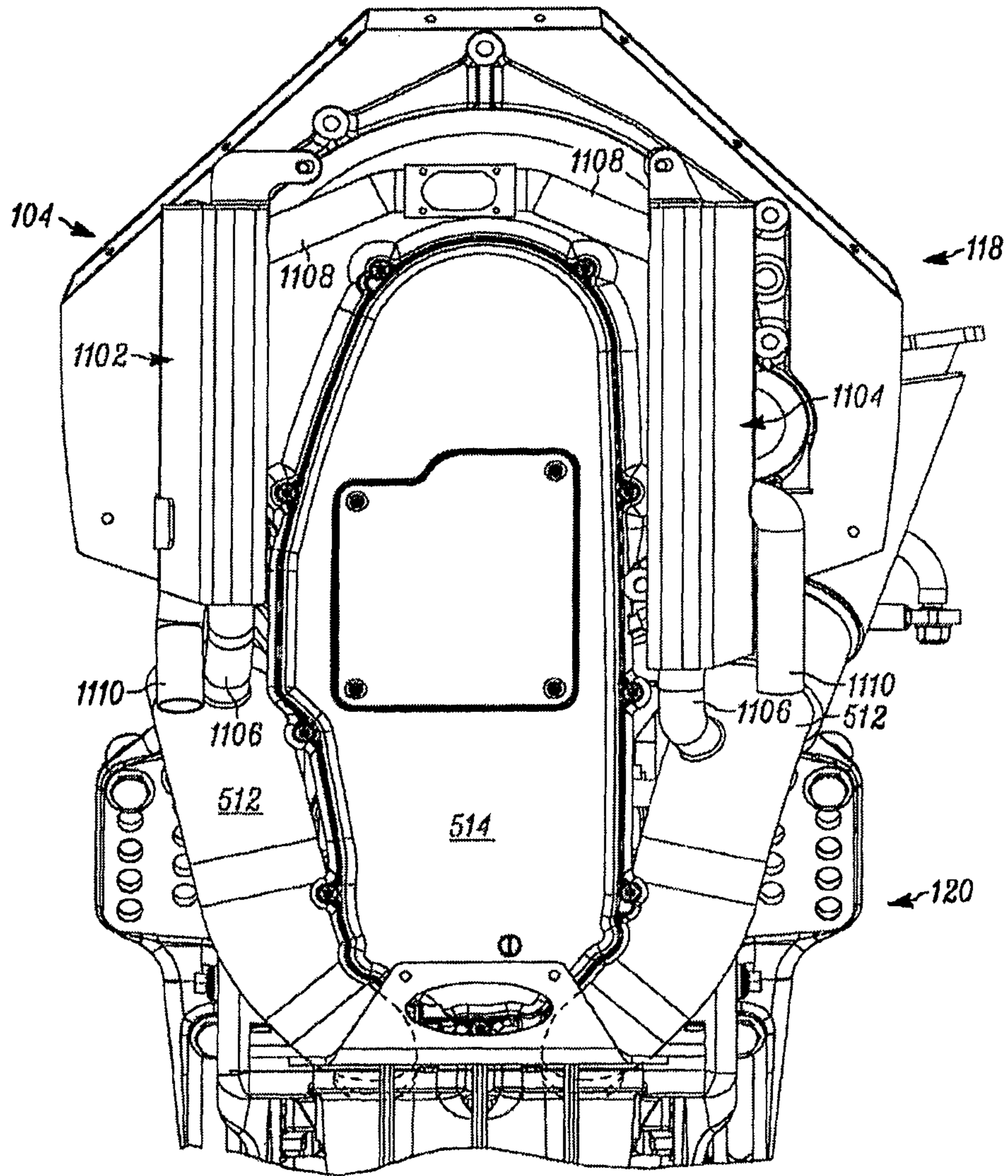
FIG. 11A
