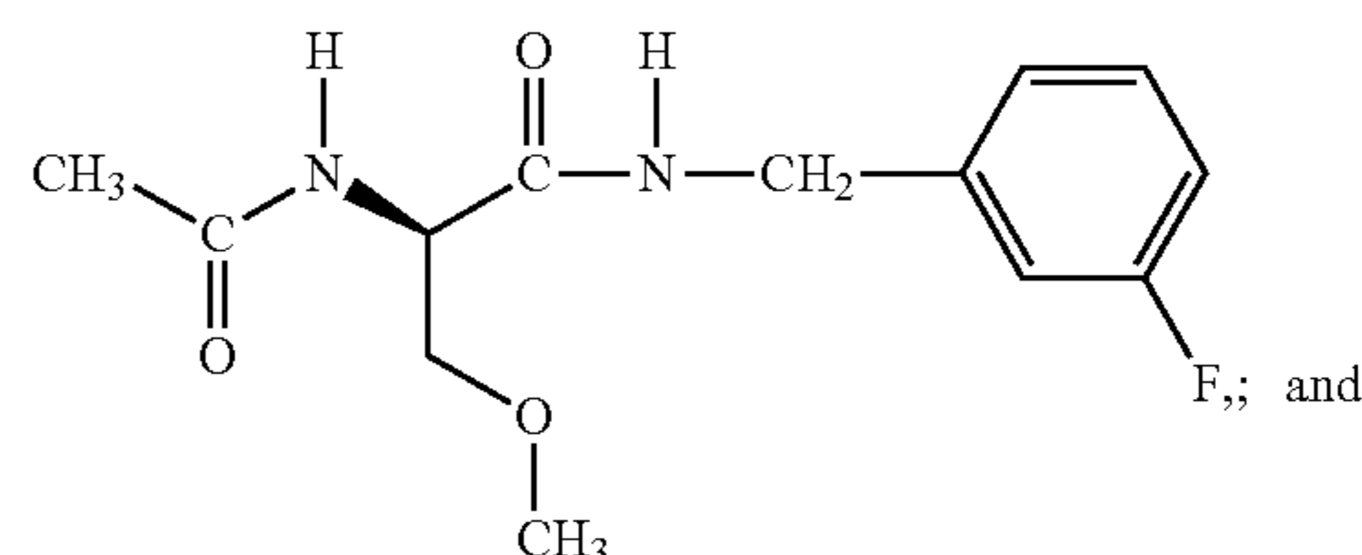
(R)-N-(3-fluorobenzyl)-2-acetamido-3-methoxy propionamide
