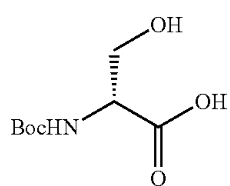
N-Boc-D-serine
