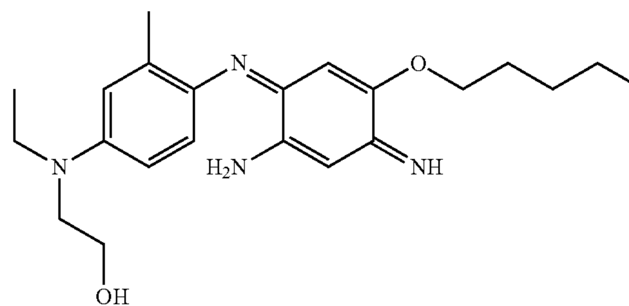
2-[[4-(2-Amino-5-hexyloxy-4-iminocyclohexa-2,5-dienylideneamino)-3-methylphenyl]ethylamino]ethanol
