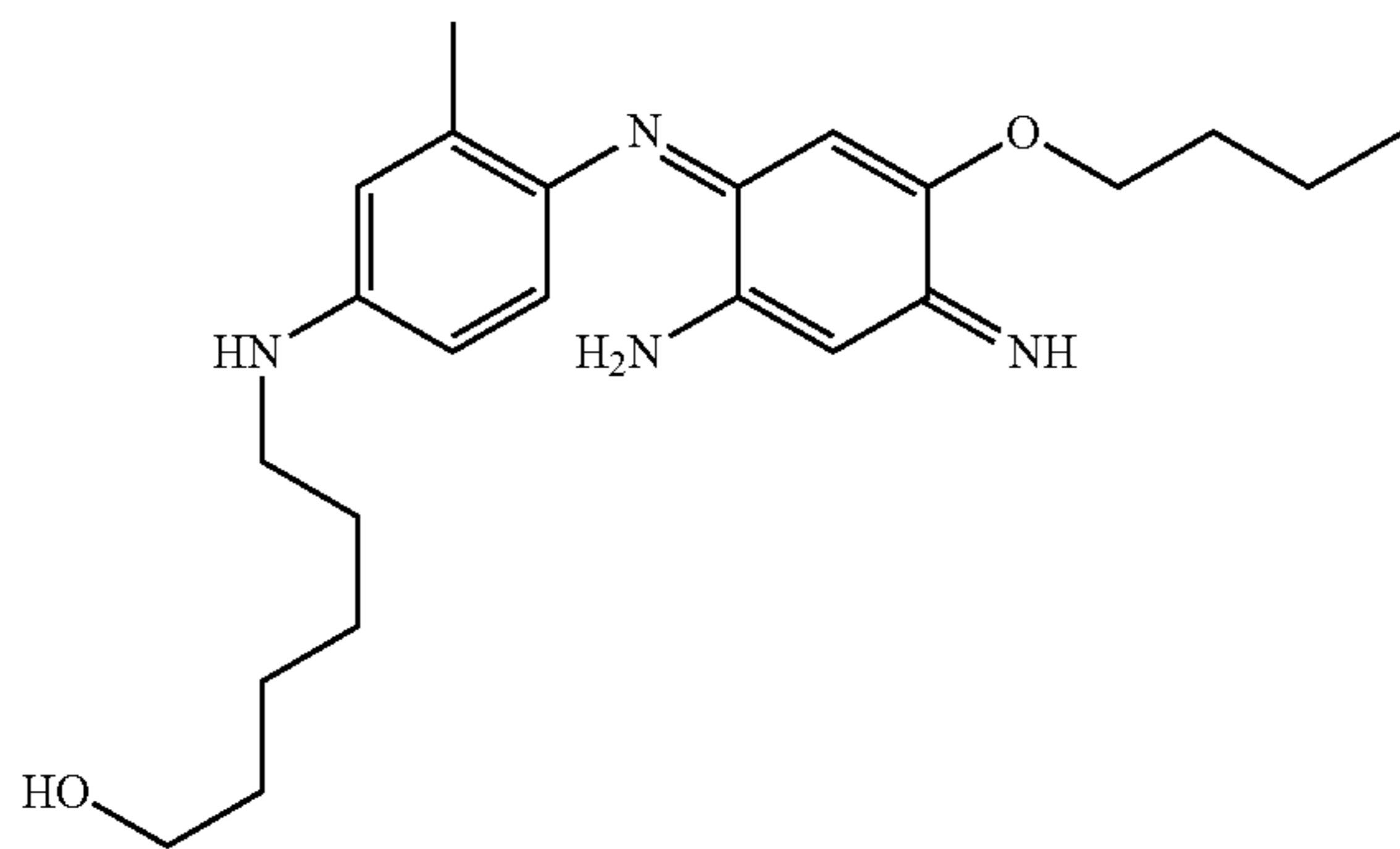
6-[4-(2-Amino-5-butoxy-4-iminocyclohexa-2,5-dienylideneamino)-3-methylphenylamino]hexan-1-ol
