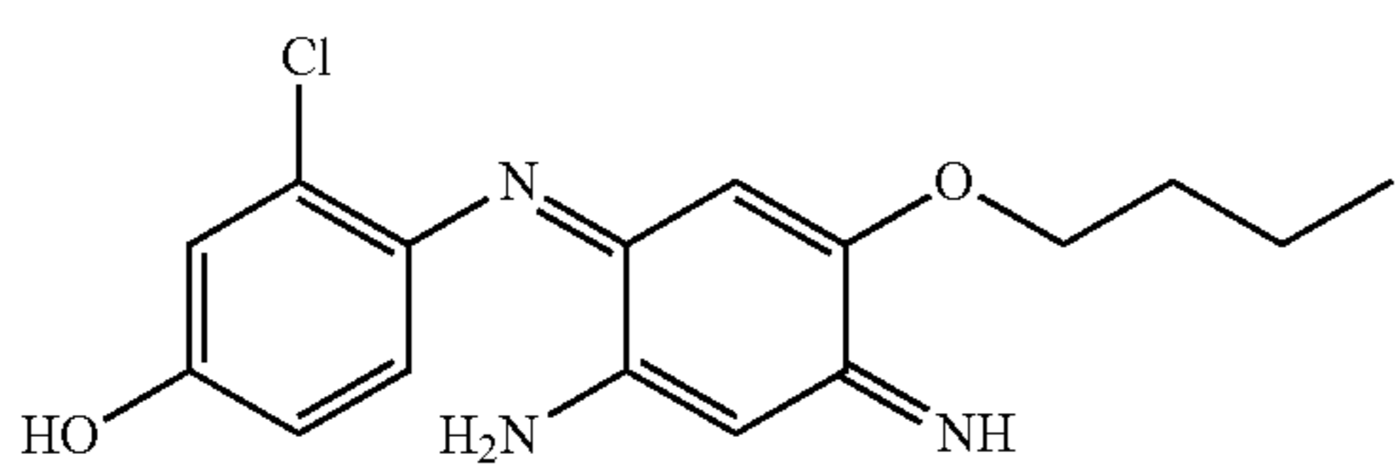
4-(2-Amino-5-butoxy-4-iminocyclohexa-2,5-dienylideneamino)-3-chlorophenol
