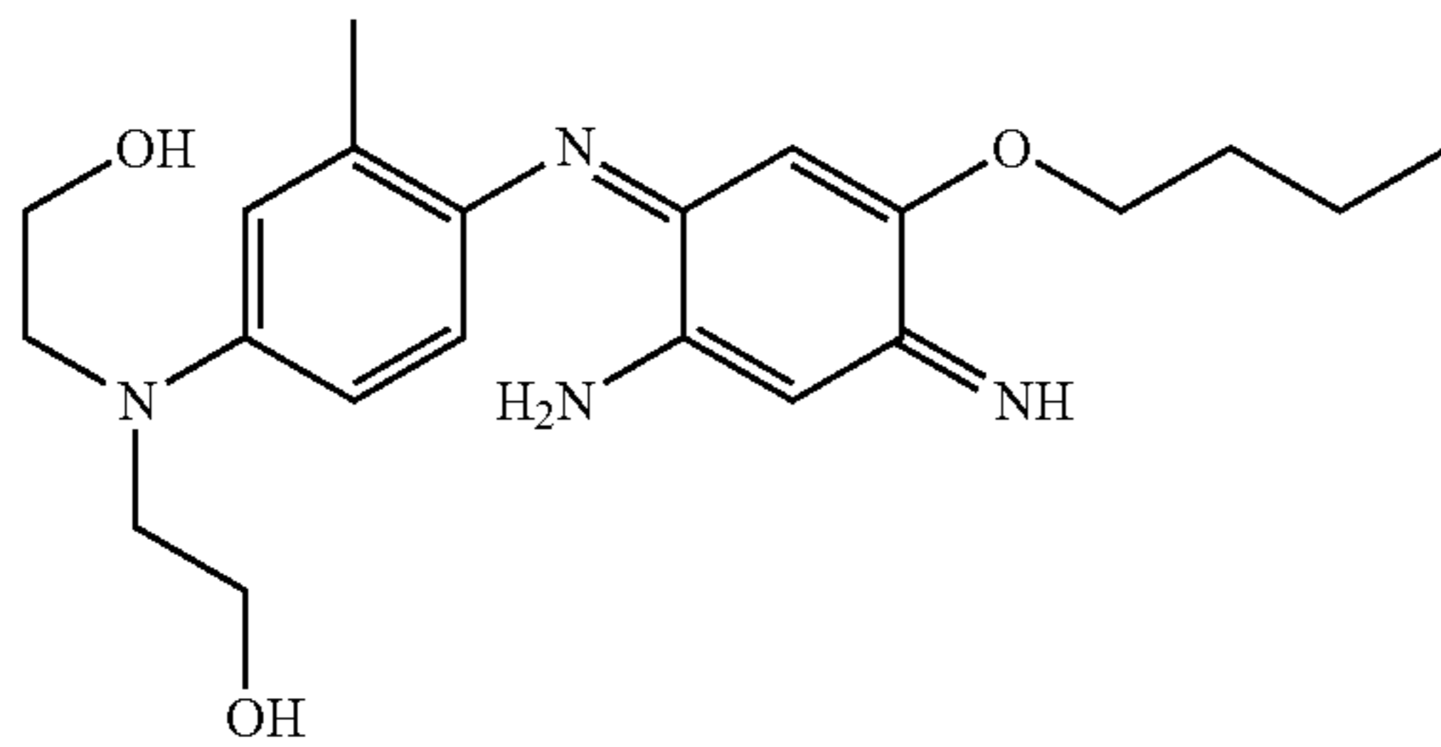
2-[[4-(2-Amino-5-butoxy-4-iminocyclohexa-2,5-dienylideneamino)-3-methylphenyl](2-hydroxyethyl)amino]ethanol
