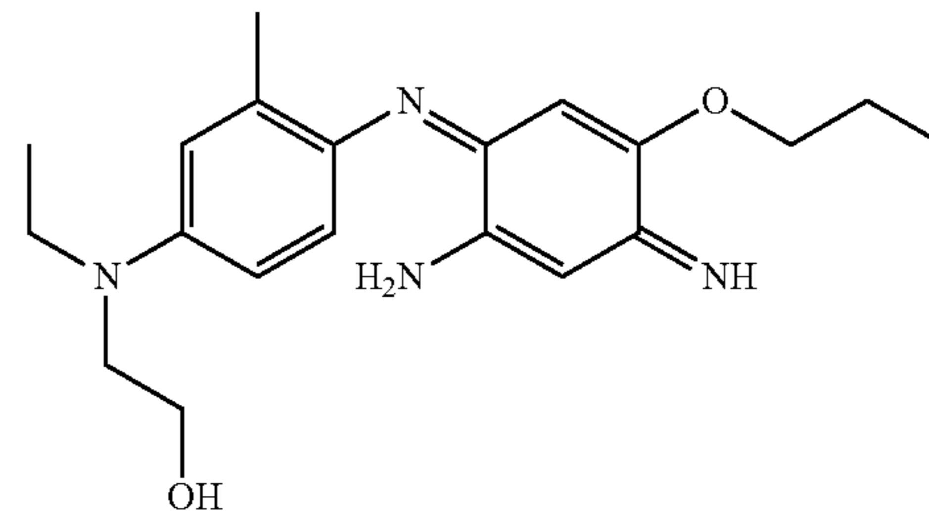
2-[[4-(2-Amino-5-propoxy-4-iminocyclohexa-2,5-dienylideneamino)-3-methylphenyl]ethylamino]ethanol
