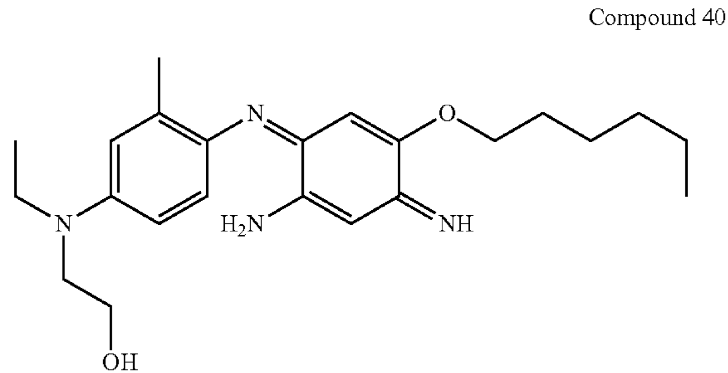
2-{[4-(2-Amino-5-hexyloxy-4-iminocyclohexa-2,5-dienylideneamino)-3-methylphenyl]ethylamino}ethanol
