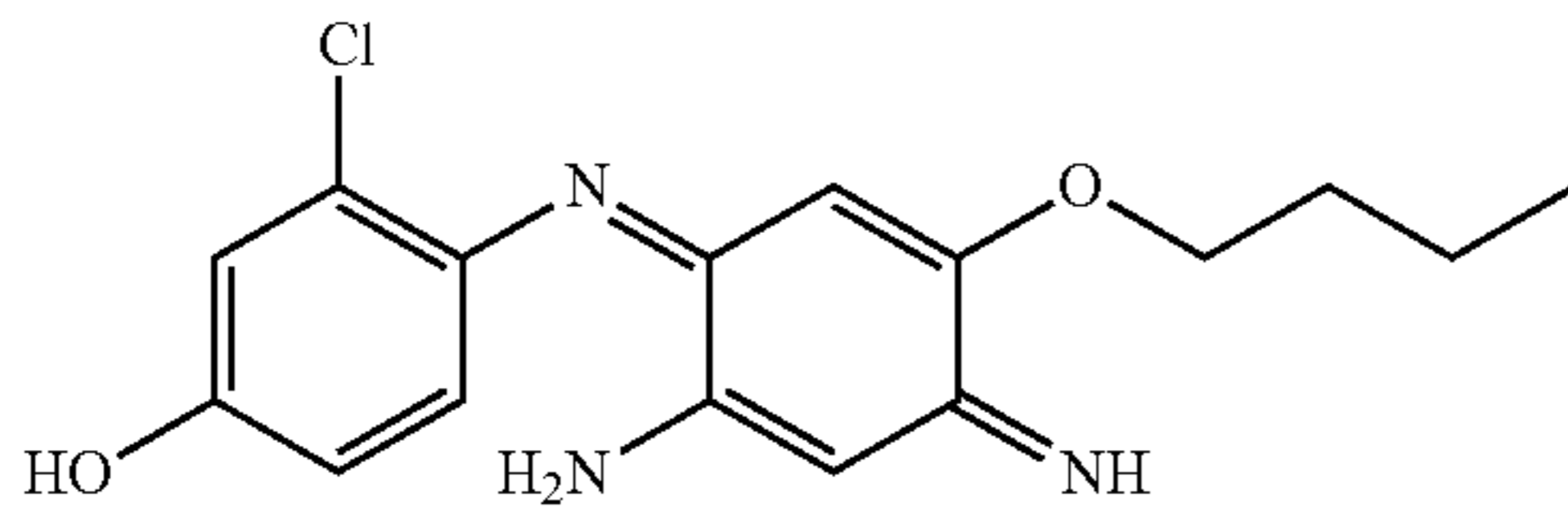
4-(2-Amino-5-butoxy-4-iminocyclohexa-2,5-dienylideneamino)-3-chlorophenol
