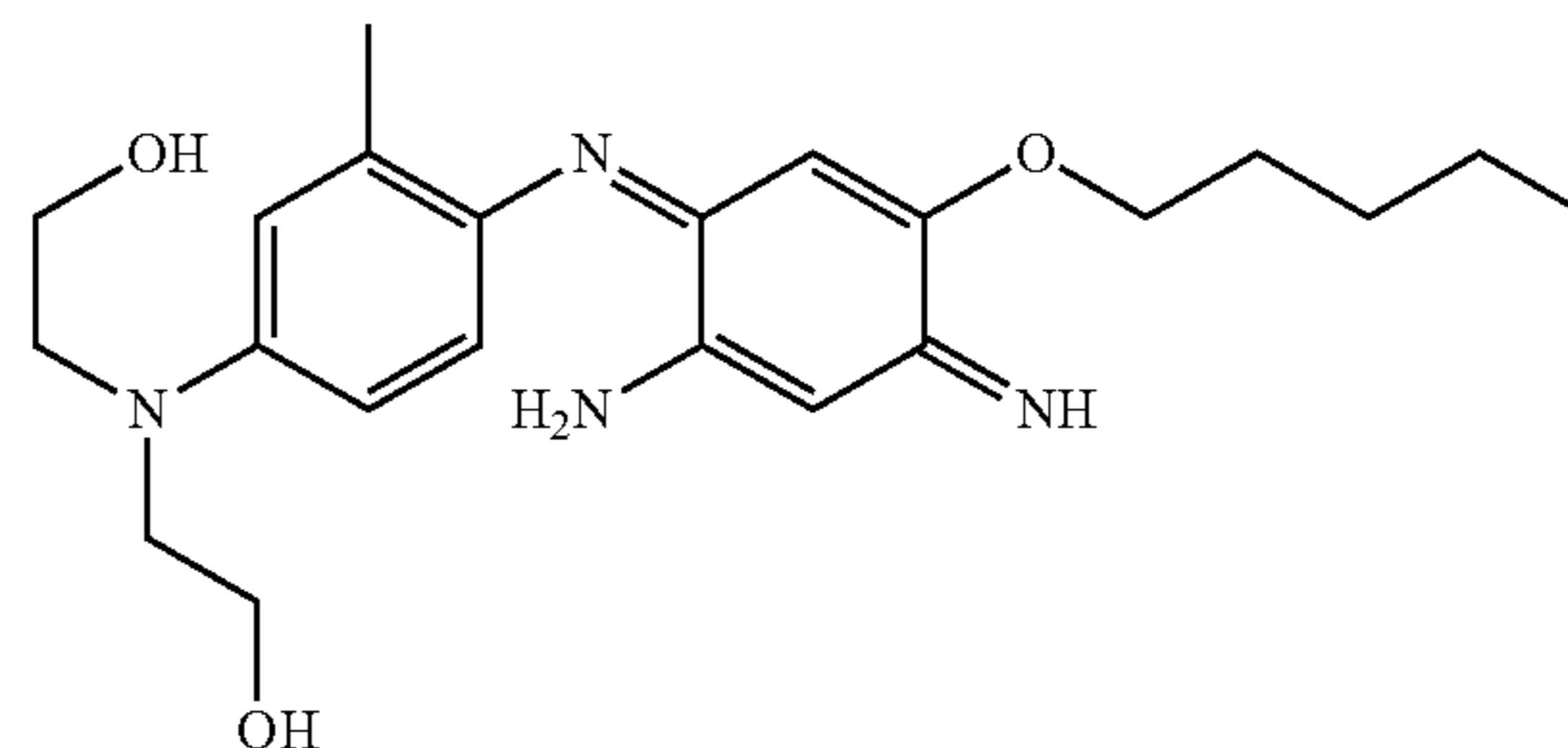
2-[[4-(2-Amino-5-hexyloxy-4-iminocyclohexa-2,5-dienylideneamino)-3-methylphenyl](2-hydroxyethyl)amino]ethanol
