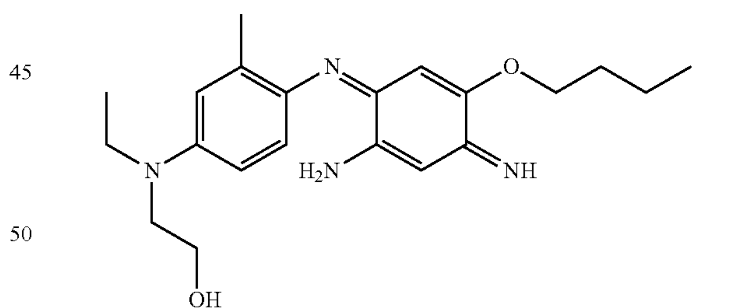
2-[[4-(2-Amino-5-butoxy-4-iminocyclohexa-2,5-dienylideneamino)-3-methylphenyl]ethylamino]ethanol
