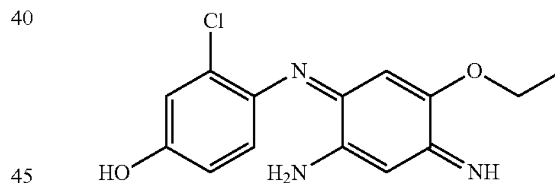
4-(2-Amino-5-ethoxy-4-iminocyclohexa-2,5-dienylideneamino)-3-chlorophenol
