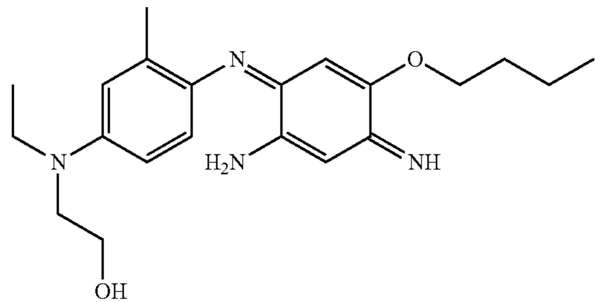
2-([4-(2-Amino-5-butoxy-4-iminocyclohexa-2,5-dienylideneamino)-3-methylphenyl]ethylamino)ethanol
