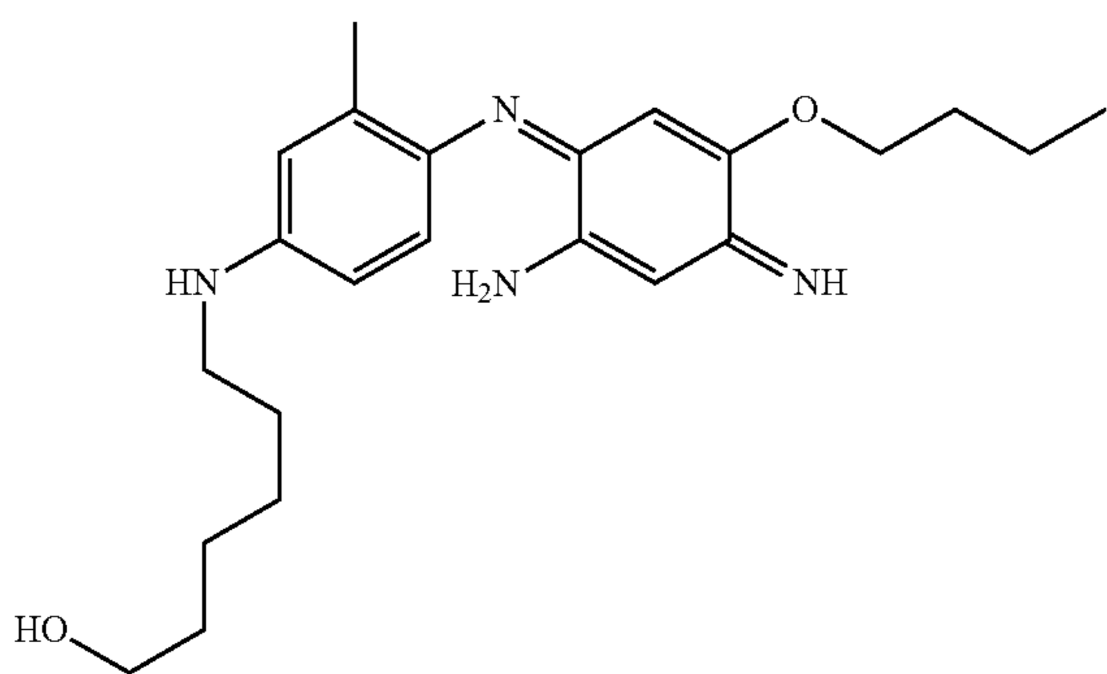
6-[4-(2-Amino-5-butoxy-4-iminocyclohexa-2,5-dienylideneamino)-3-methylphenylamino]hexan-1-ol
