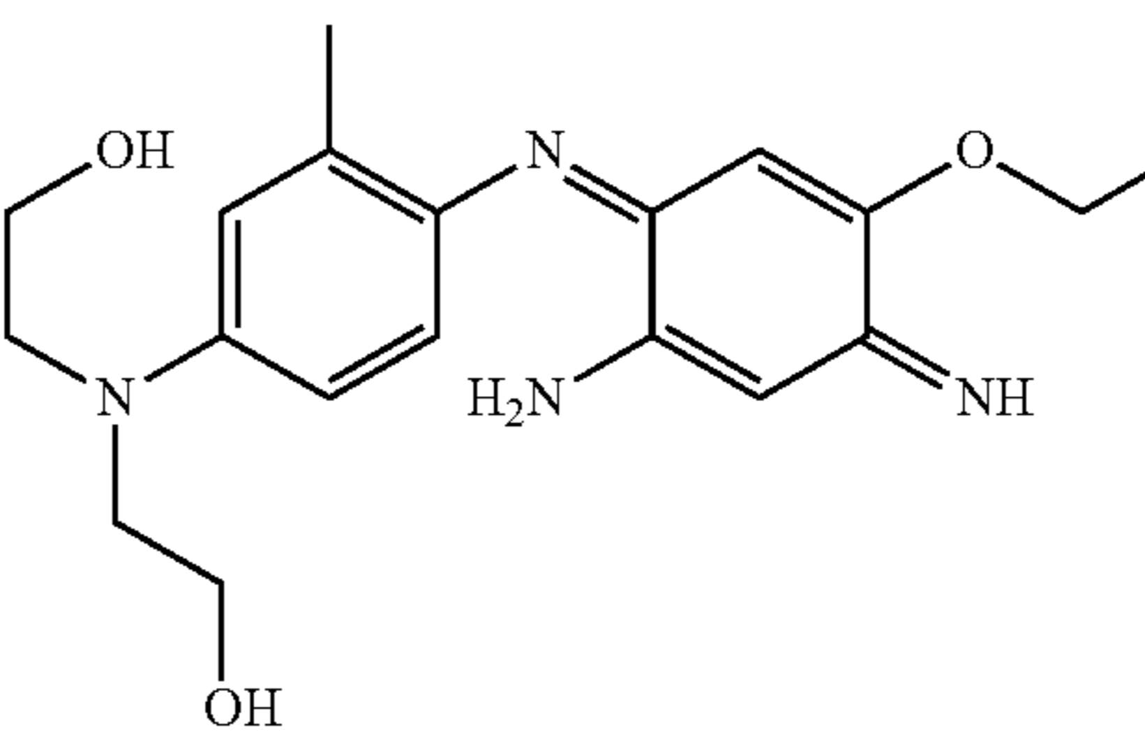
2-[[4-(2-Amino-5-ethoxy-4-iminocyclohexa-2,5-dienylideneamino)-3-methylphenyl](2-hydroxyethyl)amino]ethanol
