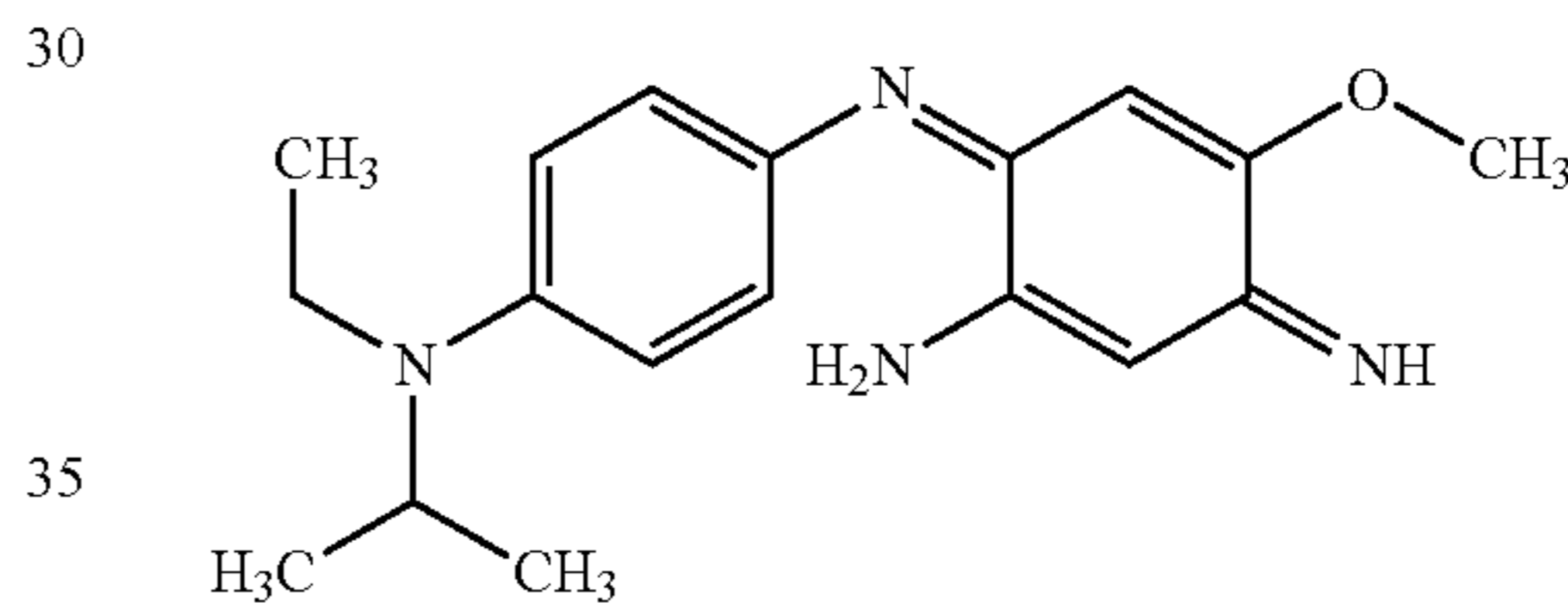
4-methoxy-6-[4-(N-ethyl-N-isopropylamino)phenylimino]-3-iminocyclohexa-1,4-dienyl-1-amine
