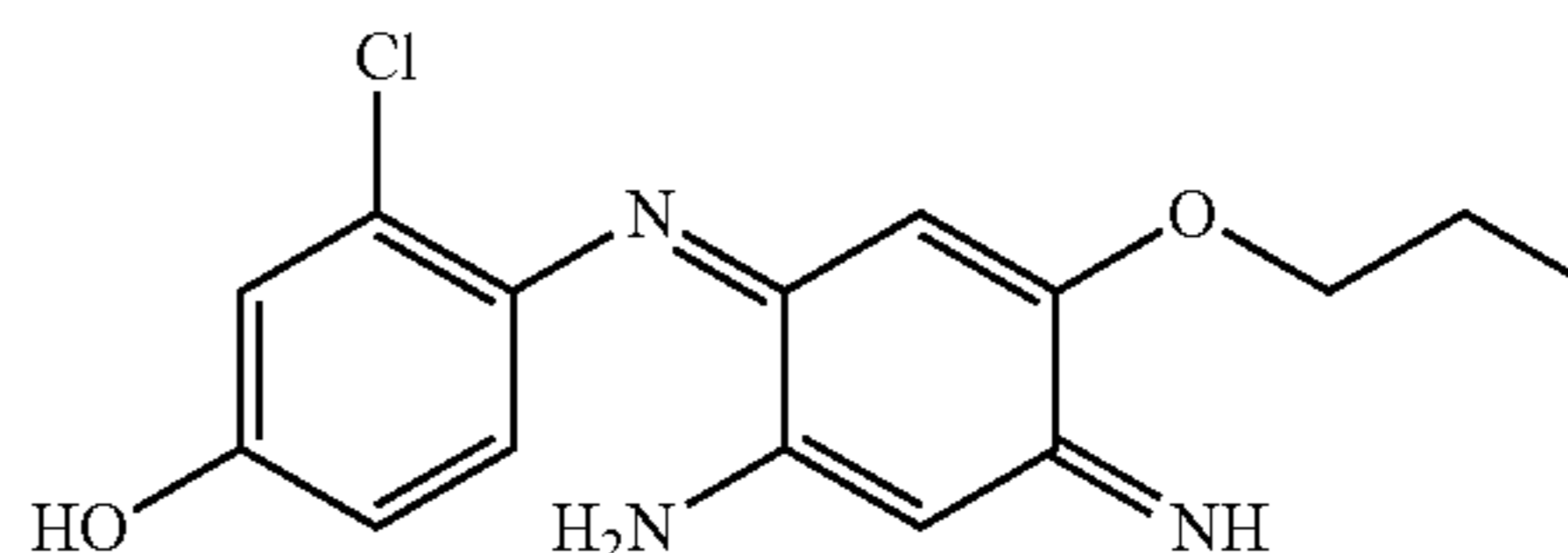
4-(2-Amino-5-propoxy-4-iminocyclohexa-2,5-dienylideneamino)-3-chlorophenol
