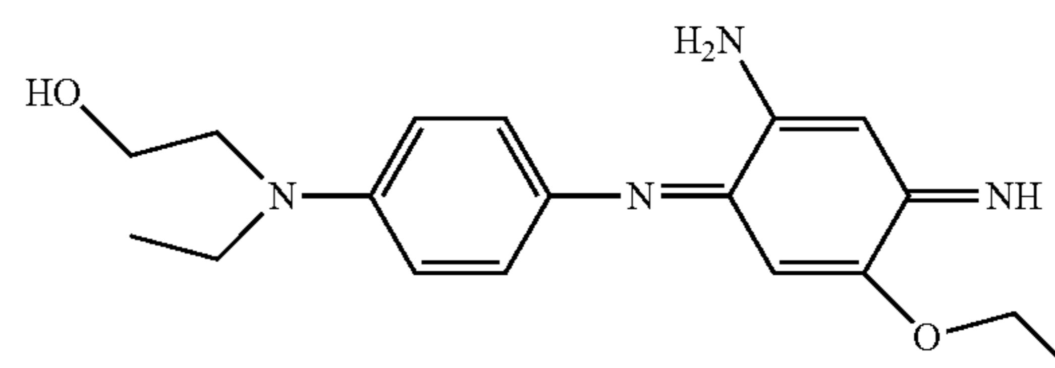
2-[[4-(2-Amino-5-ethoxy-4-iminocyclohexa-2,5-dienylideneamino)phenyl]ethylamino]ethanol
