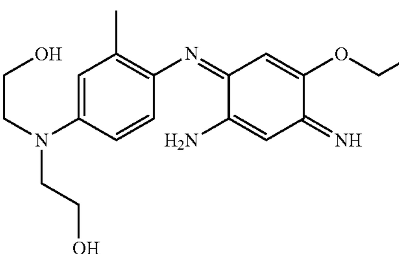
2-[[4-(2-Amino-5-ethoxy-4-iminocyclohexa-2,5-dienylideneamino)-3-methylphenyl](2-hydroxyethyl)amino]ethanol
