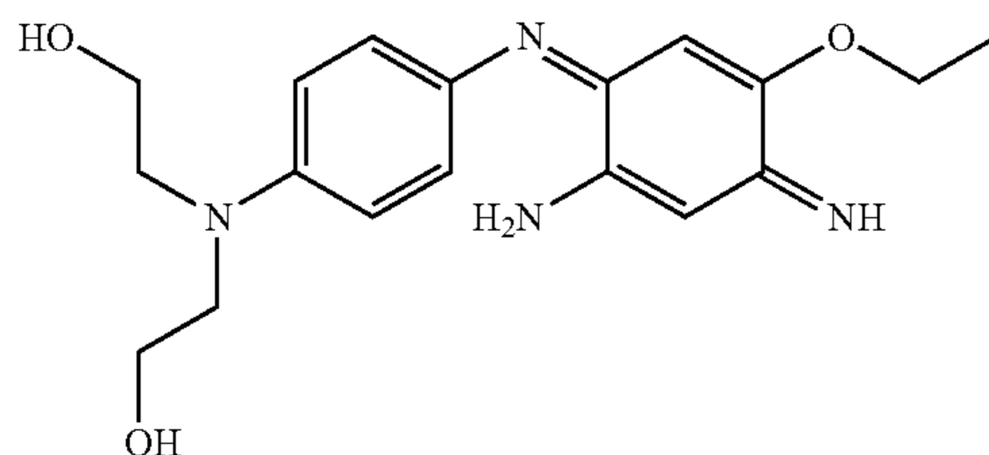
2-[[4-(2-Amino-5-ethoxy-4-aminocyclohexa-2,5-dienylideneamino)phenyl](2-hydroxyethyl)amino]ethanol
