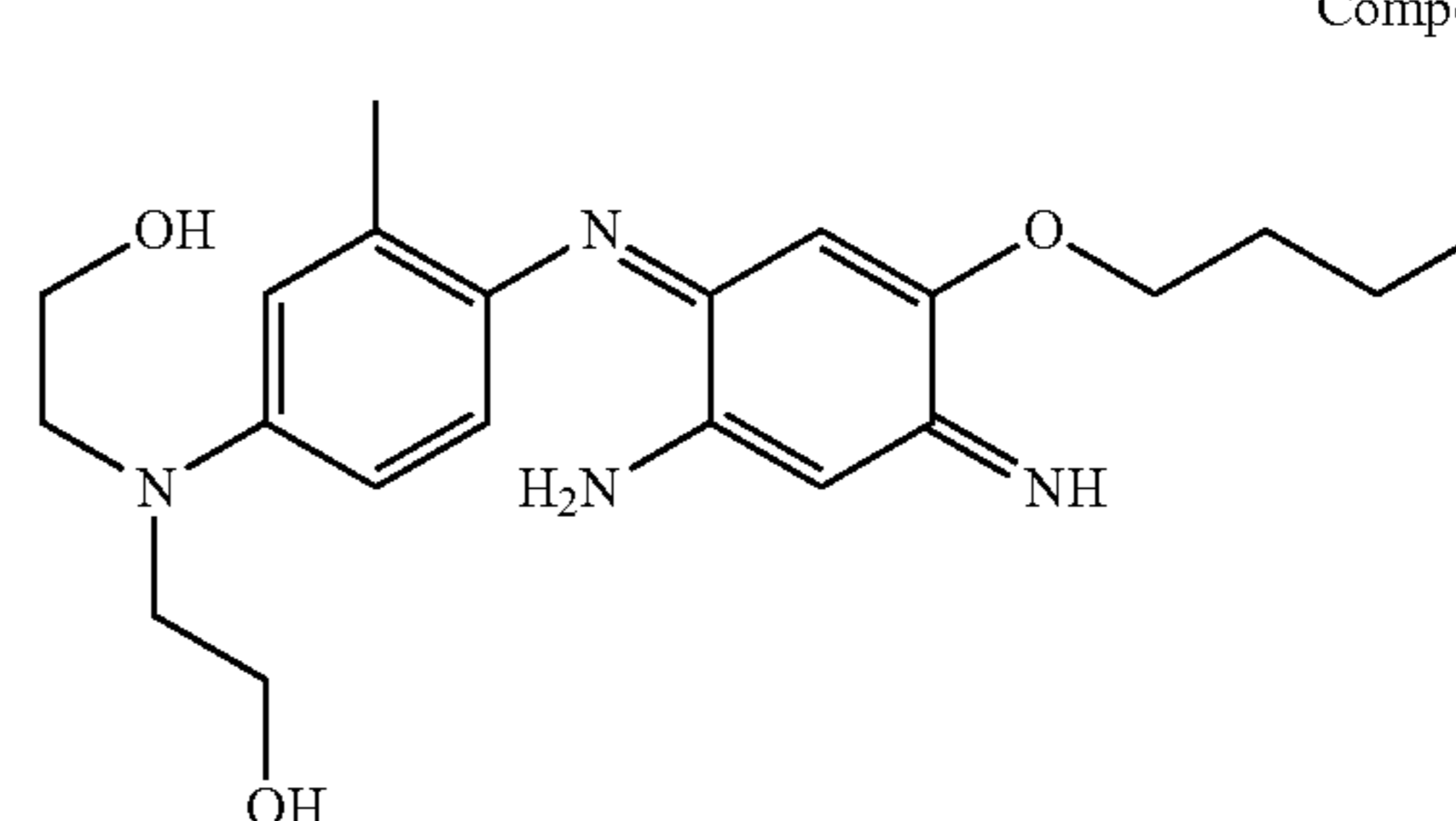
2-([4-(2-Amino-5-butoxy-4-iminocyclohexa-2,5-dienylideneamino)-3-methylphenyl](2-hydroxyethyl)amino)ethanol
