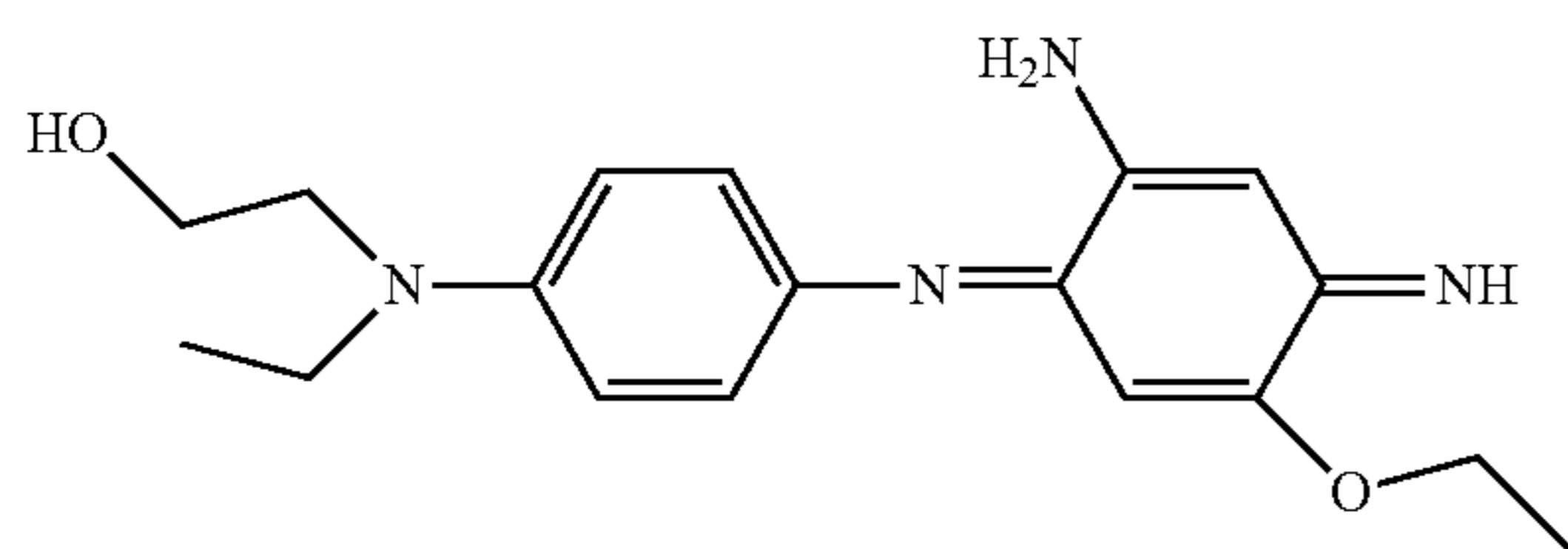
2-([4-(2-Amino-5-ethoxy-4-iminocyclohexa-2,5-dienylideneamino)phenyl]ethylamino)ethanol
