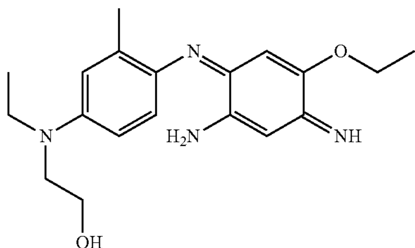
2-[[4-(2-Amino-5-ethoxy-4-iminocyclohexa-2,5-dienylideneamino)-3-methylphenyl]ethylamino]ethanol
