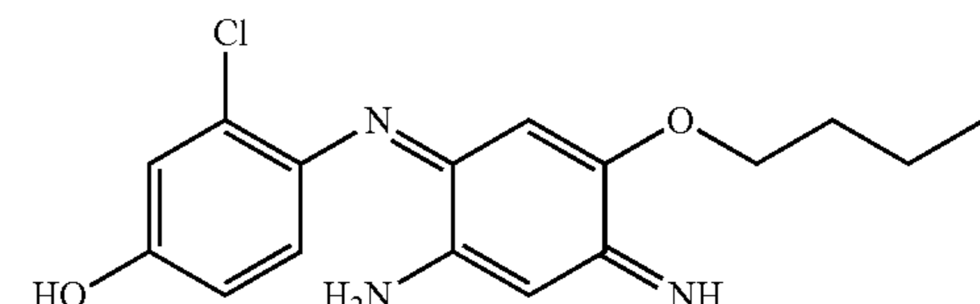
4-(2-Amino-5-butoxy-4-iminocyclohexa-2,5-dienylideneamino)-3-chlorophenol
