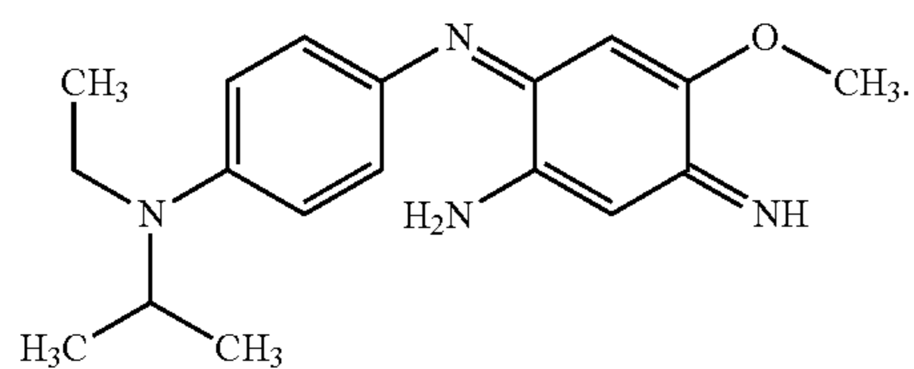
4-methoxy-6-[4-(N-ethyl-N-isopropylamino)phenylimino]-3-iminocyclohexa-1,4-dienyl-1-amine
