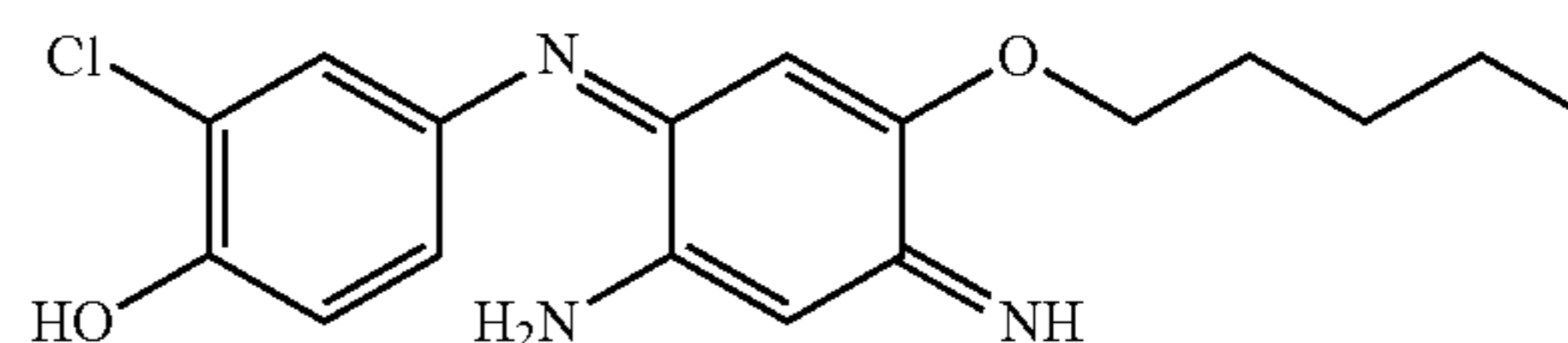
4-(2-Amino-5-hexyloxy-4-iminocyclohexa-2,5-dienylideneamino)-2-chlorophenol
