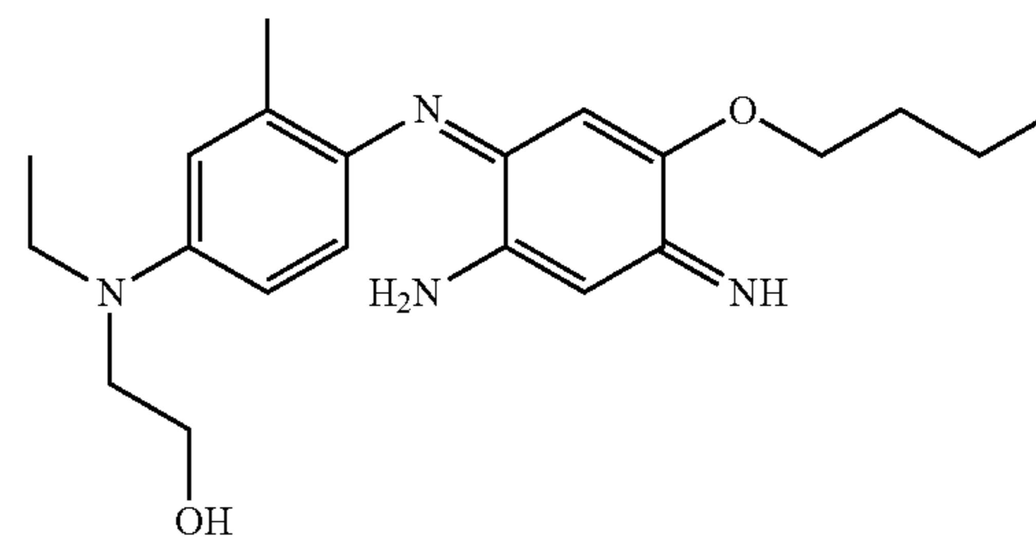
2-[[4-(2-Amino-5-butoxy-4-iminocyclohexa-2,5-dienylideneamino)-3-methylphenyl]ethylamino]ethanol
