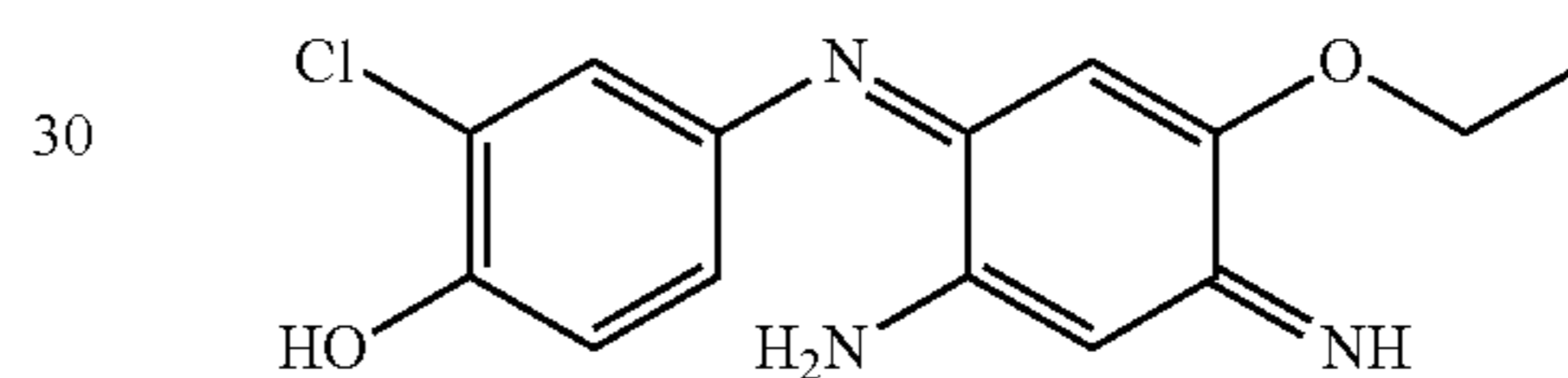
4-(2-Amino-5-ethoxy-4-iminocyclohexa-2,5-dienylideneamino)-2-chlorophenol
