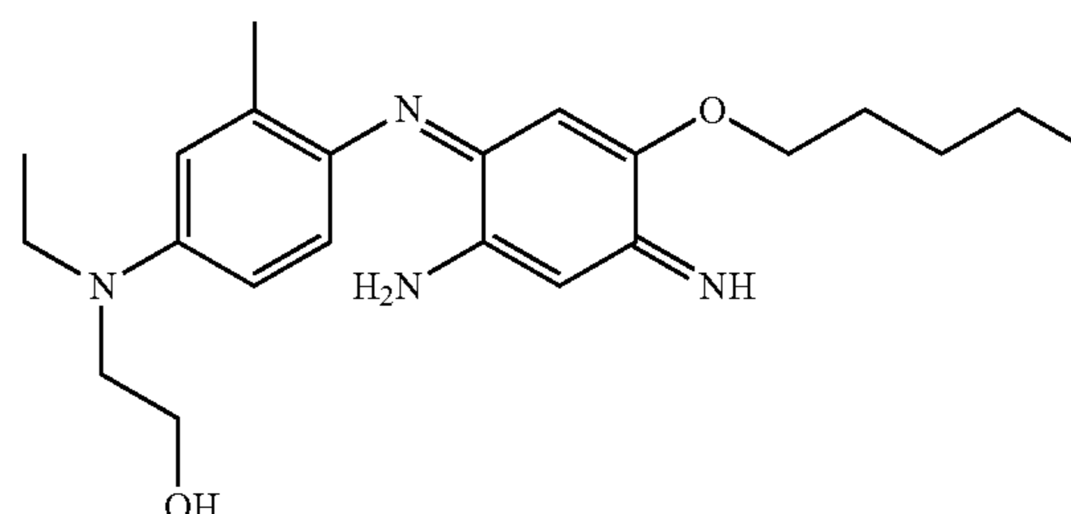
2-[[4-(2-Amino-5-pentyloxy-4-aminocyclohexa-2,5-dienylideneamino)-3-methylphenyl]ethylamino]ethanol
