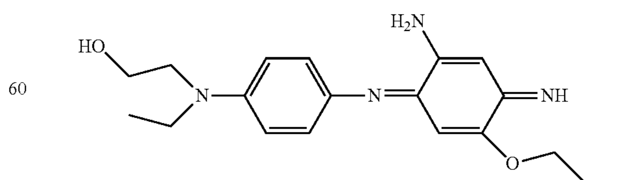
2-[[4-(2-Amino-5-ethoxy-4-iminocyclohexa-2,5-dienylideneamino)phenyl]ethylamino]ethanol
