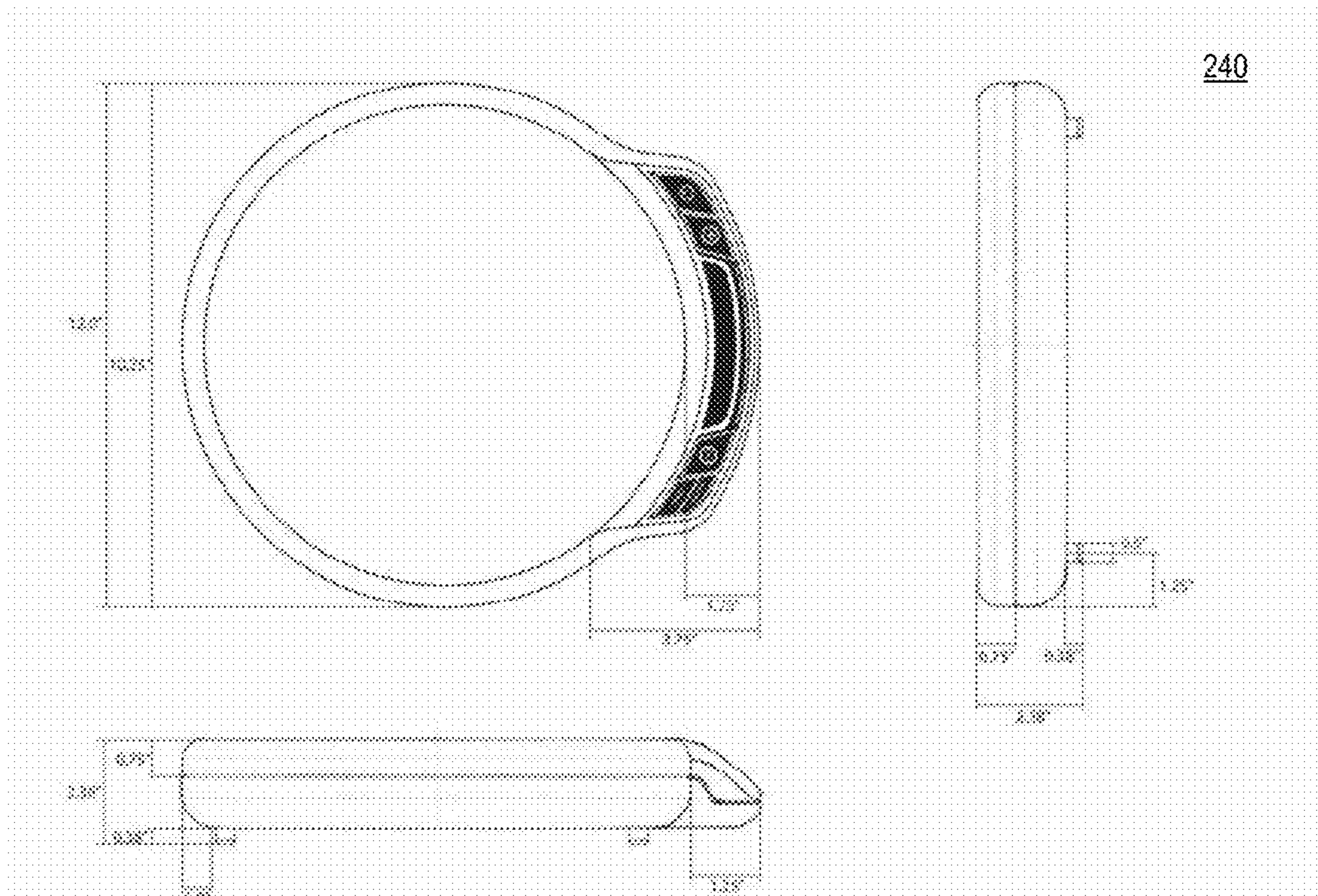
FIG. 2C
