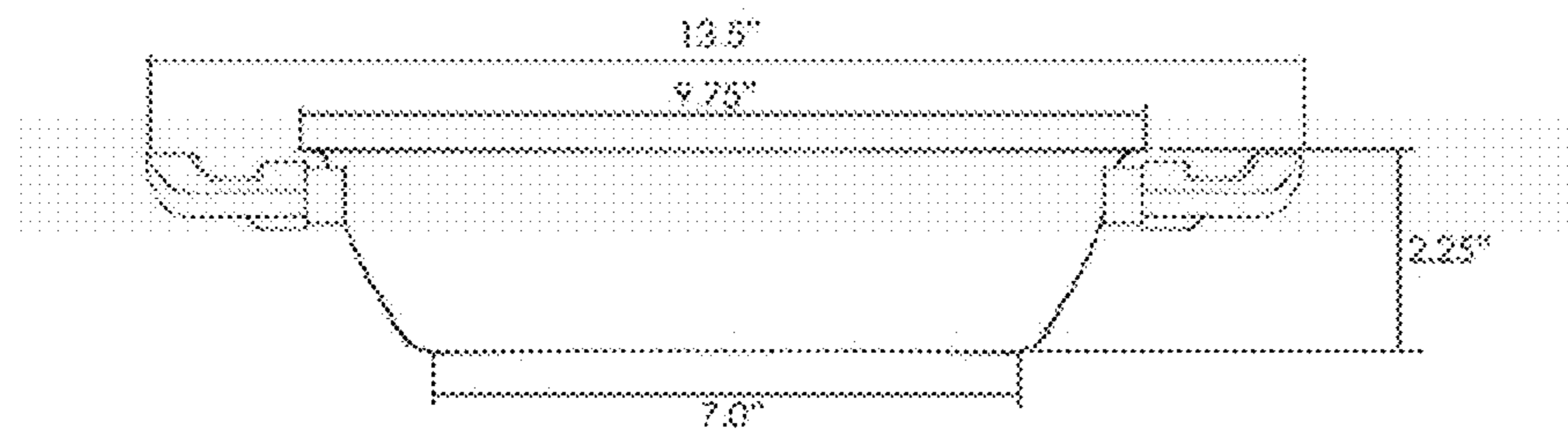
FIG. 12E
