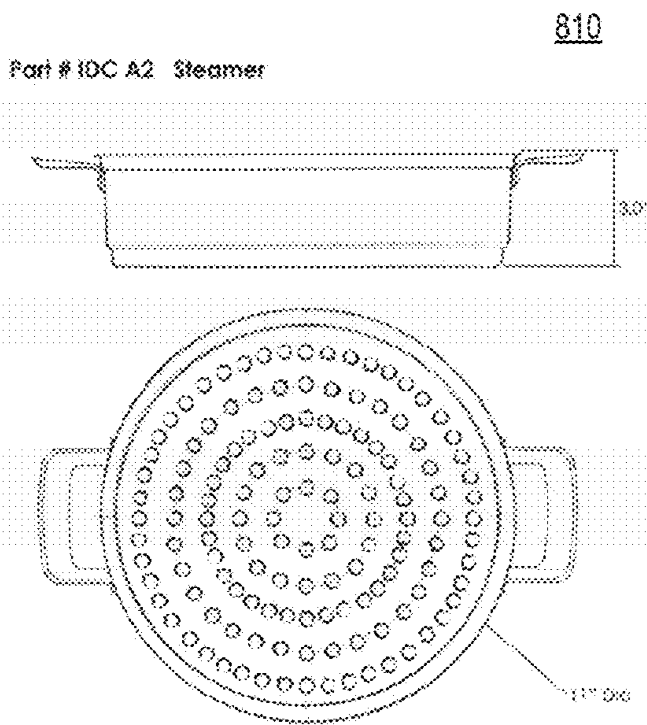
FIG. 8B
