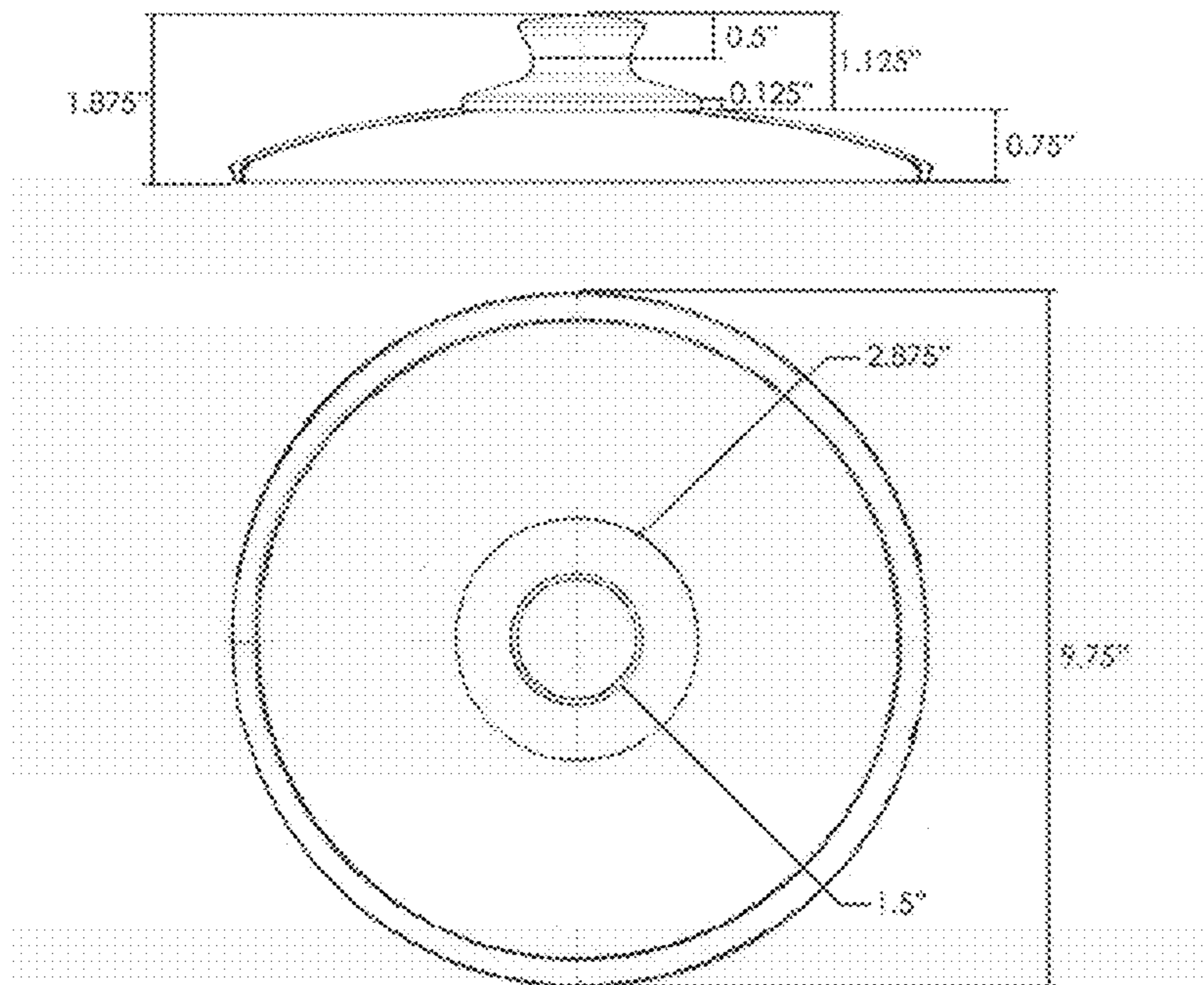
FIG. 12C
