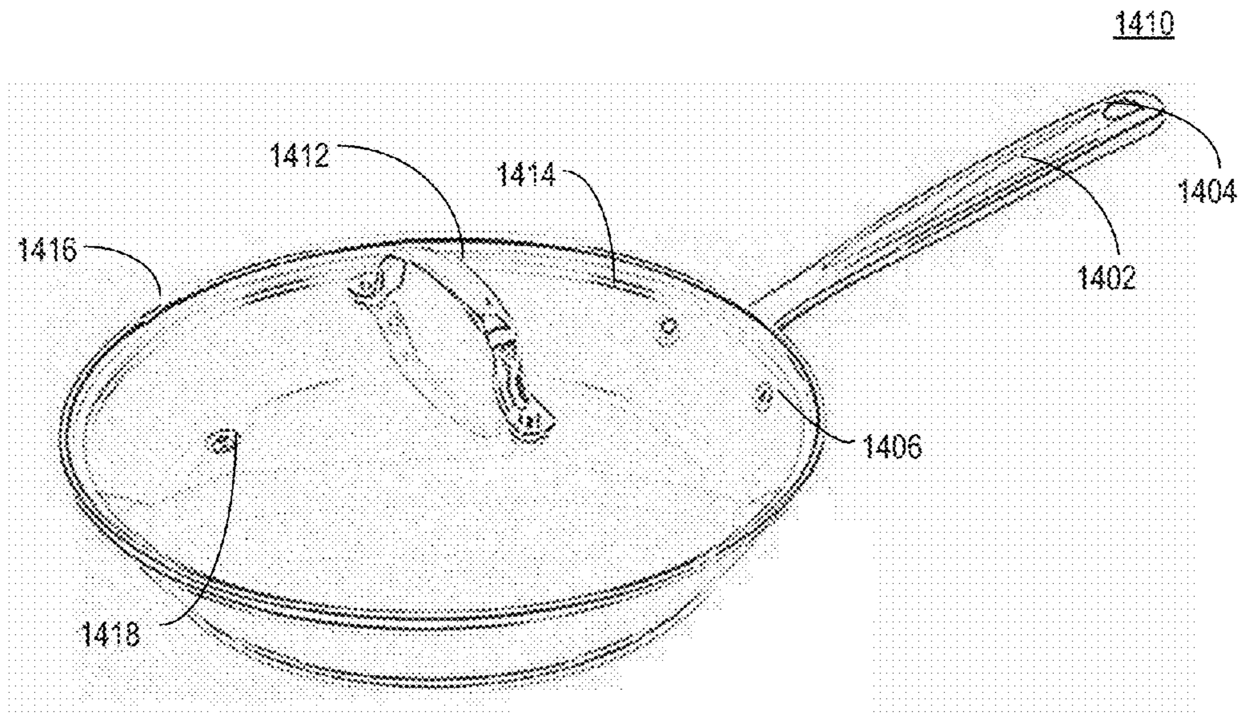
FIG. 14C
