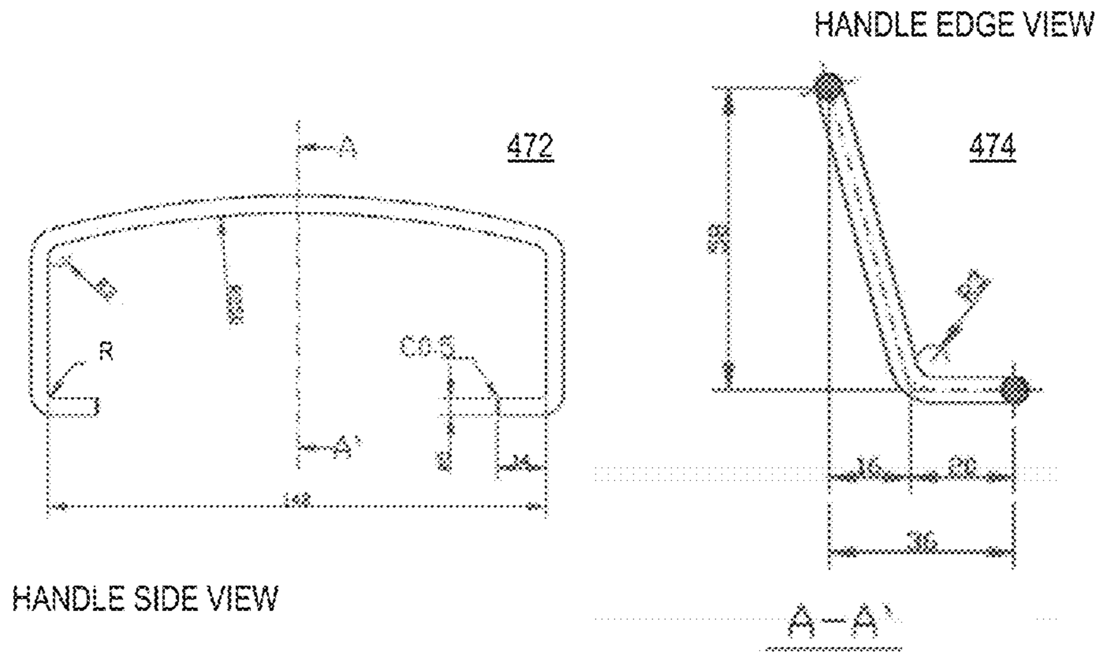
FIG. 4F
