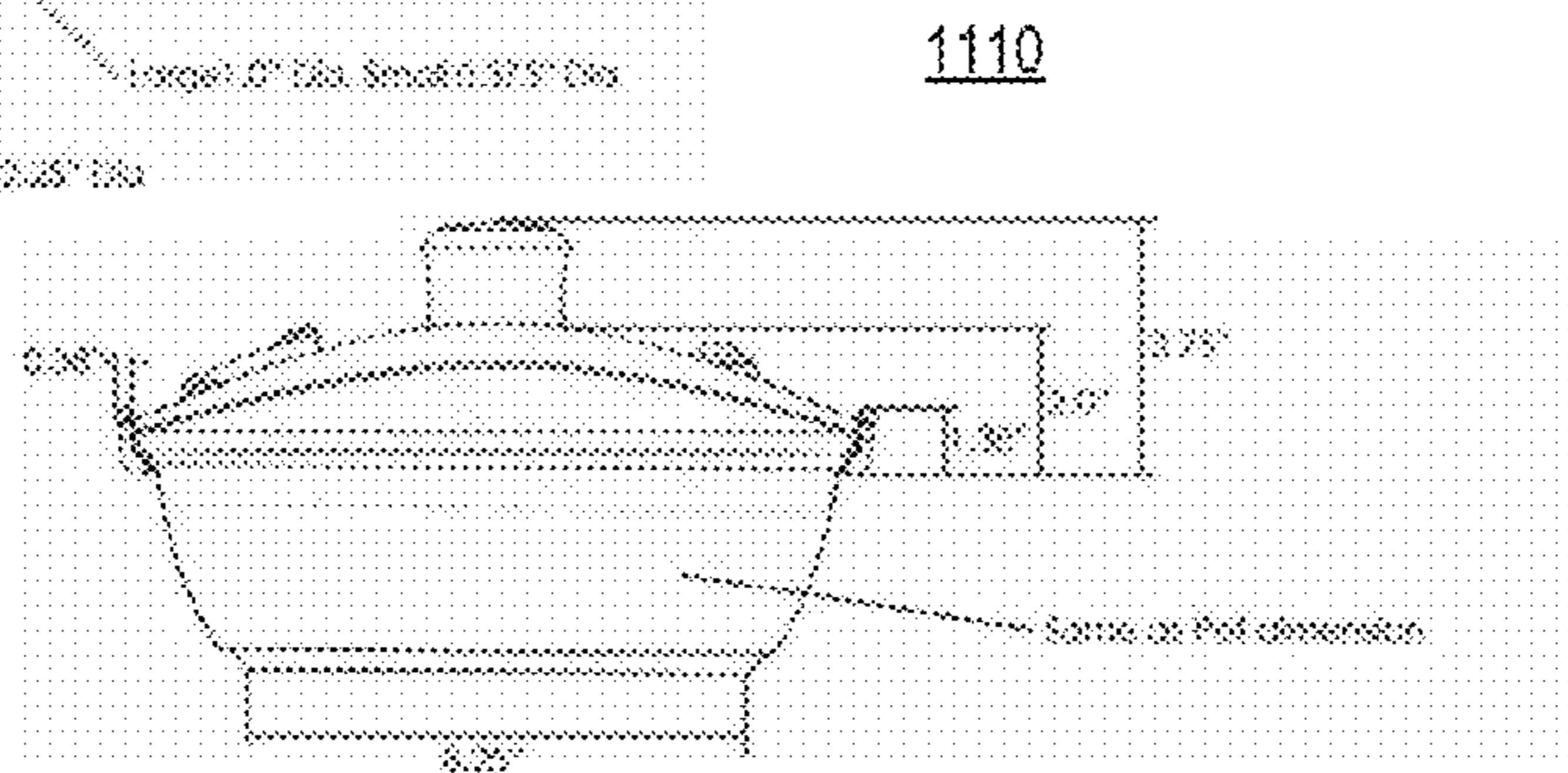
FIG. 11B1
