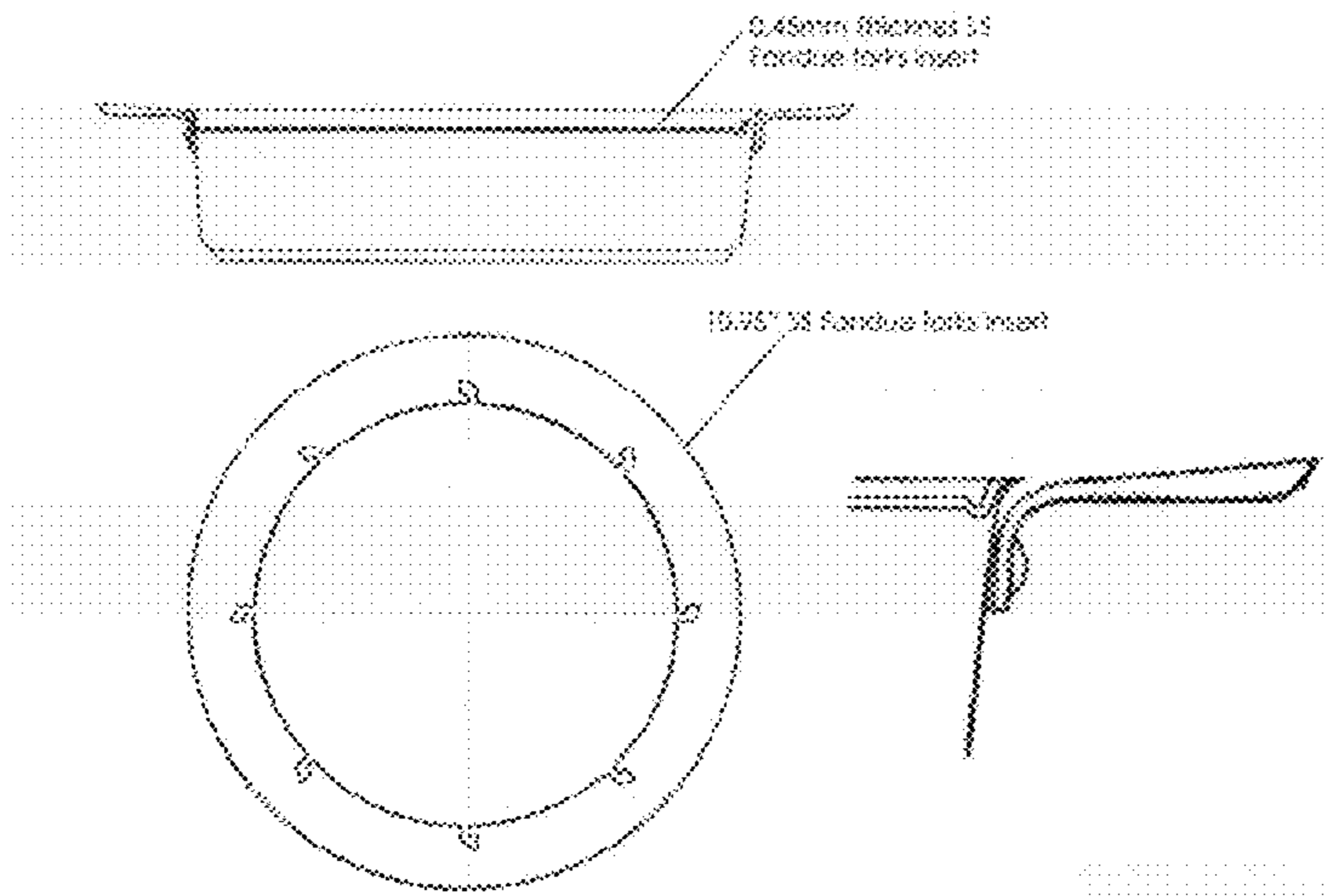
Part # 106 A5 Fondue Plate
