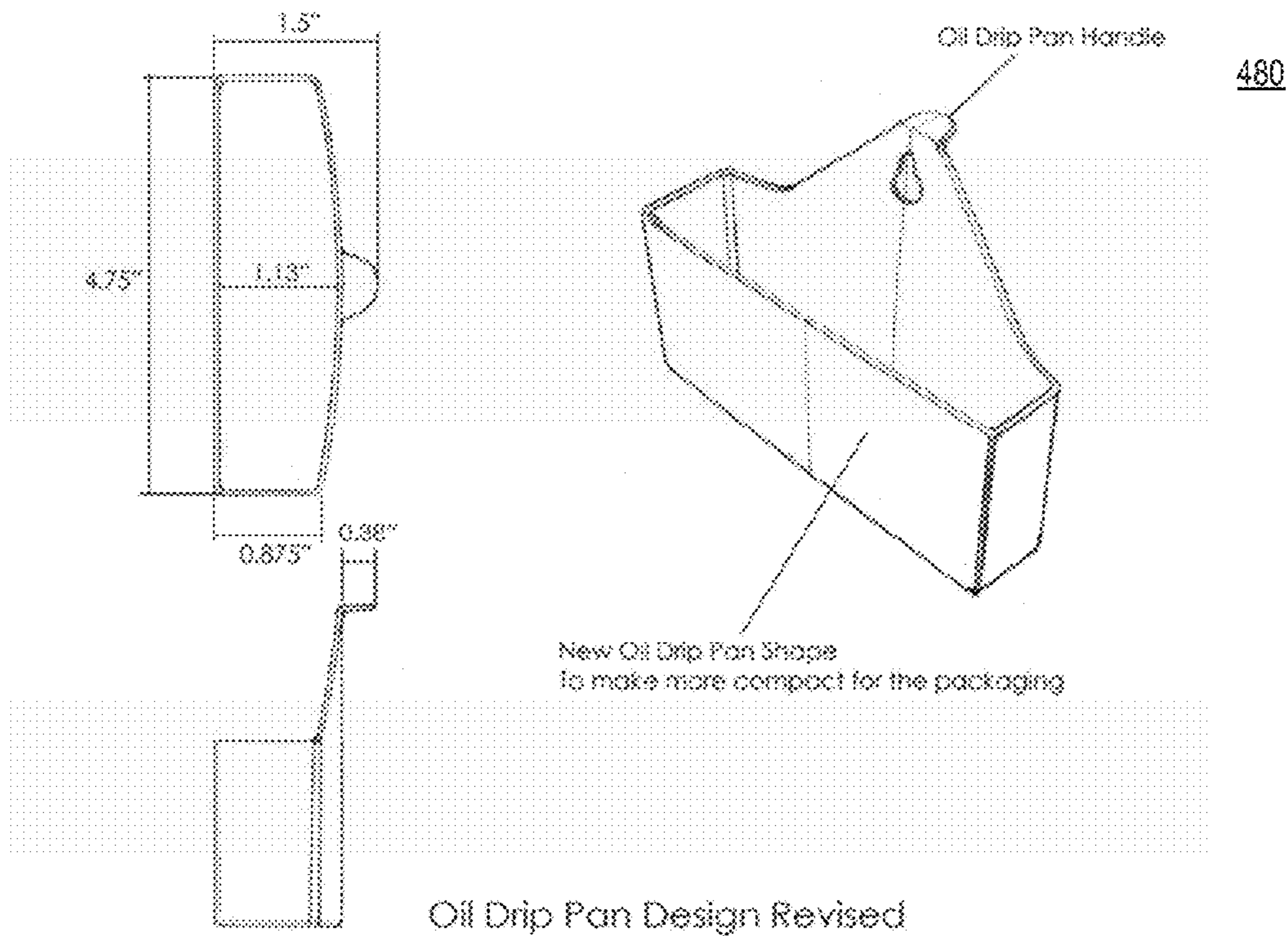
FIG. 4G
