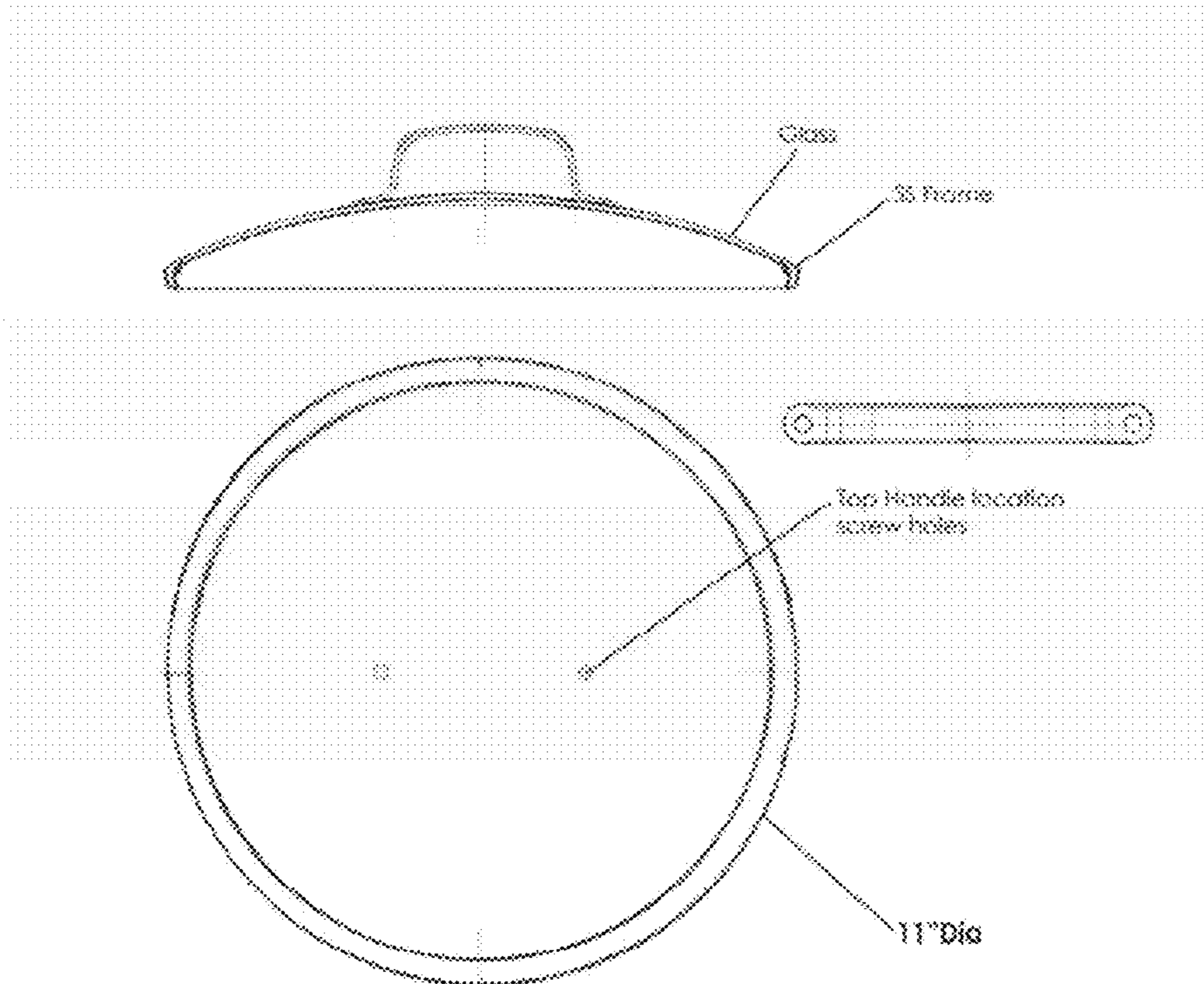
FIG. 10C
