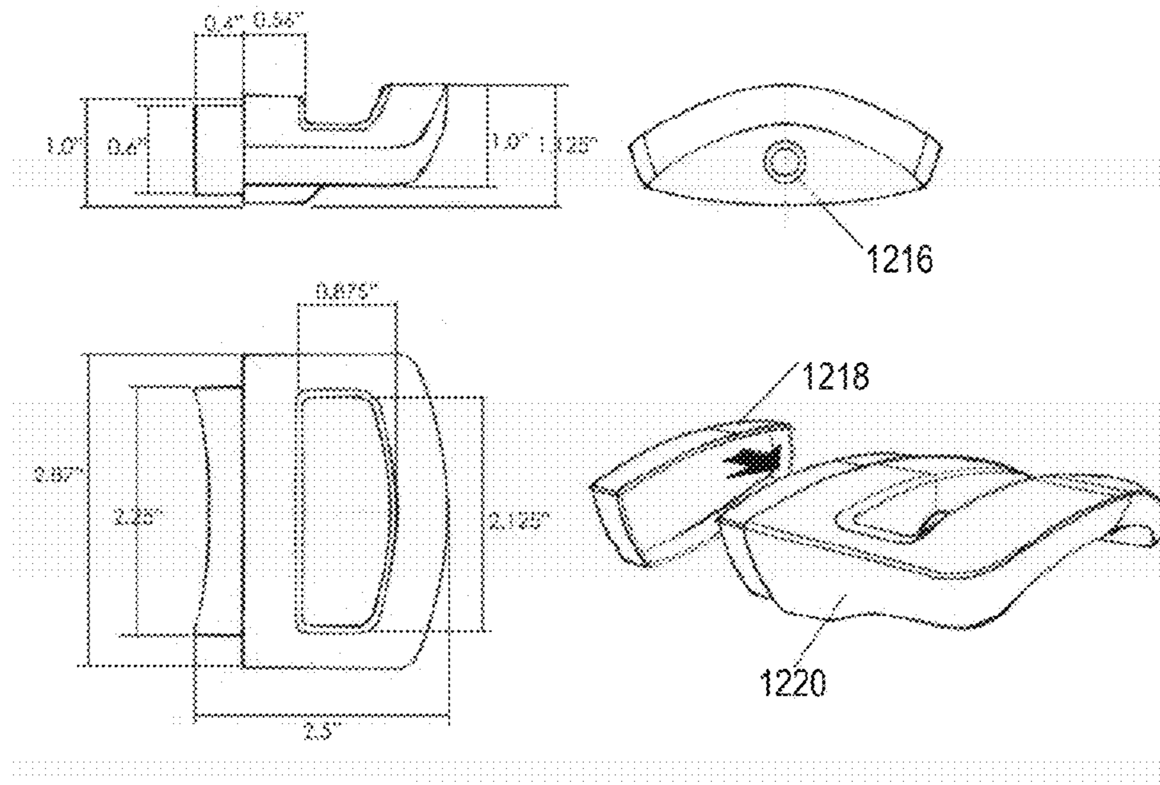
FIG. 12C
