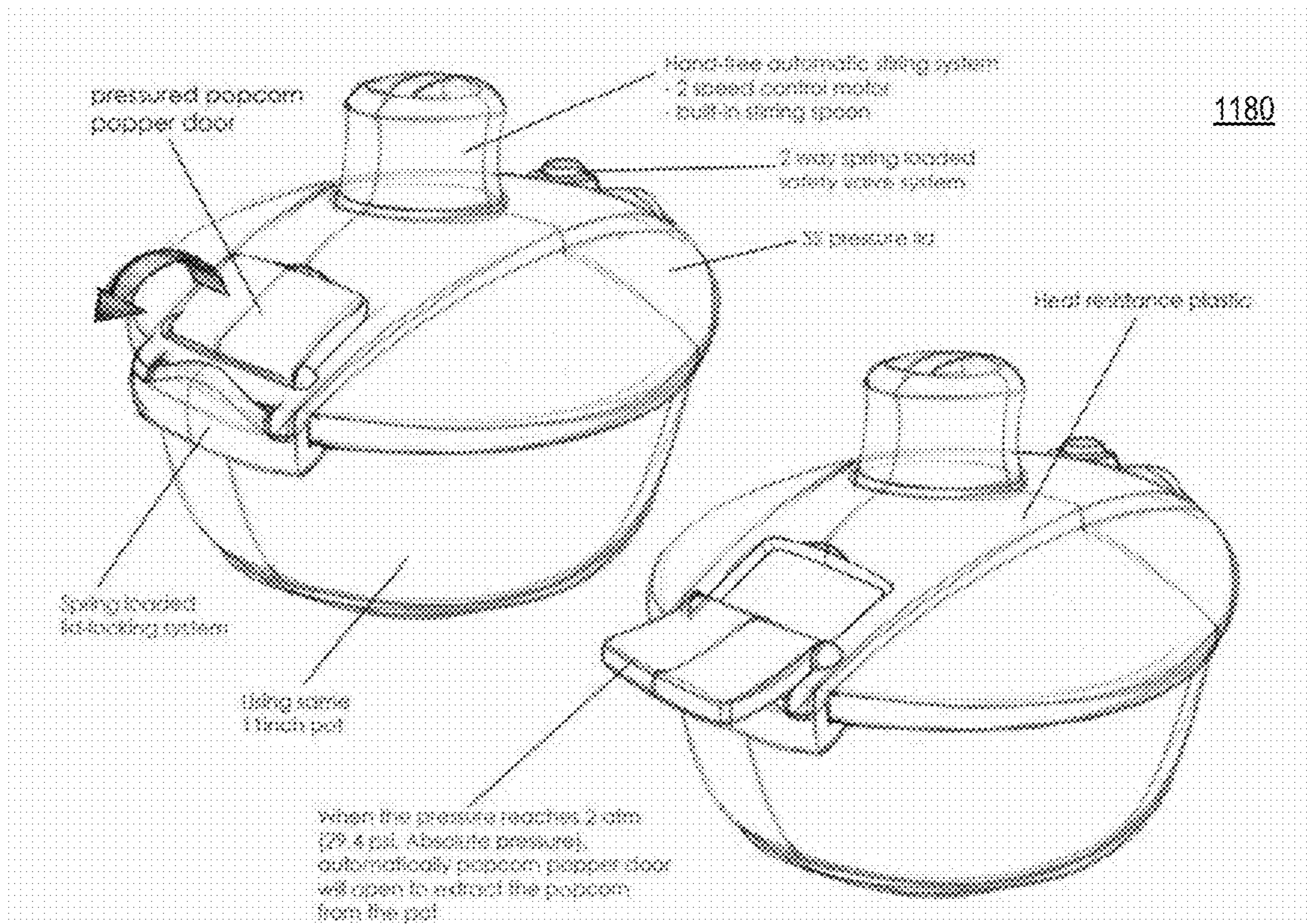
FIG. 11E
