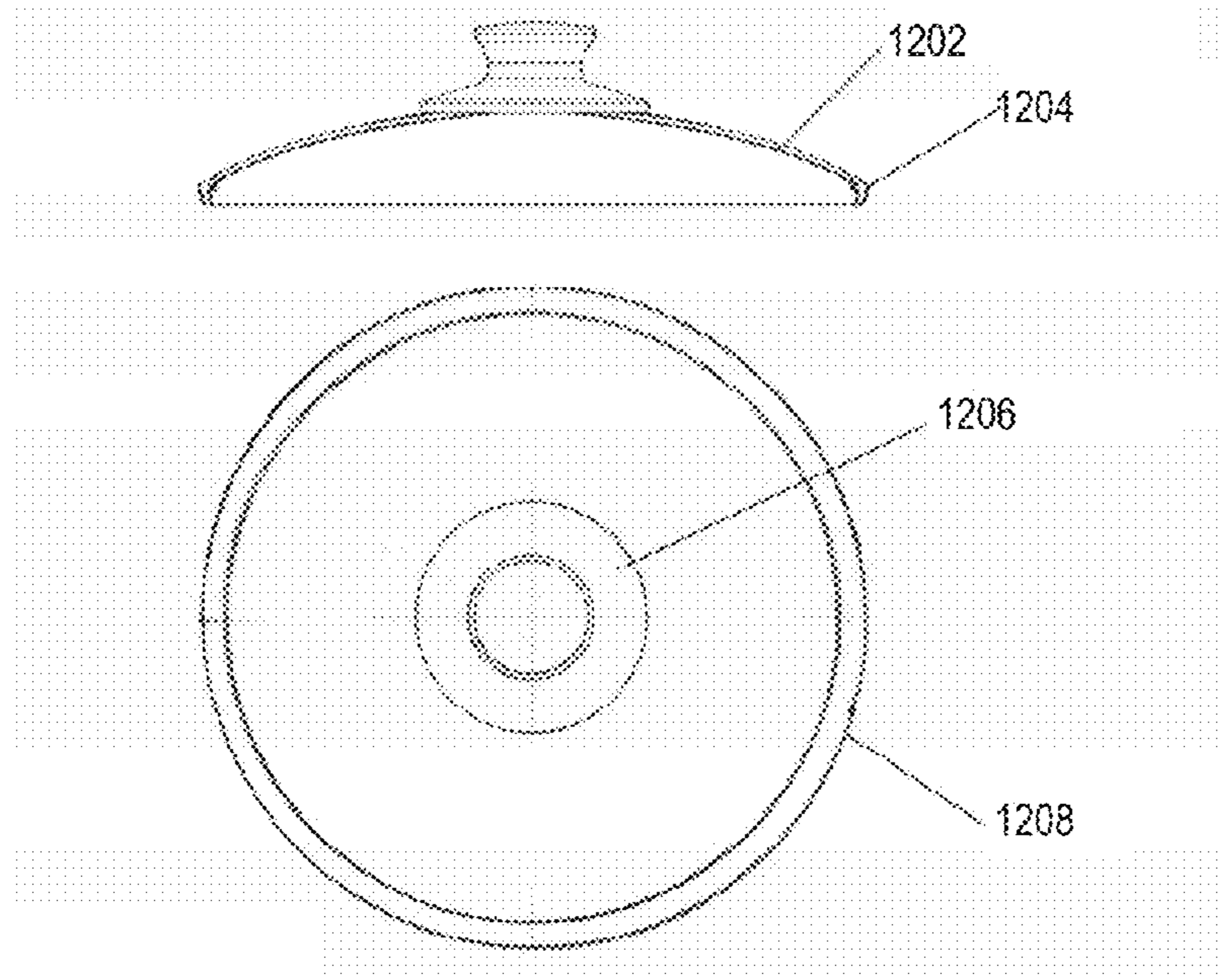
FIG. 12A
