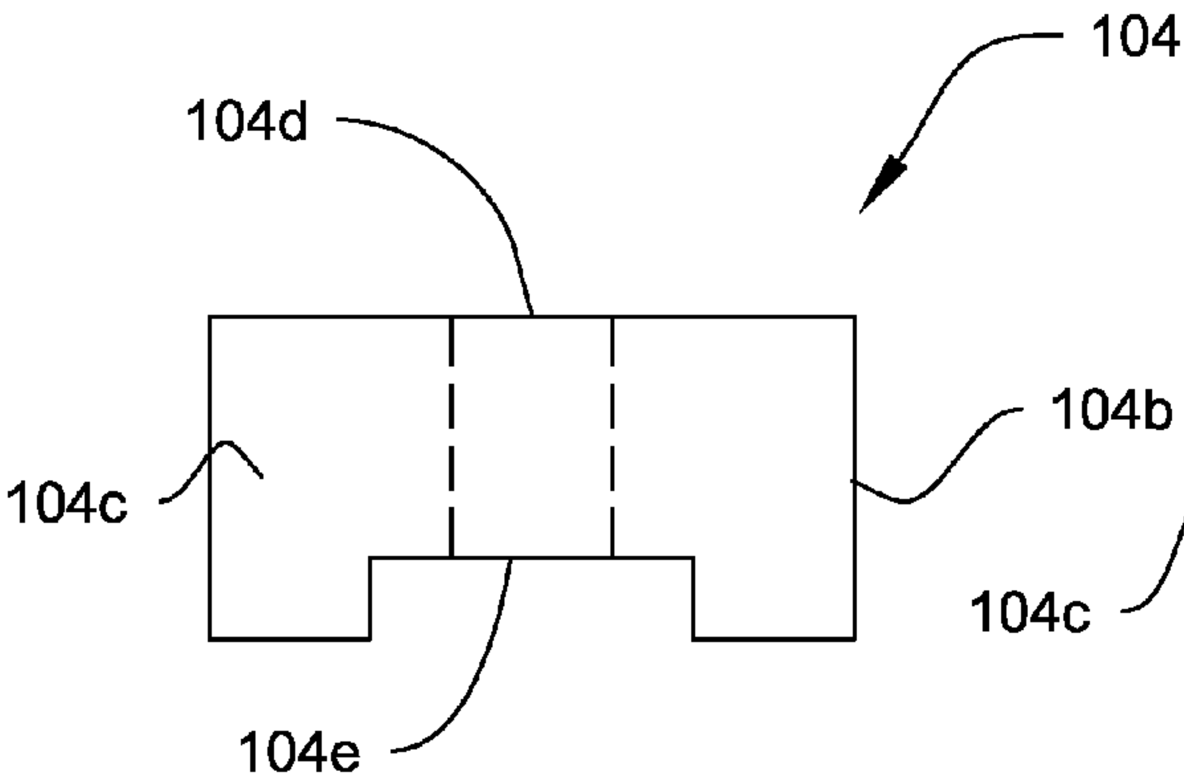
FIG. 7D
