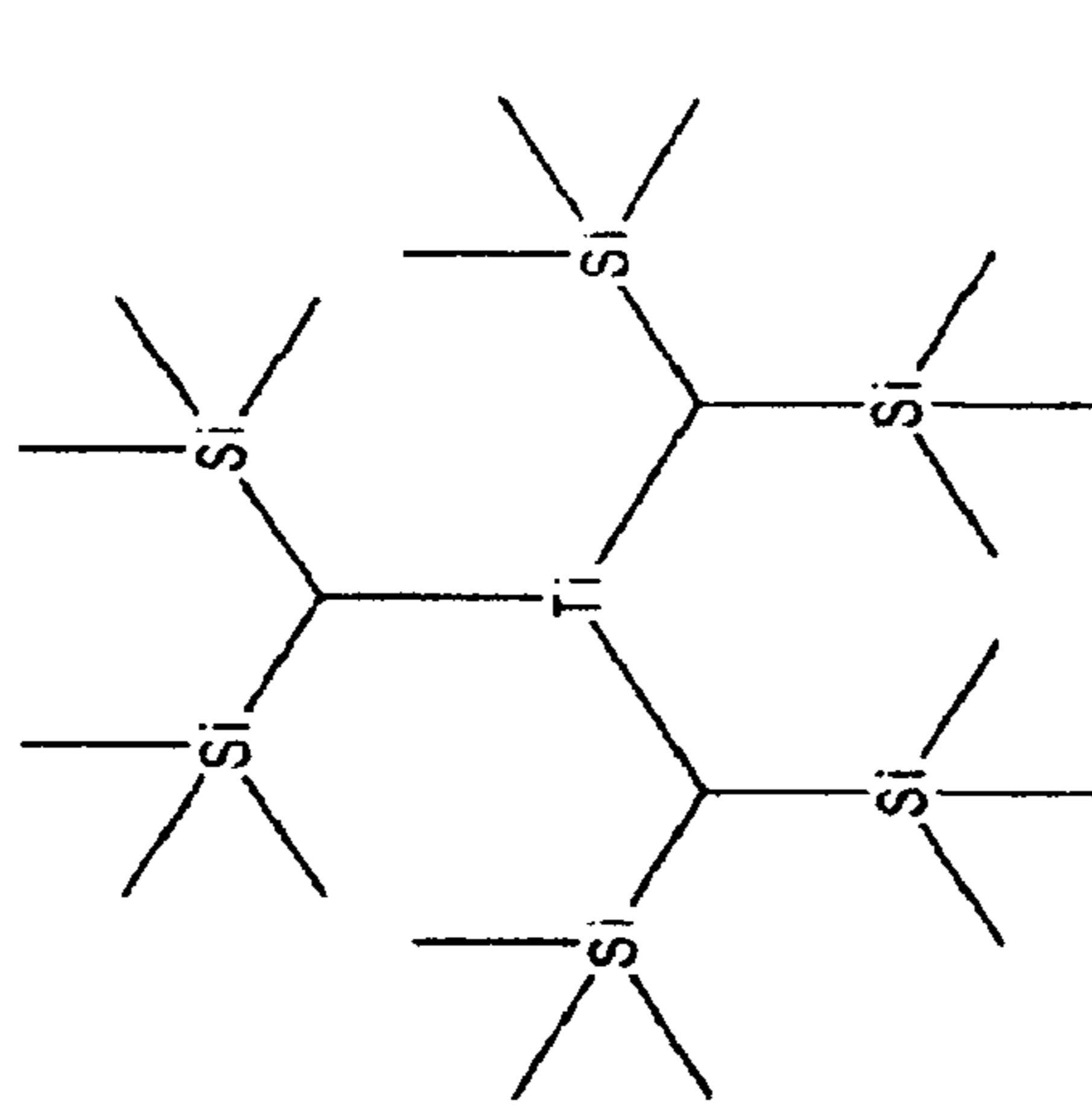
tris [bis(trimethylsilyl)methyl]Titanium
