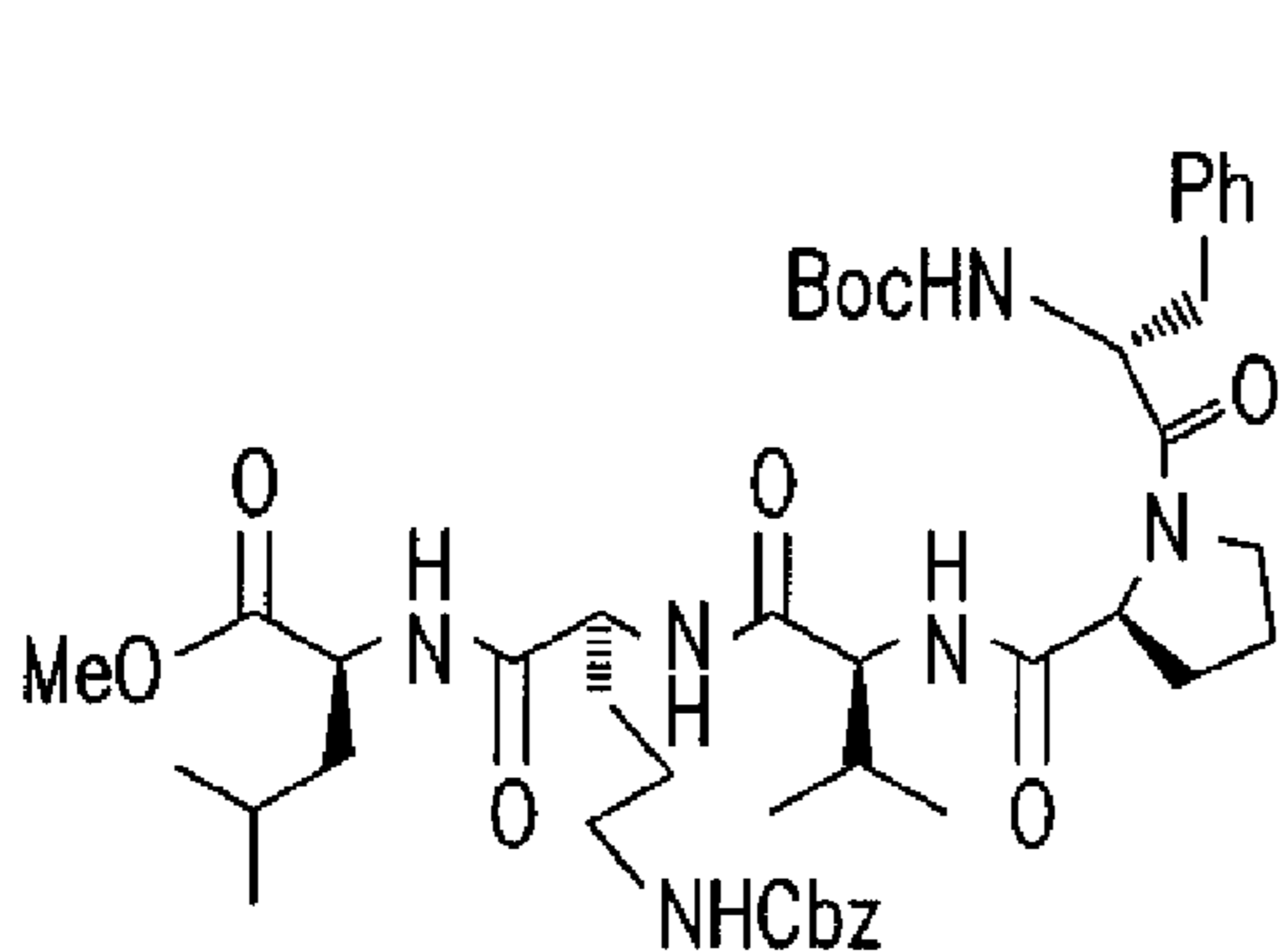
XJB-2-300
