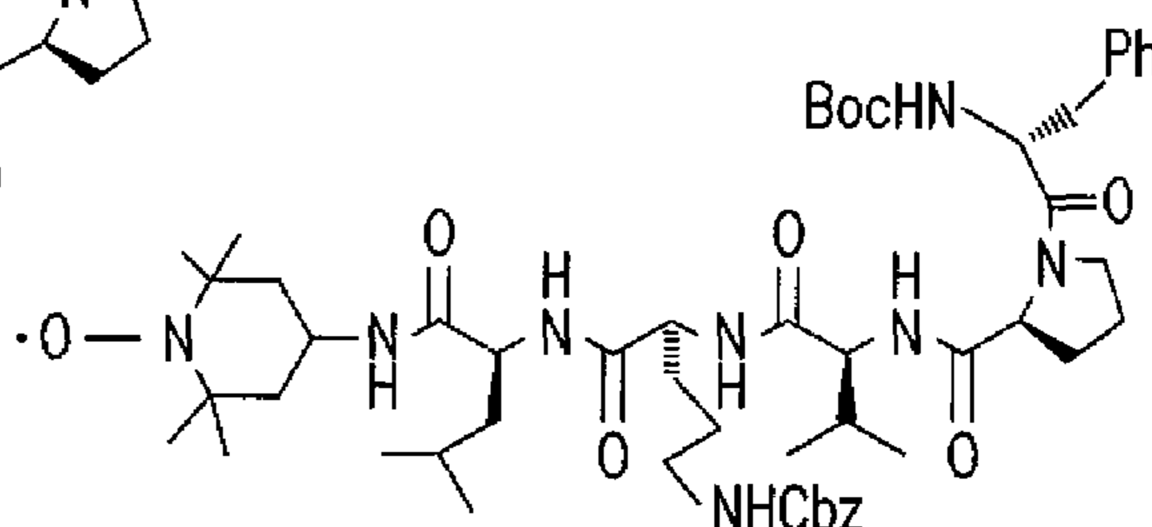
XJB-7-75
