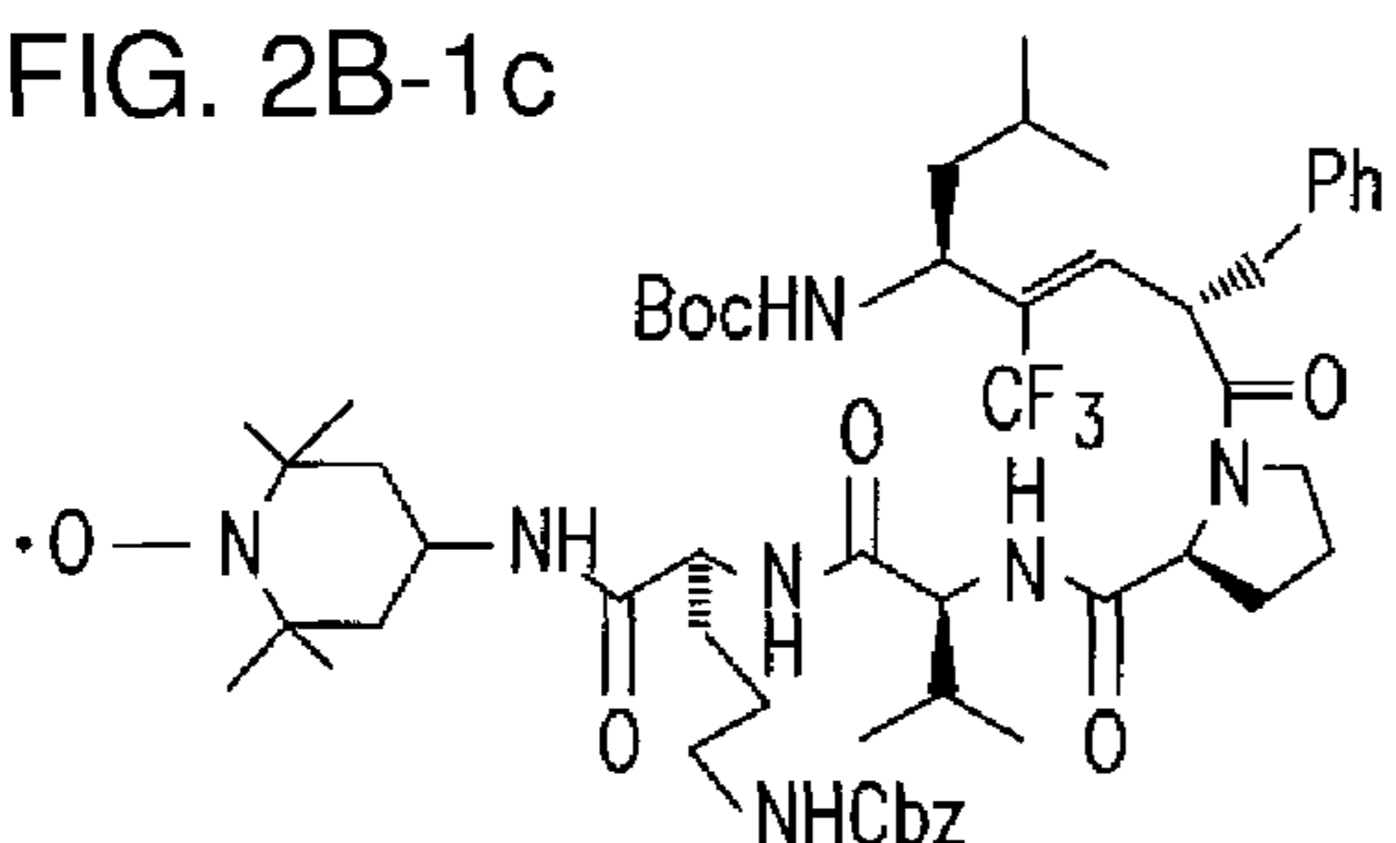
XJB-7-55
