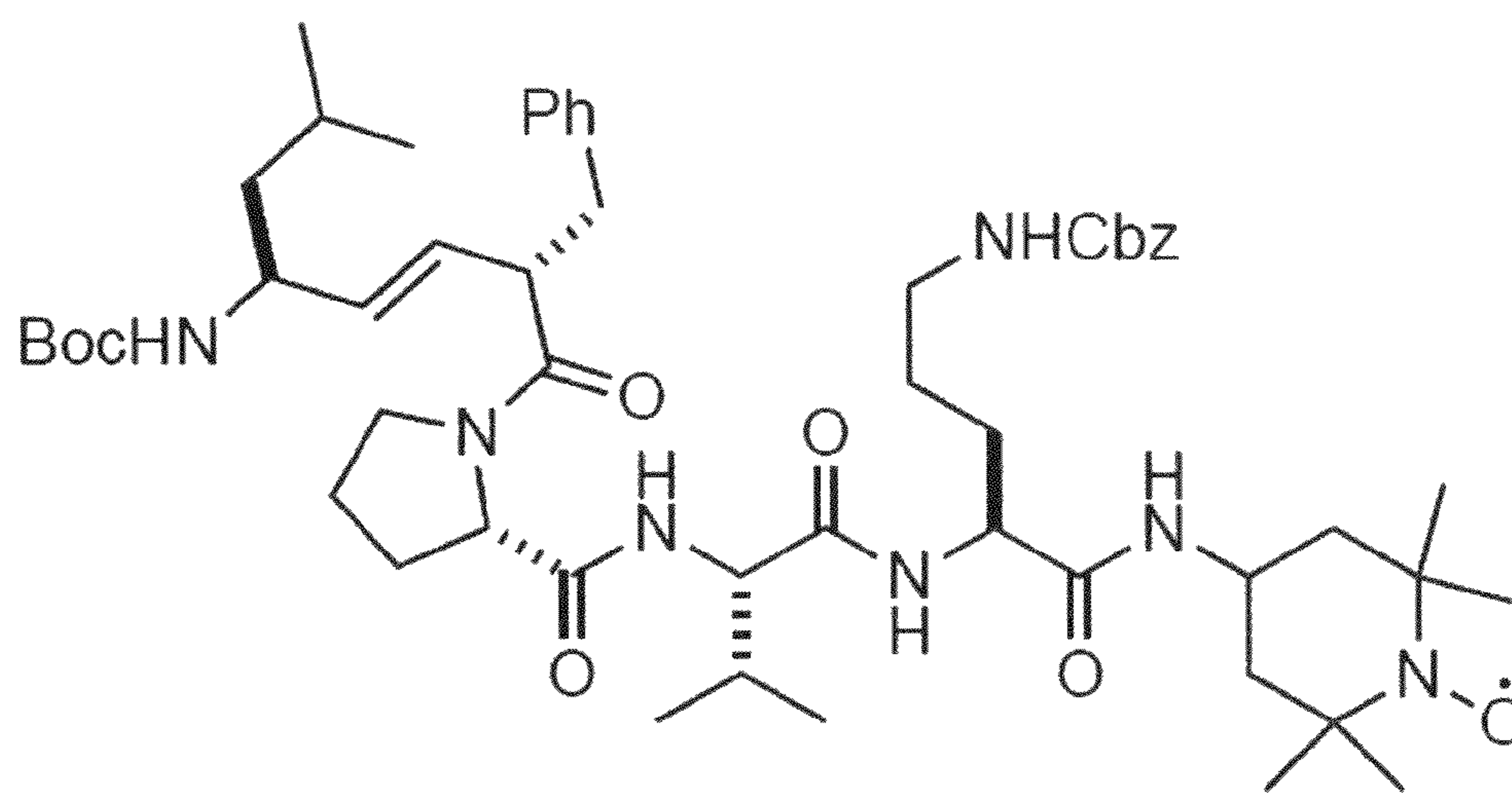
XJB-5-131
