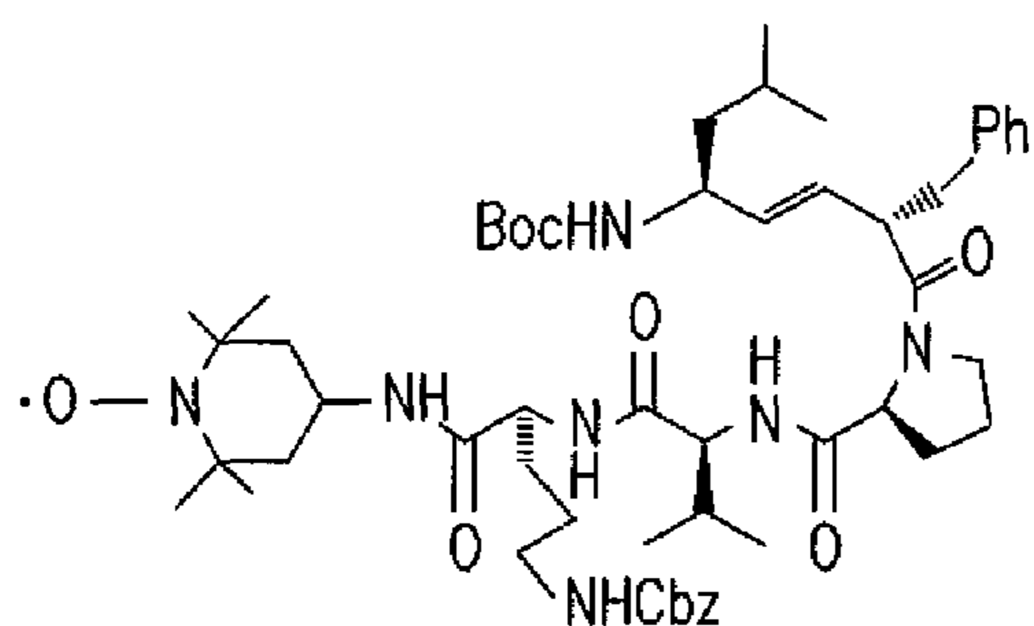
XJB-5-131
