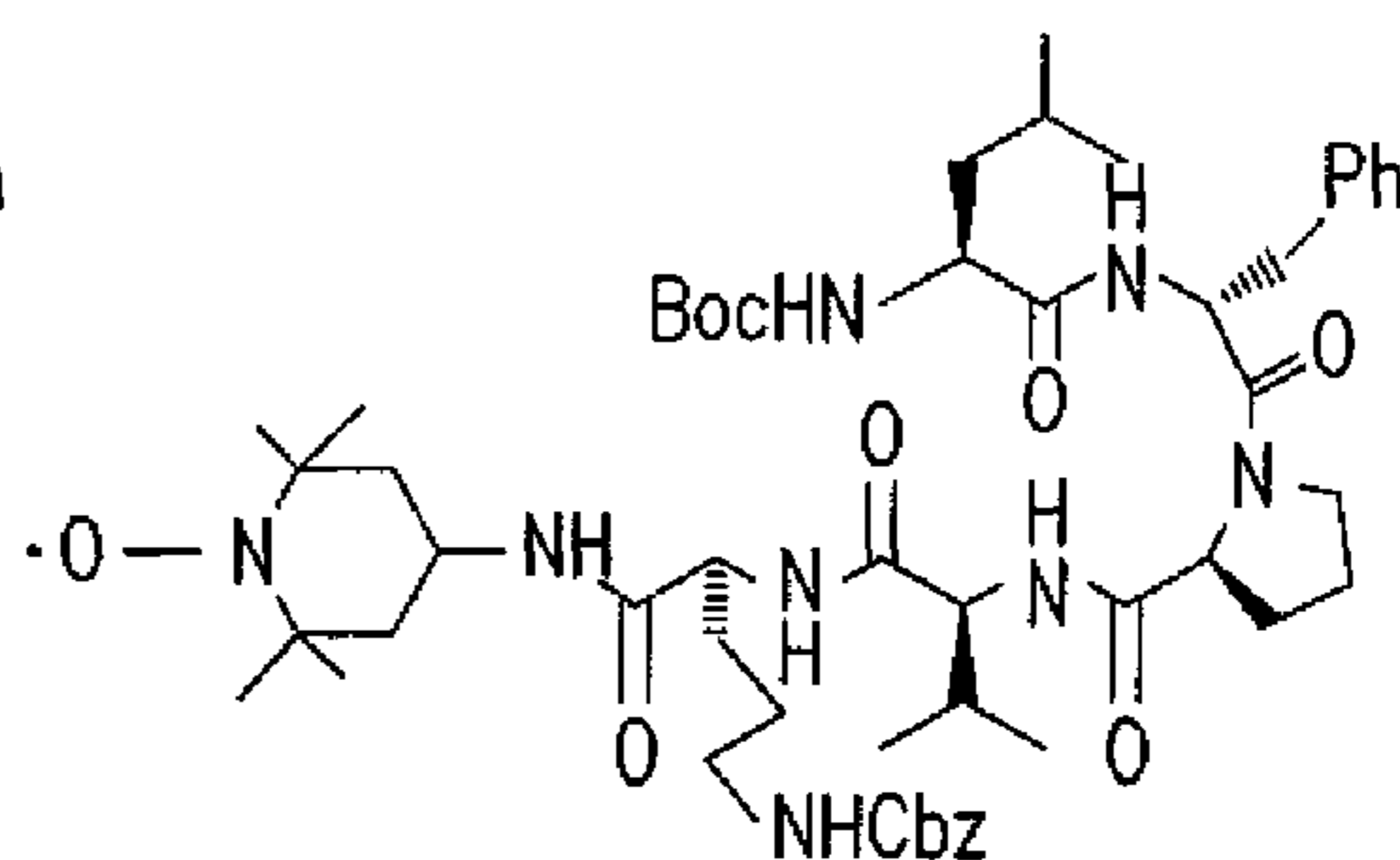
XJB-5-125
