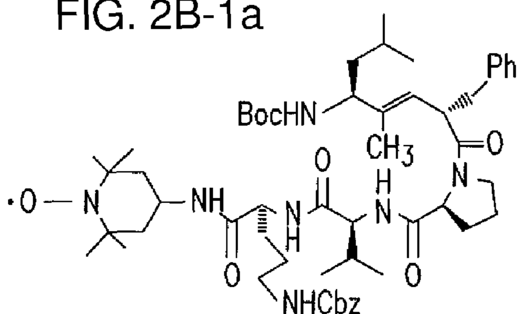
XJB-5-197
