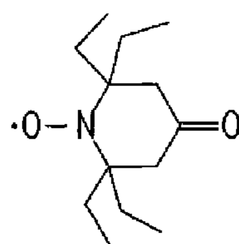
G6, LogP=3.2
