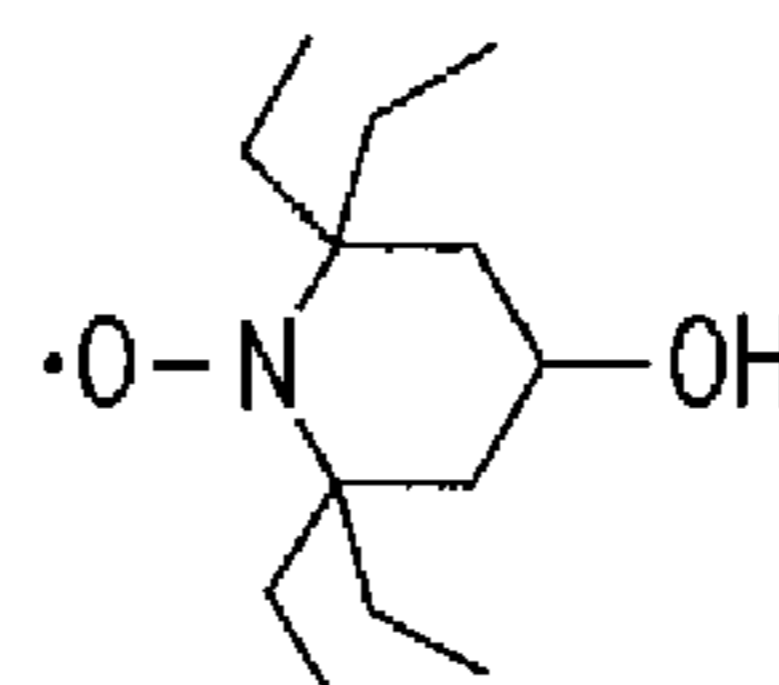
G3, LogP=3.4
