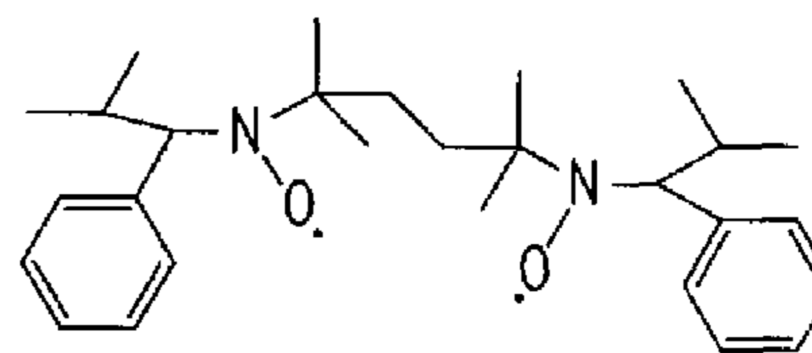
Bis-TIPNO, LogP=7.3
