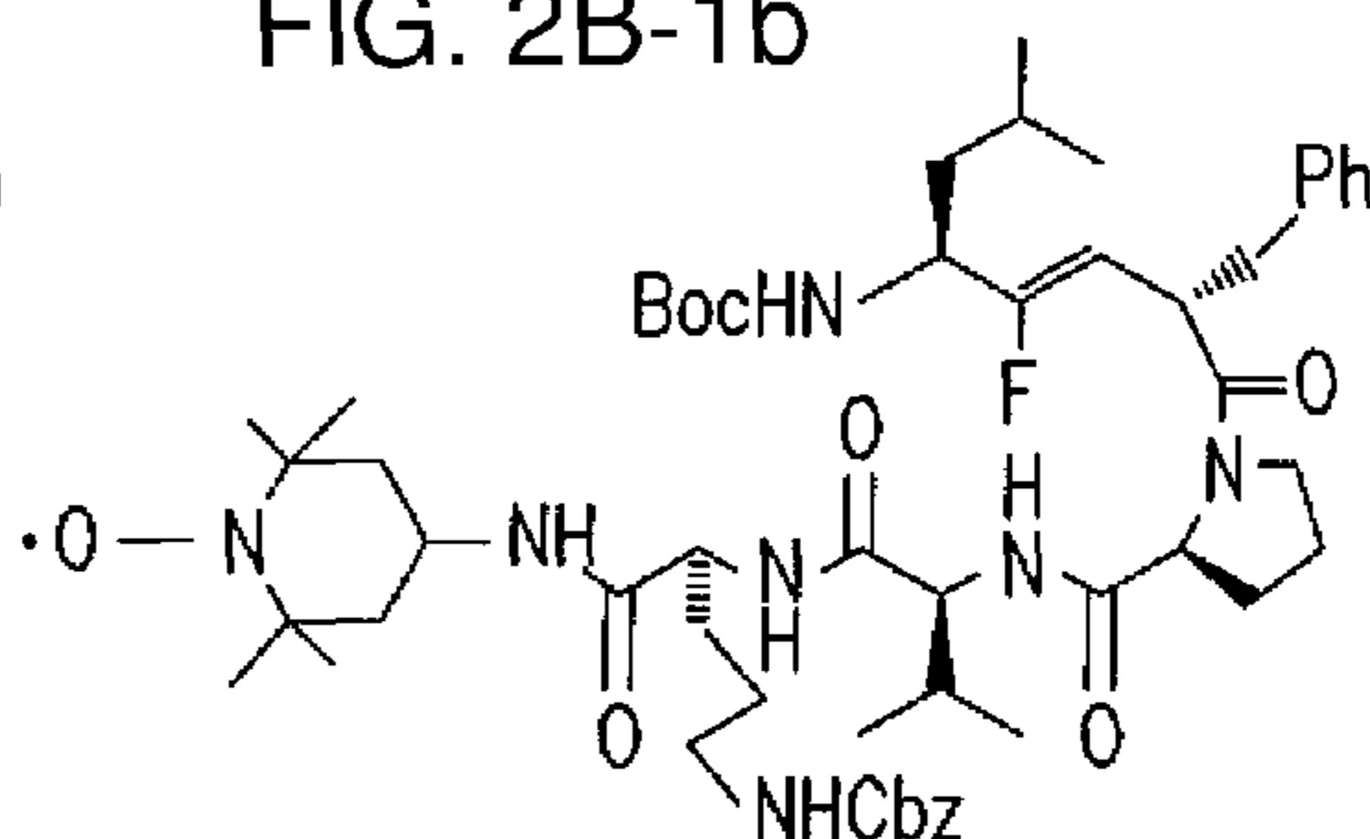
XJB-7-53
