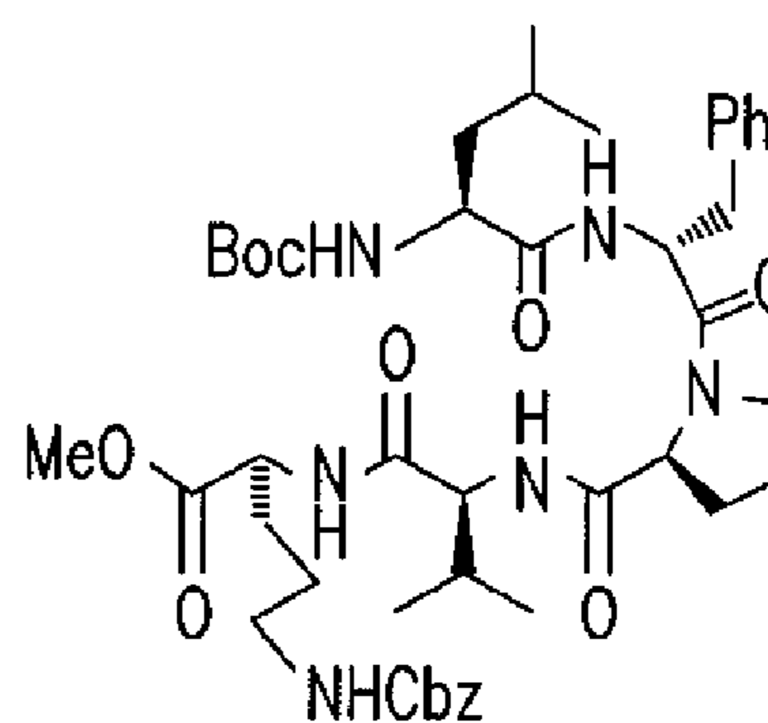
XJB-2-70
