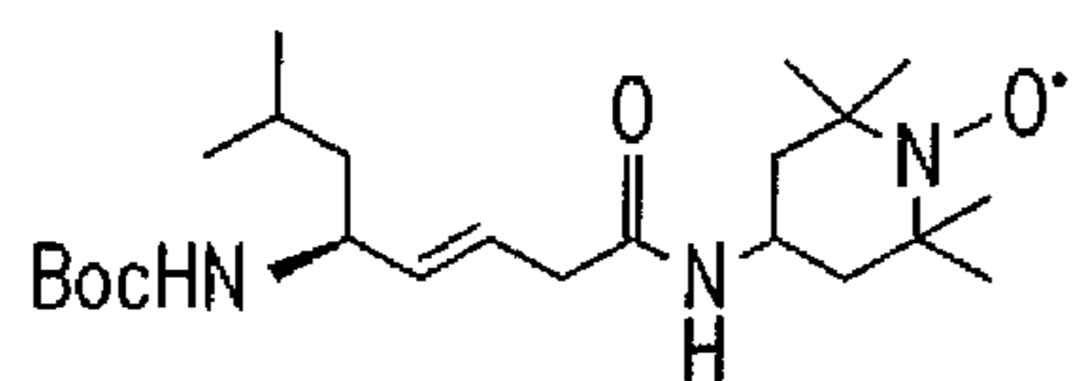
JP4-039
