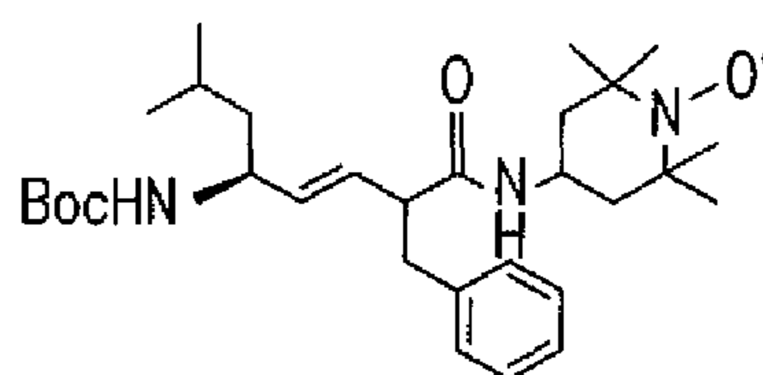
JP4-049
