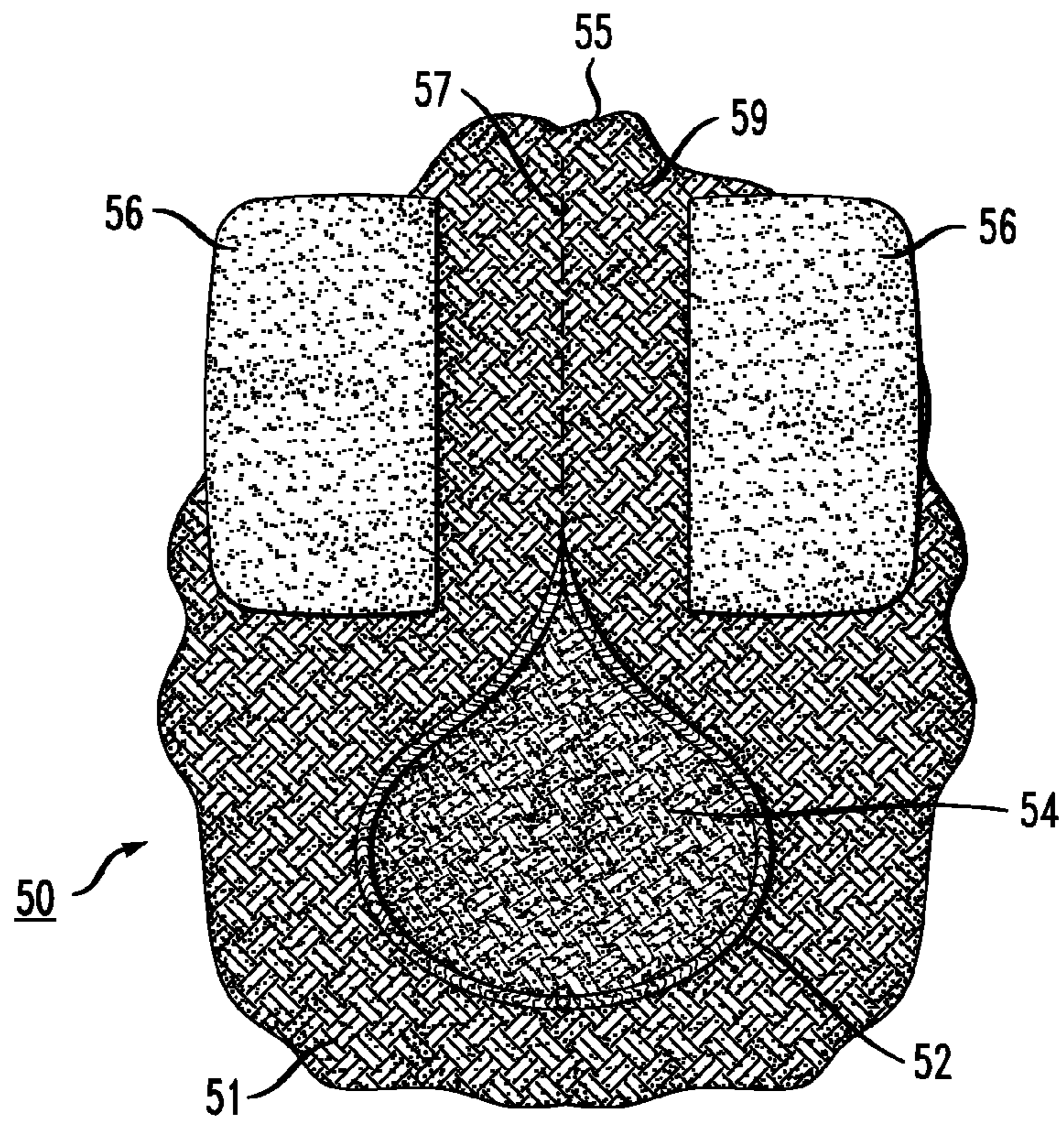
FIG. 5A
