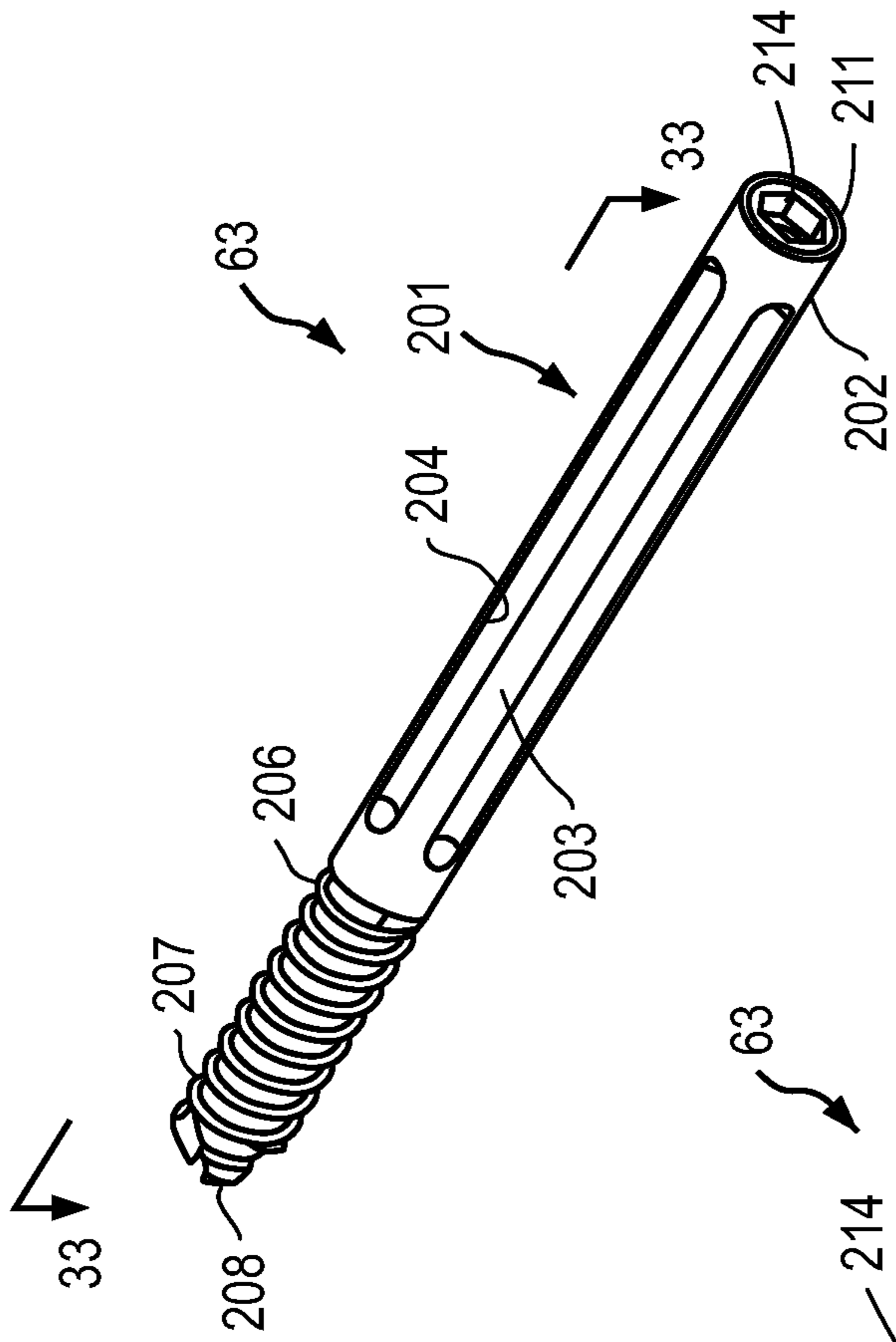
FIG. 32
