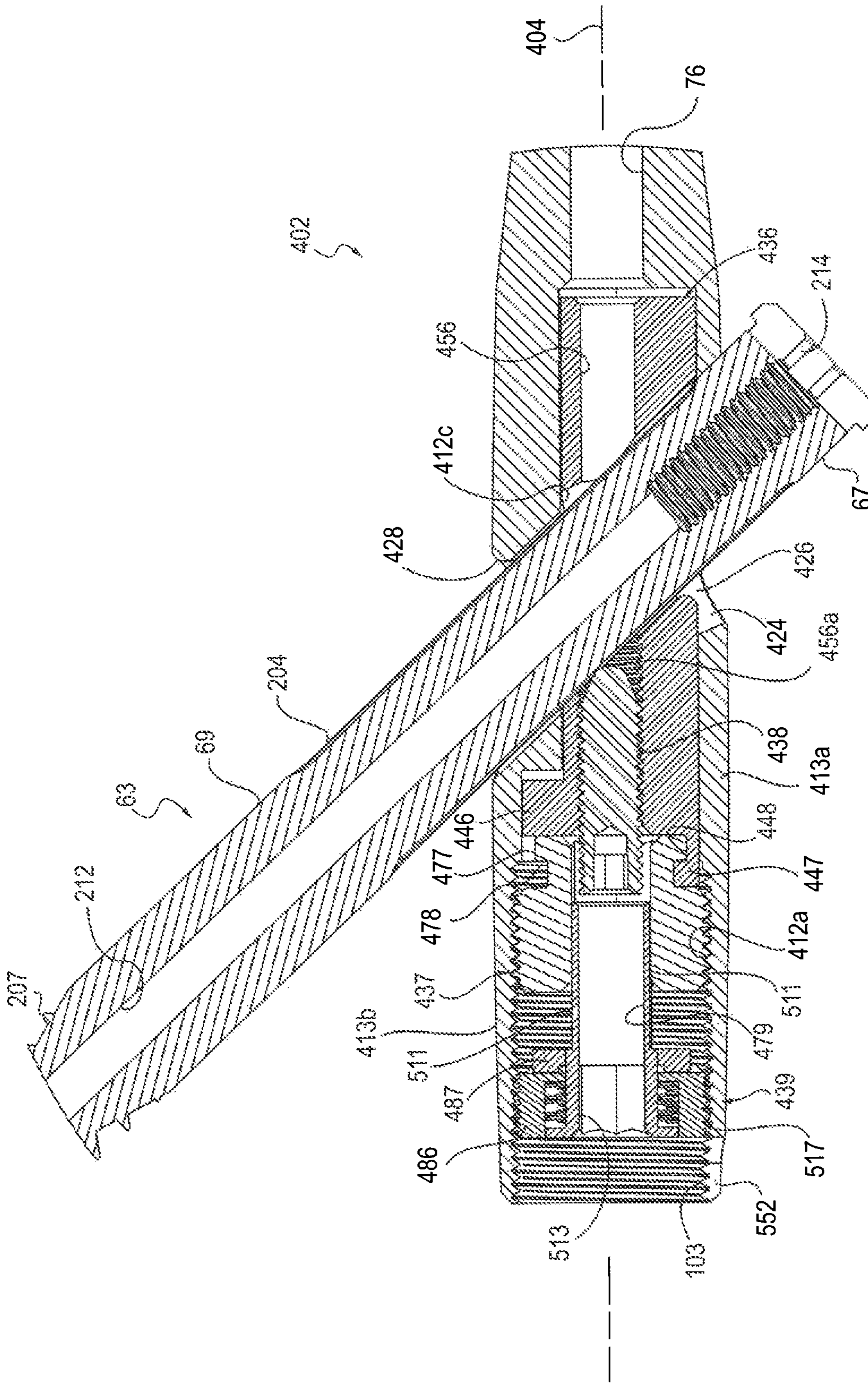
FIG. 81
