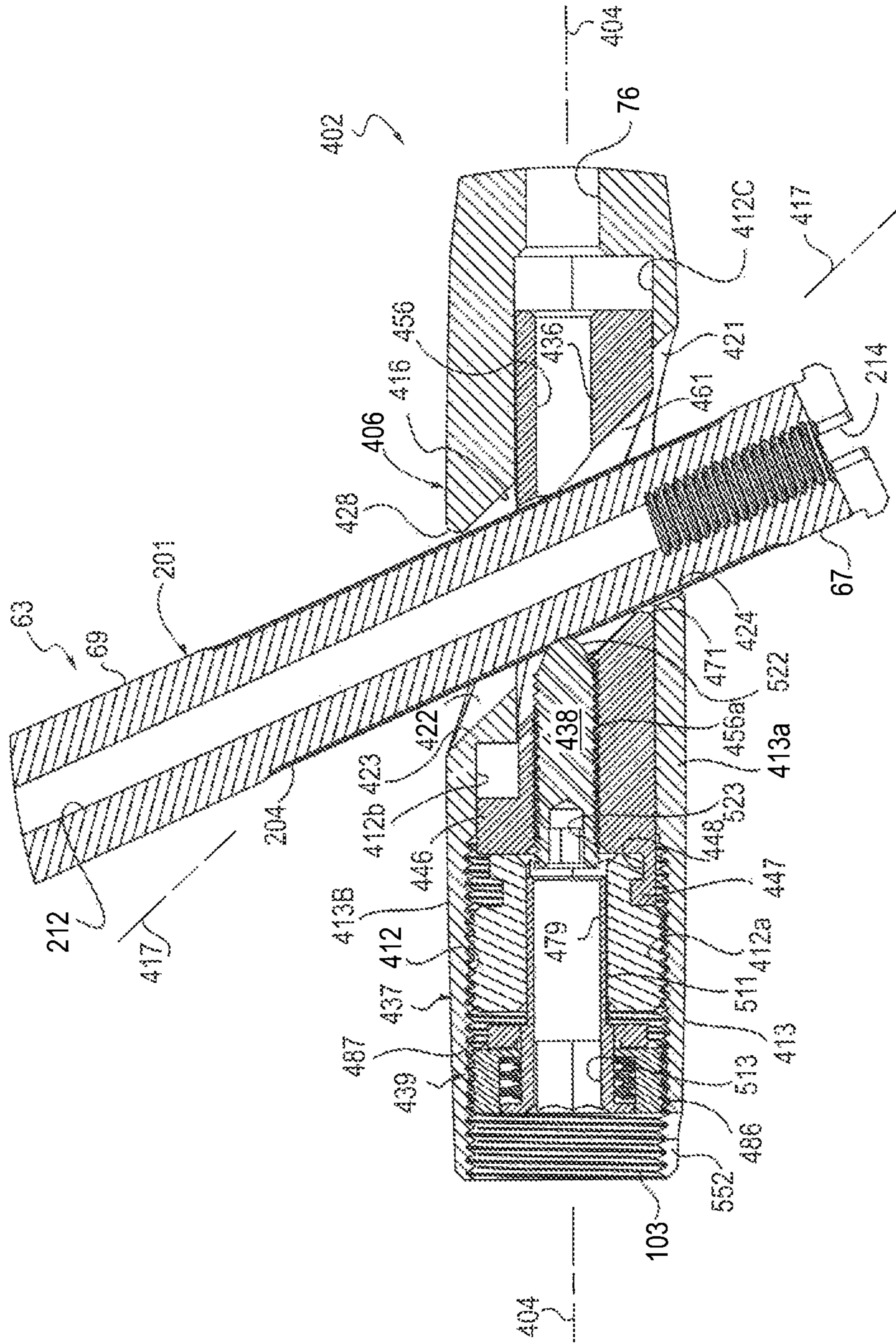
FIG. 68
