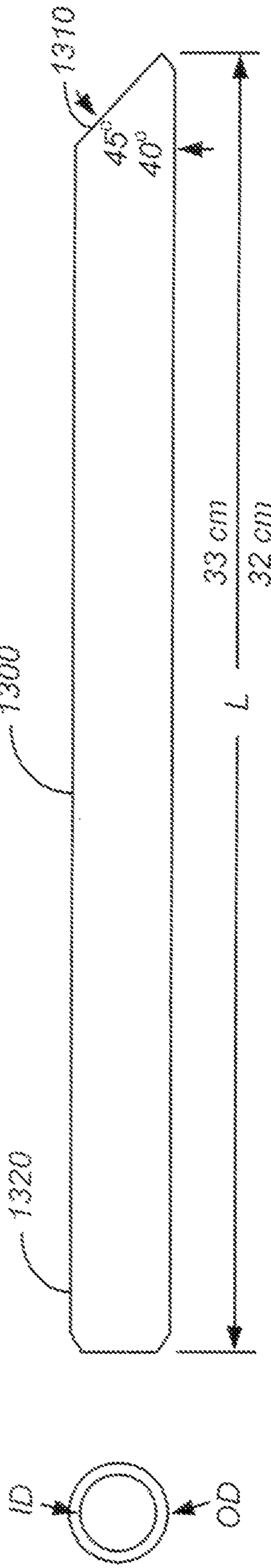
FIG. 13B
