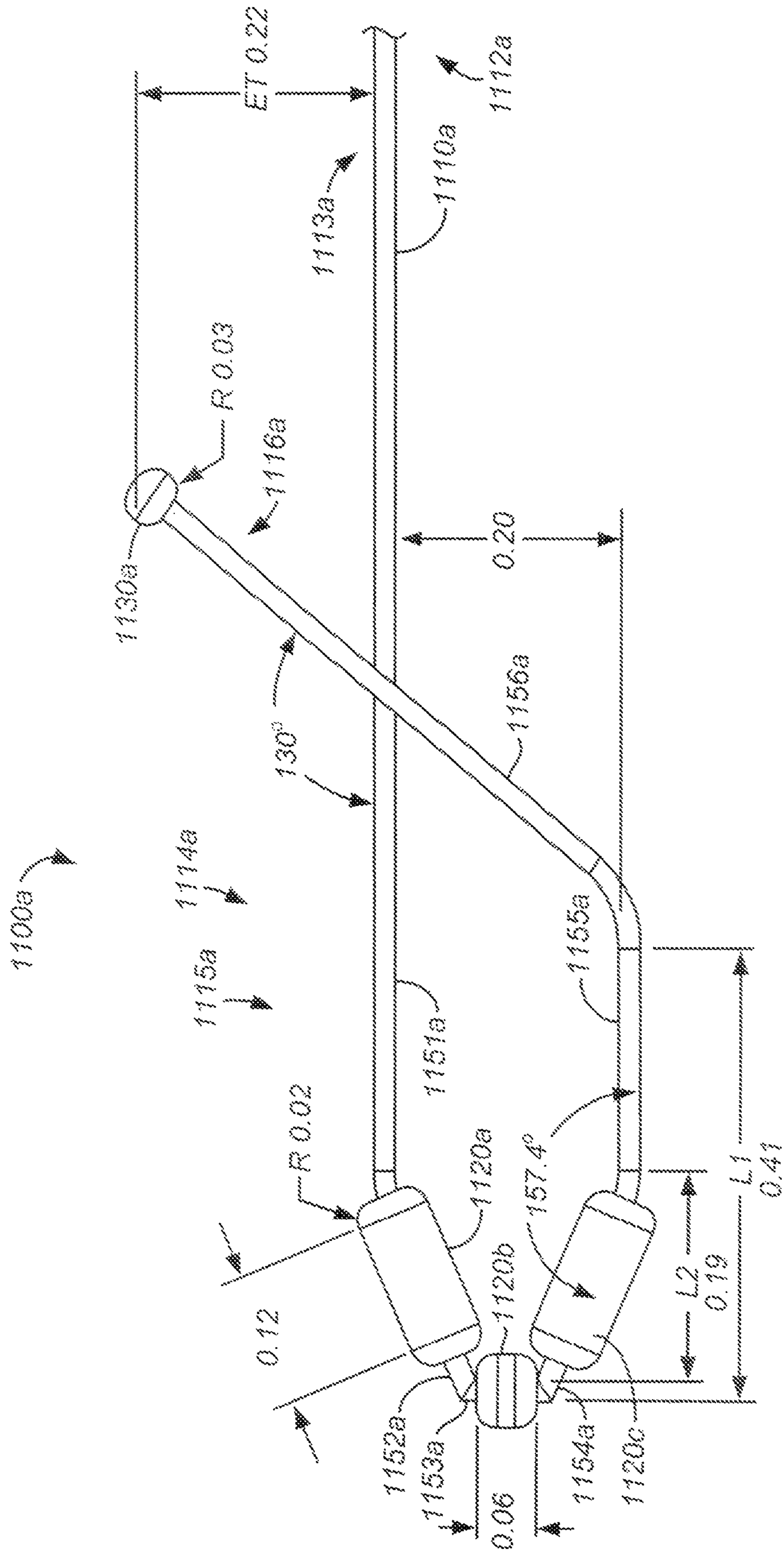
FIG. 11A
