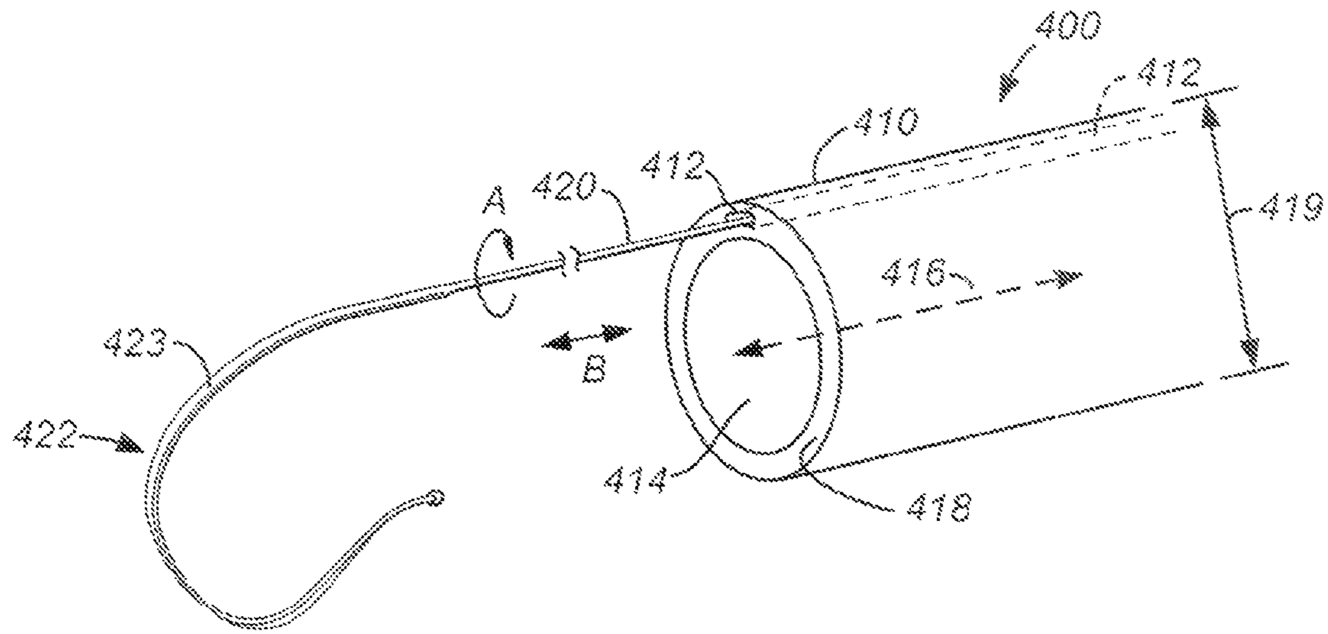
FIG. 4A
