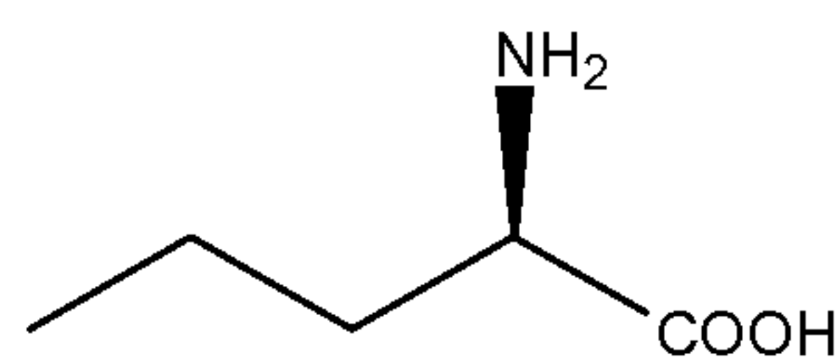
D-norvaline
