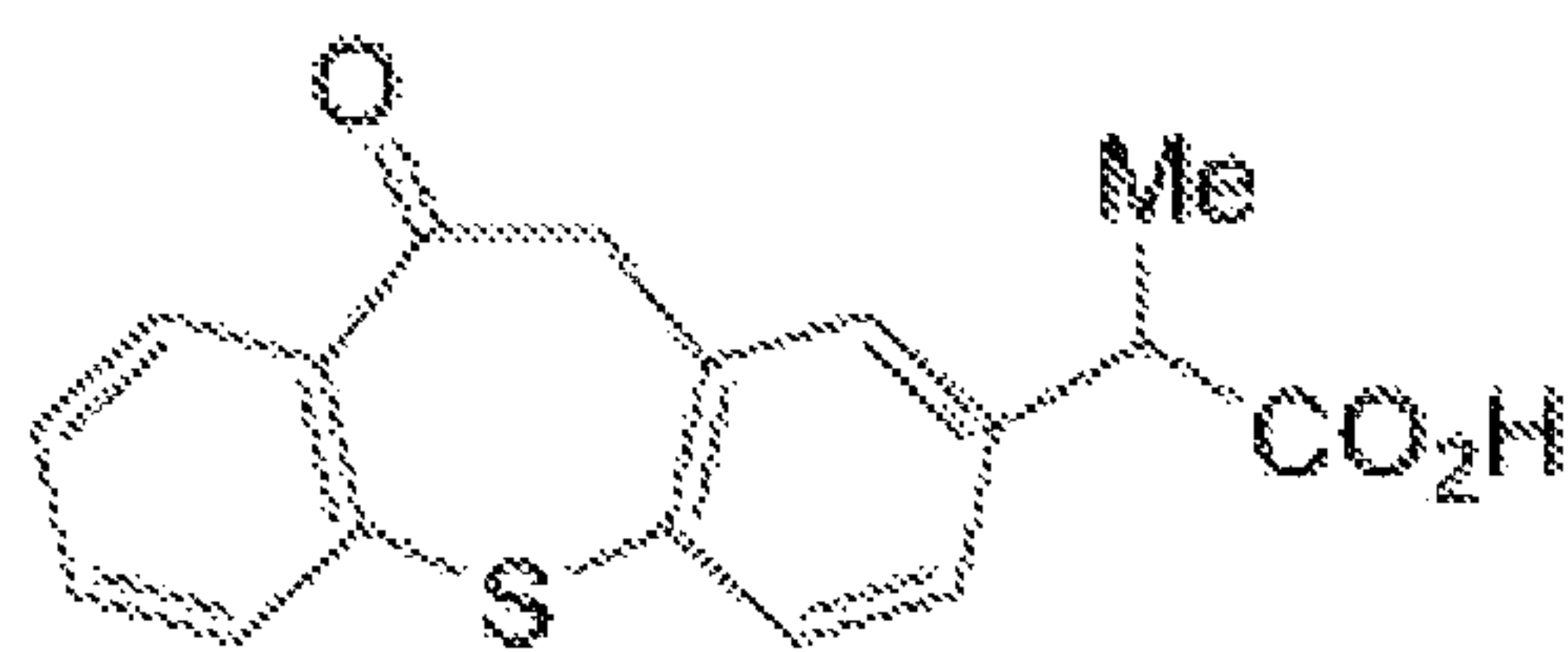
Zaltoprofen
