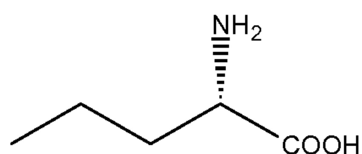
L-norvaline
