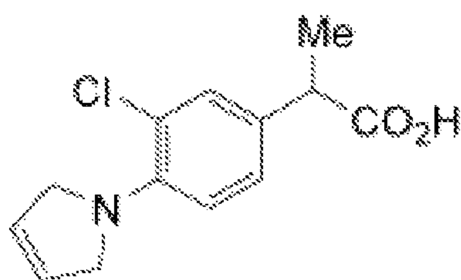
Pirprofen
