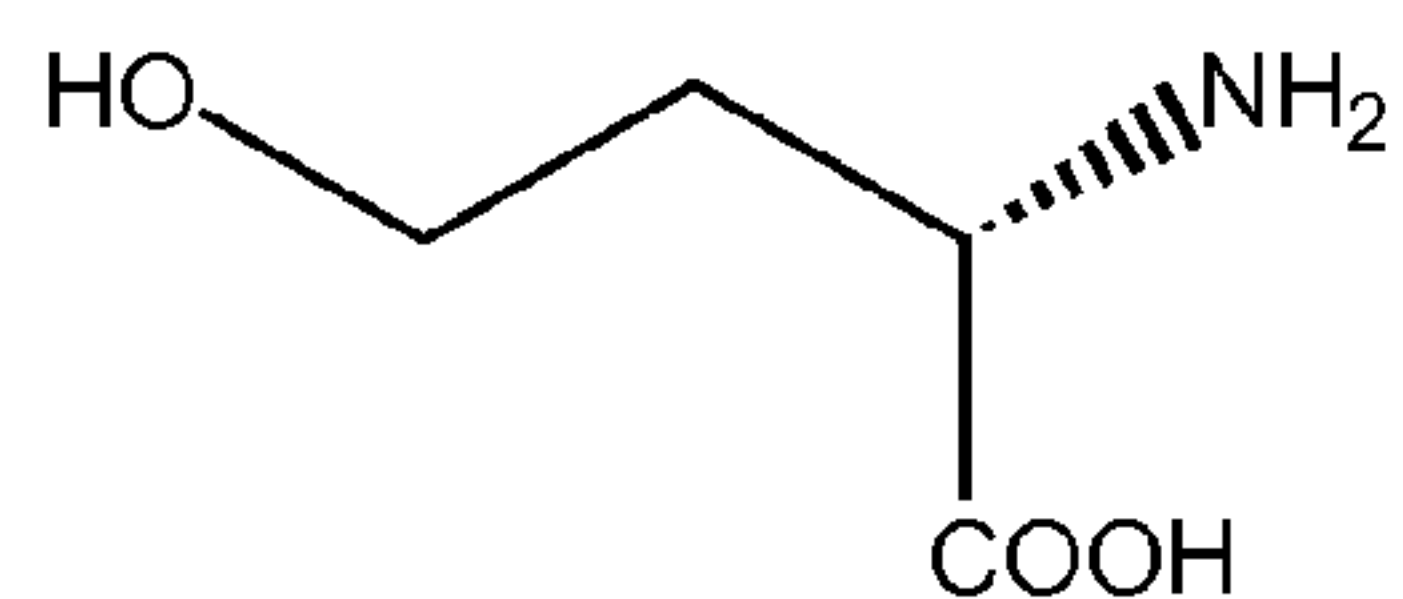
L-homoserine
