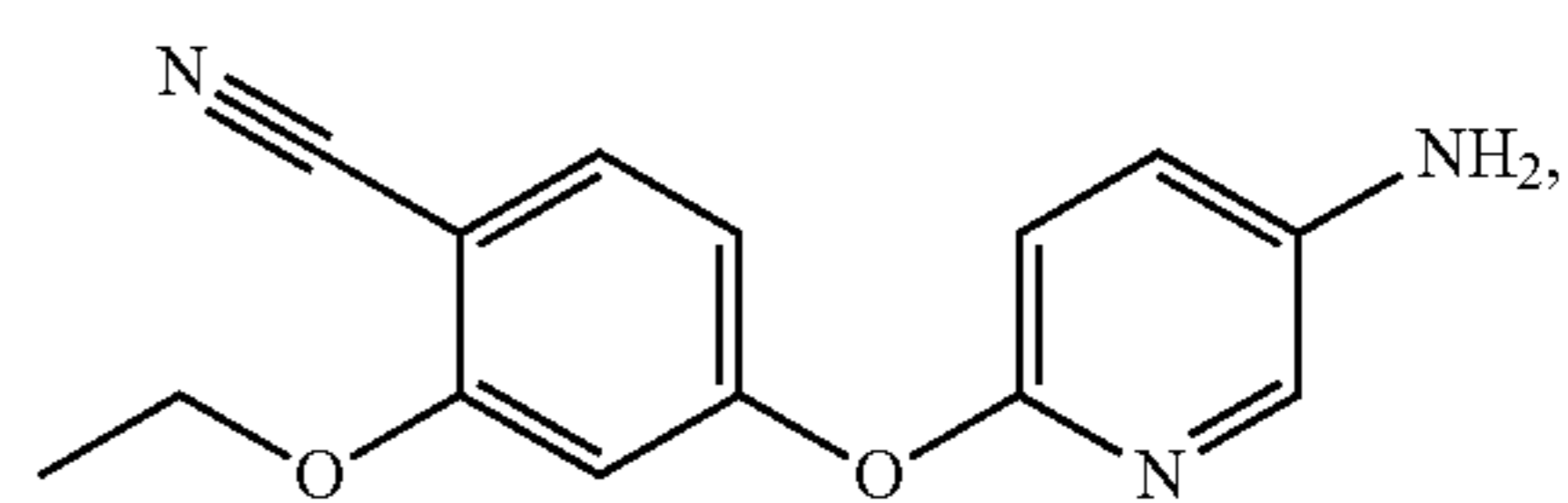
4-[[5-amino-2-pyridinyl]oxy]-2-(ethoxy)benzonitrile
