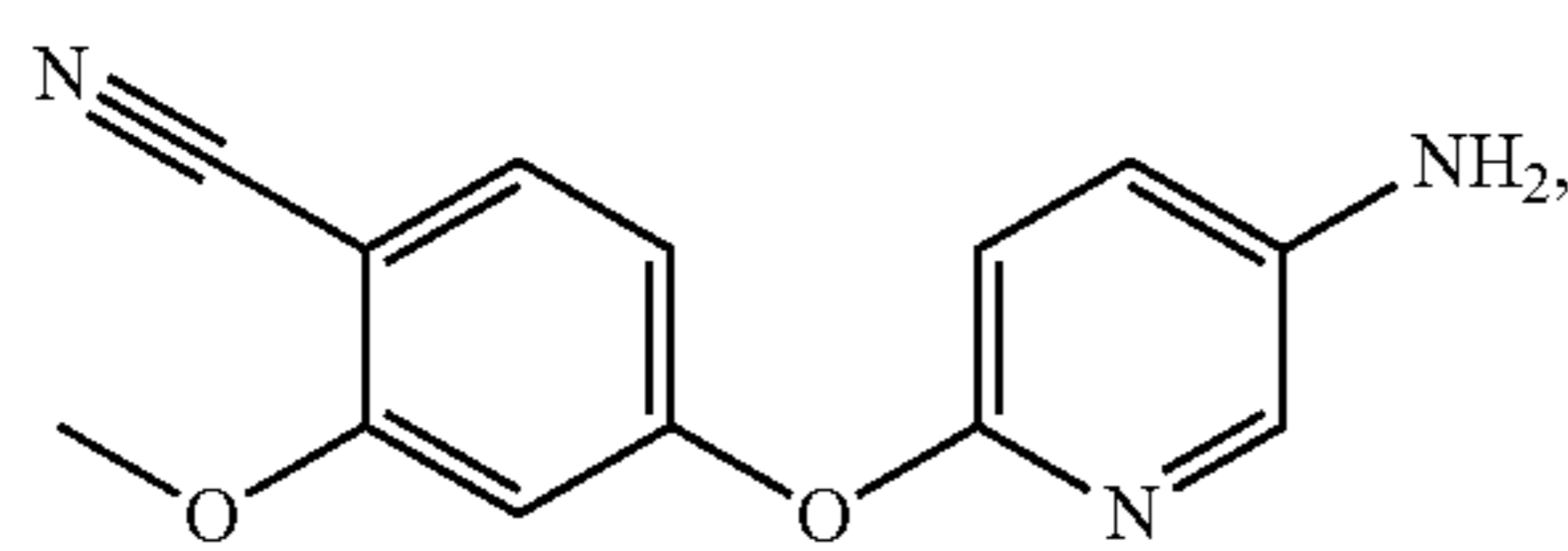
4-[[5-amino-2-pyridinyl]oxy]-2-(methoxy)benzonitrile
