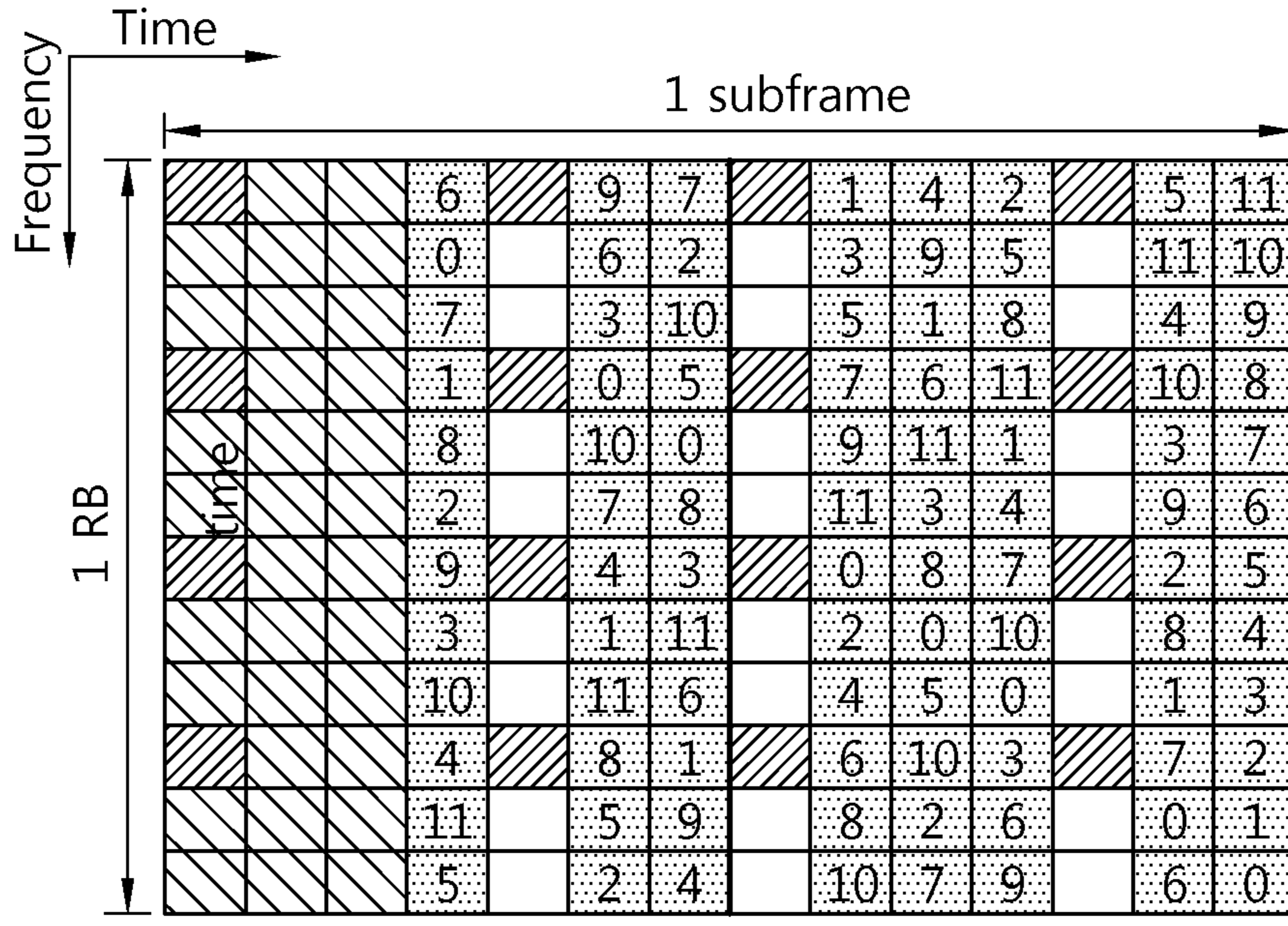
Normal subframe
