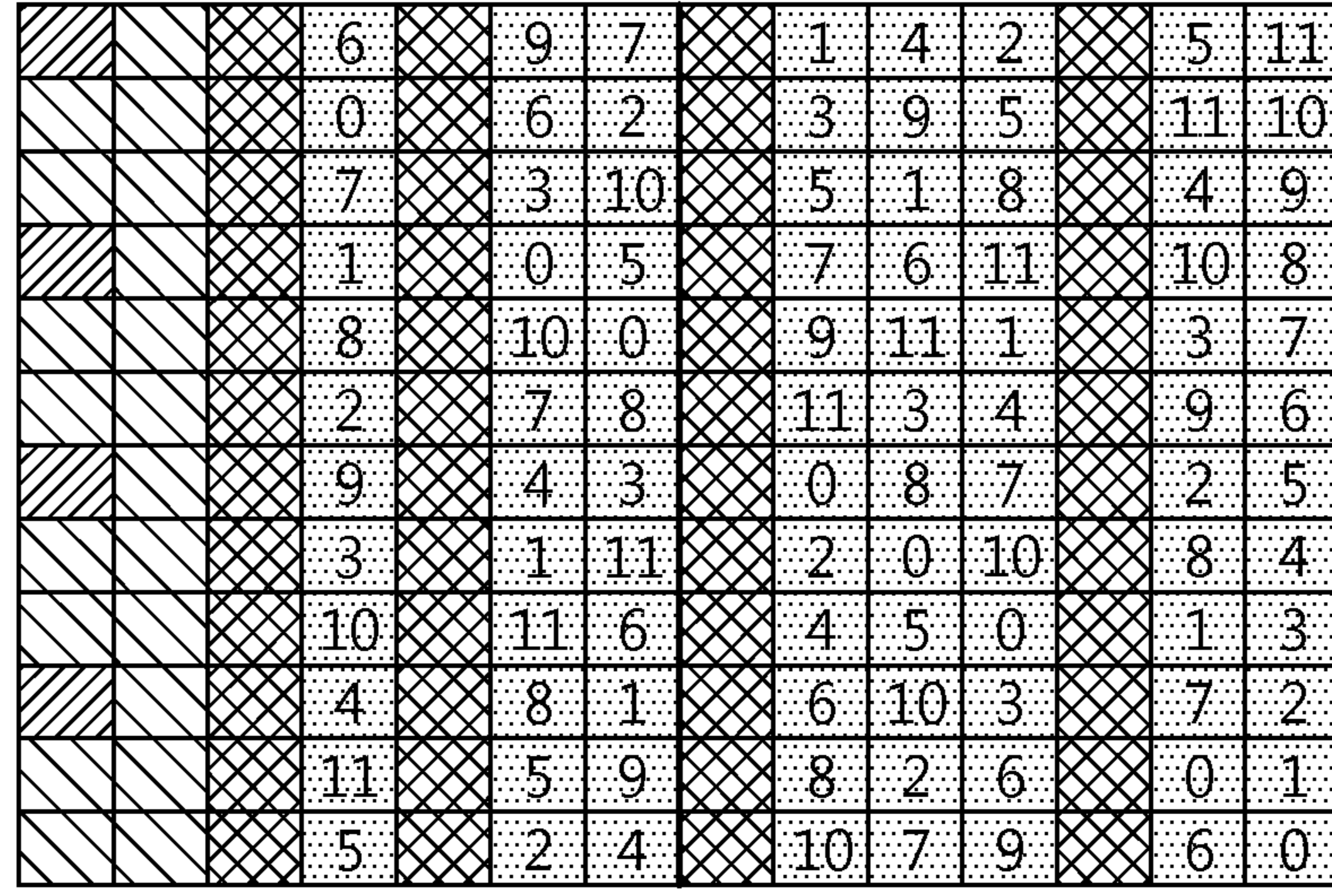
MBSFN subframe
