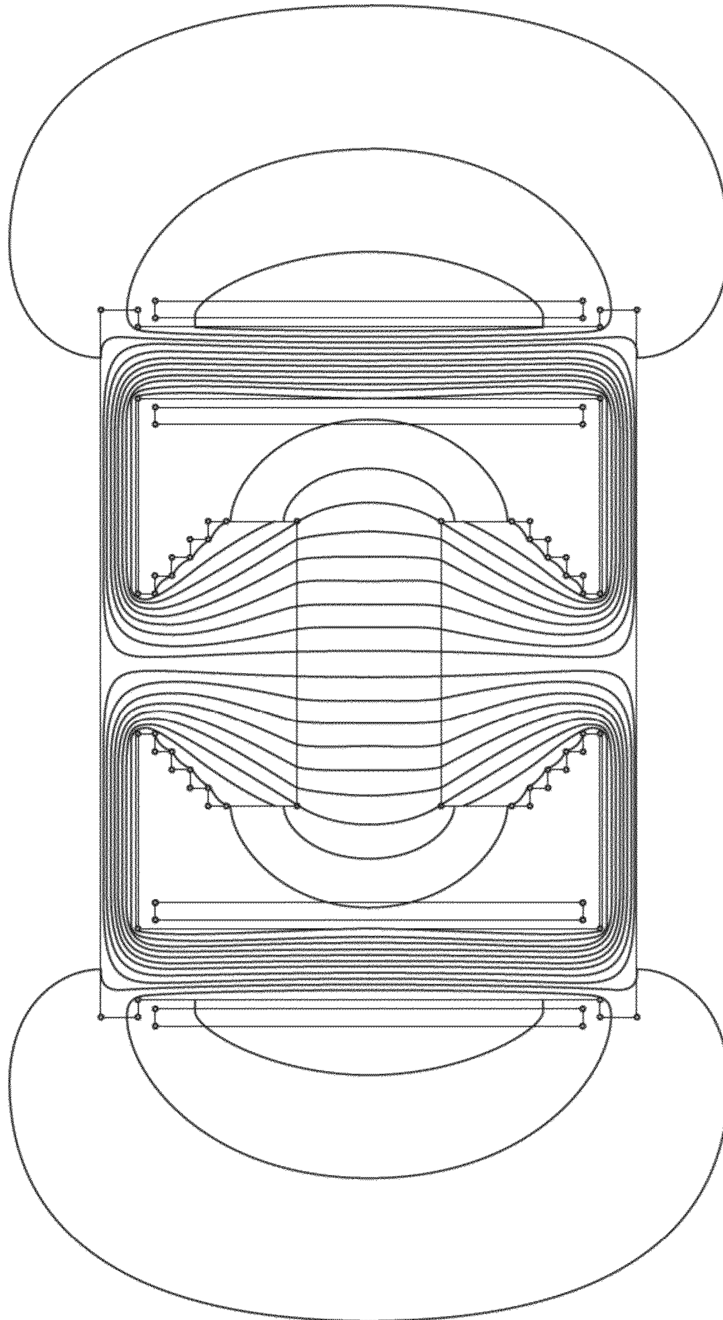
FIG. 4
