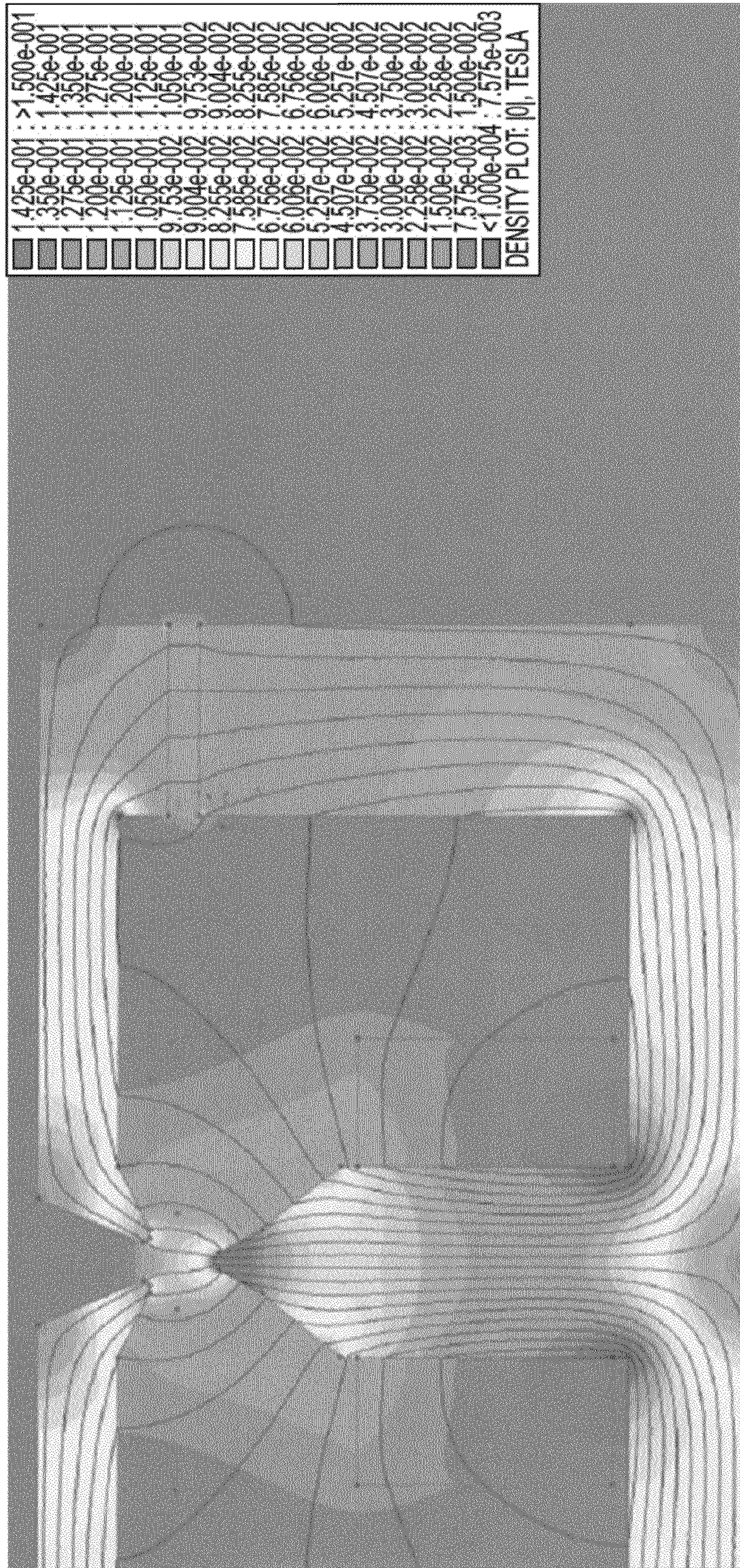
FIG. 11
