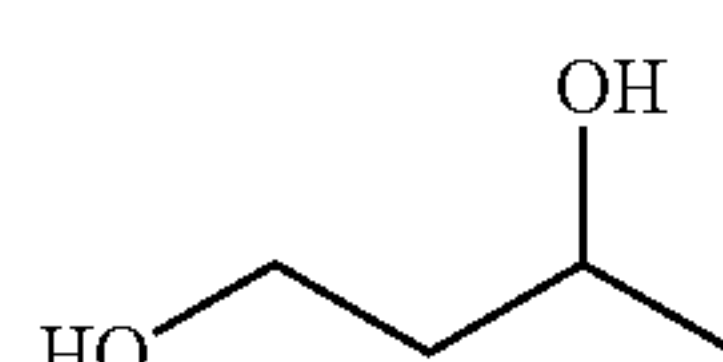
1,3-Butanediol
