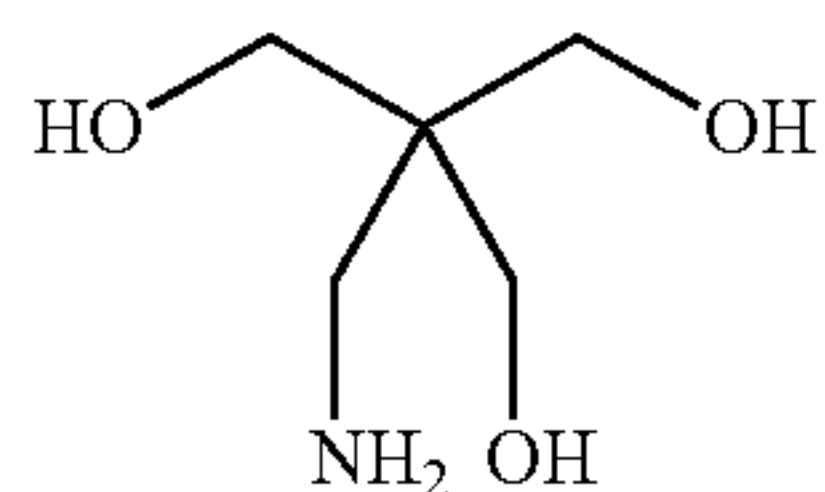
2-Amino-2-(hydroxymethyl)-1,3-propanediol
