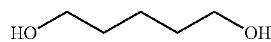
1,5-Pentanediol
