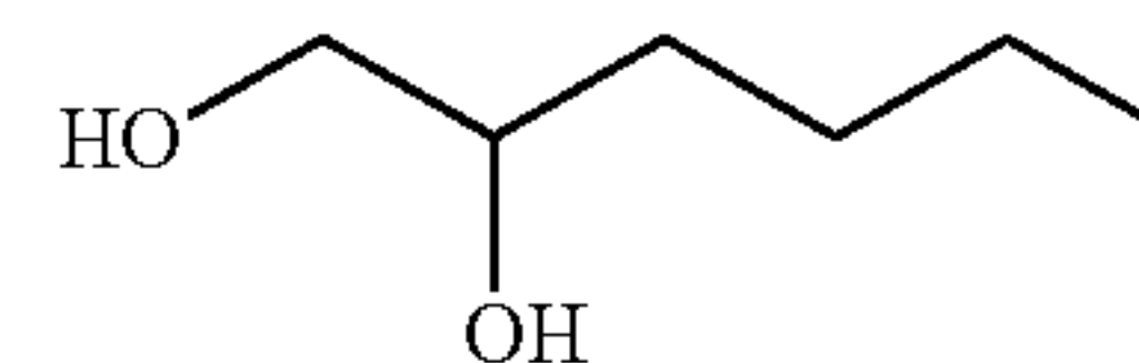
1,2-Hexanediol
