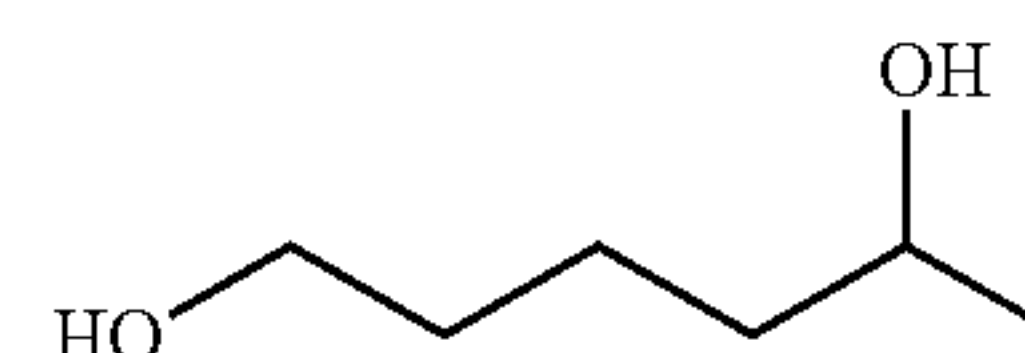
1,5-Hexanediol
