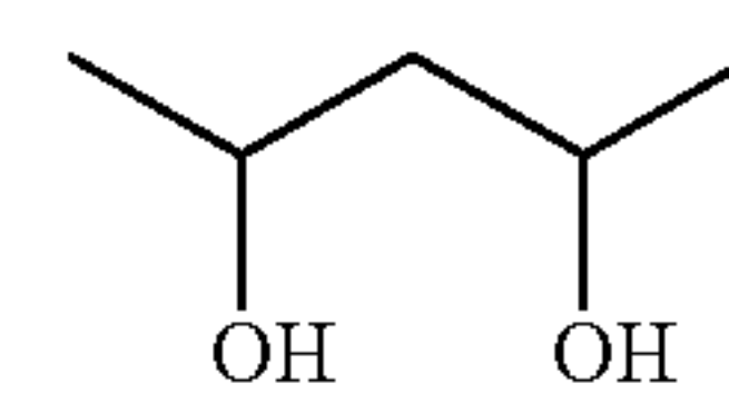
2,4-Pentanediol
