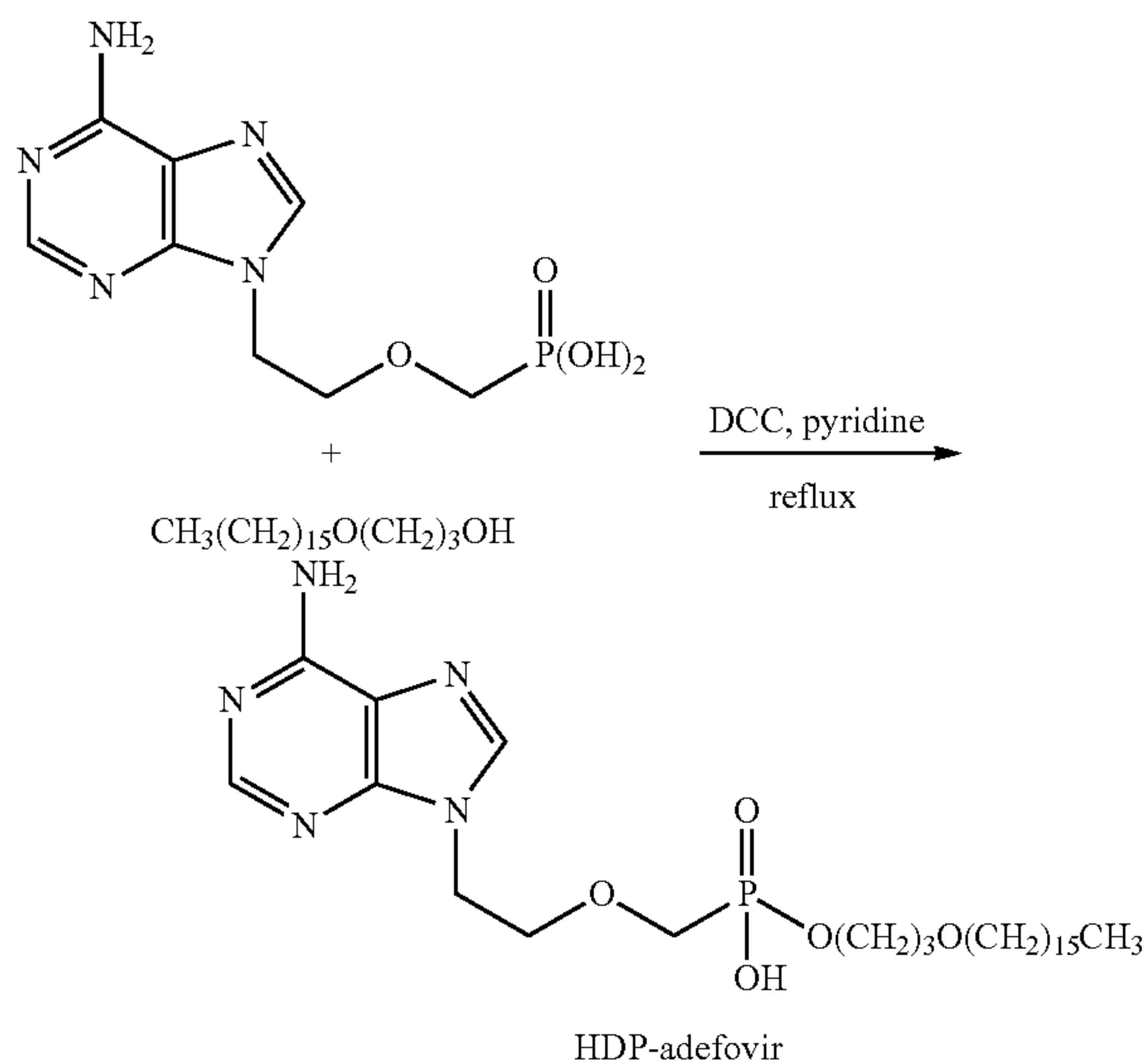
Scheme VI
