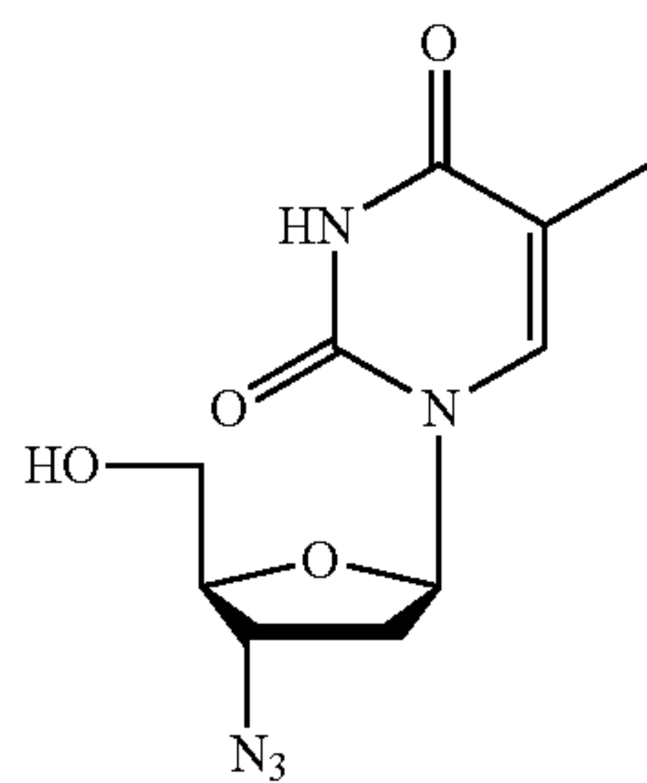
AZT
