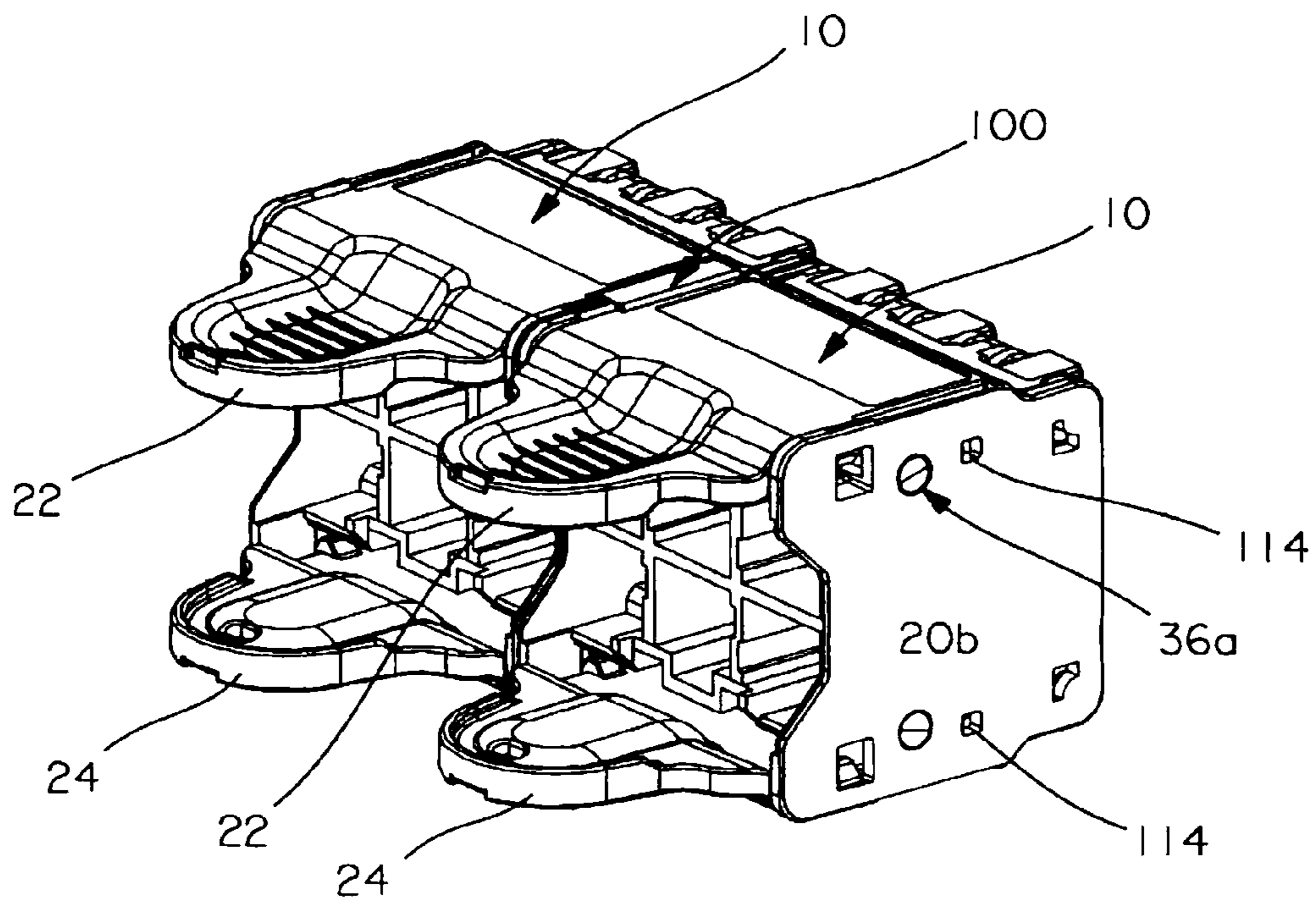
FIG. 23
