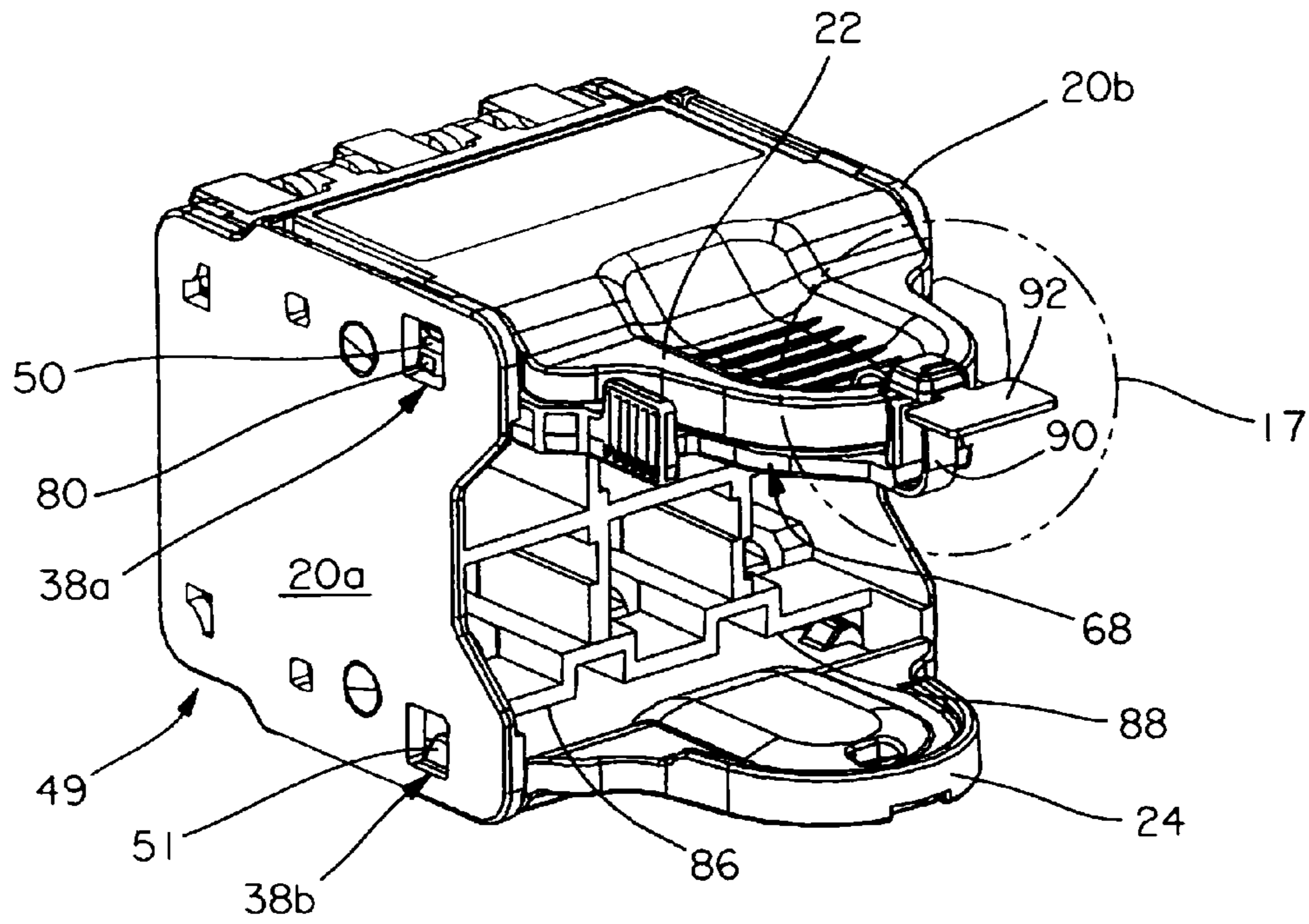
FIG. 16
