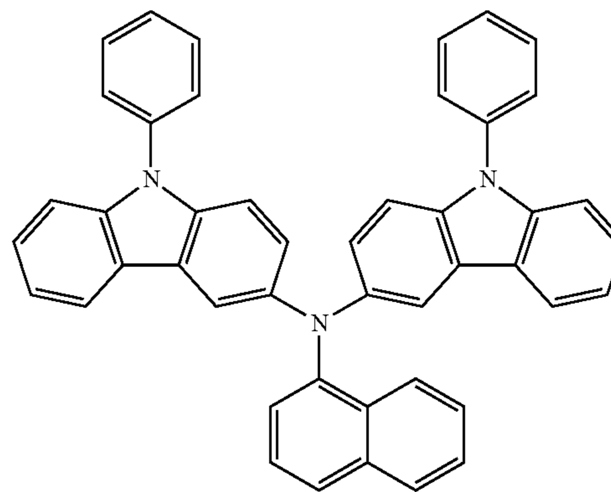
PCzPCN1
