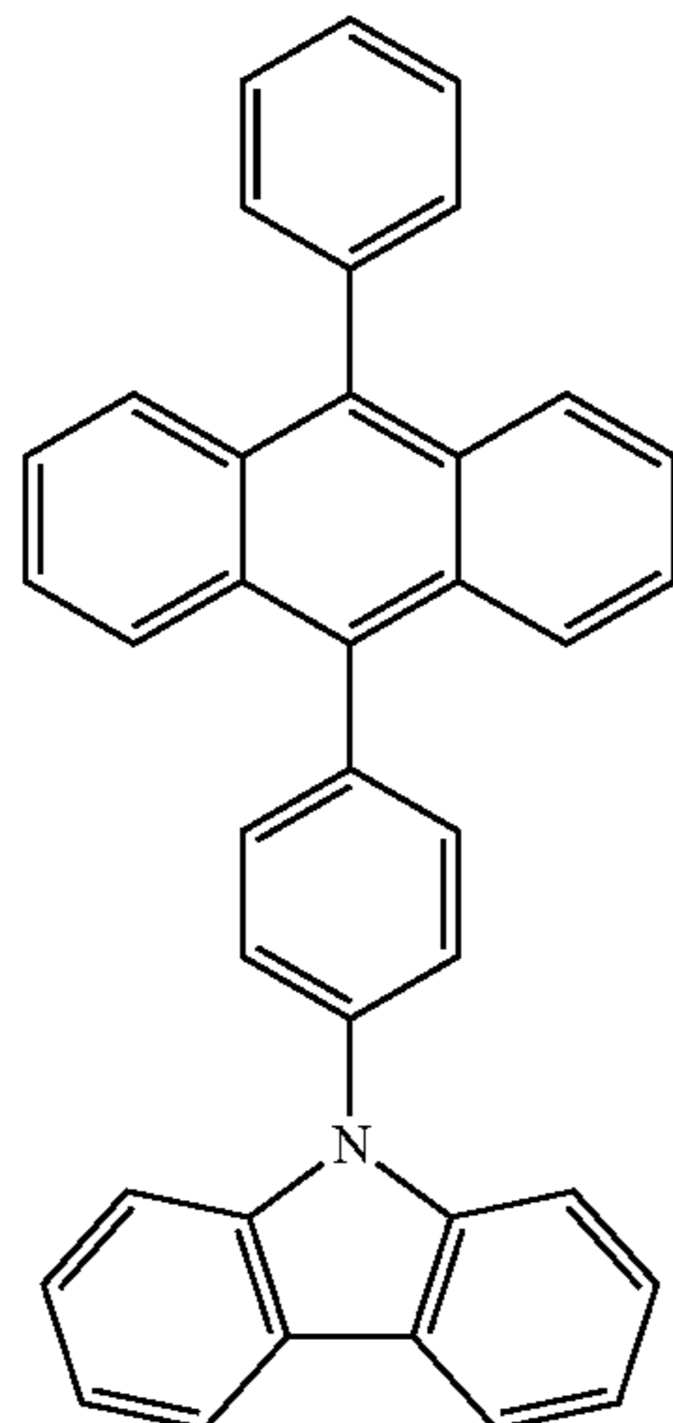
CzPA
