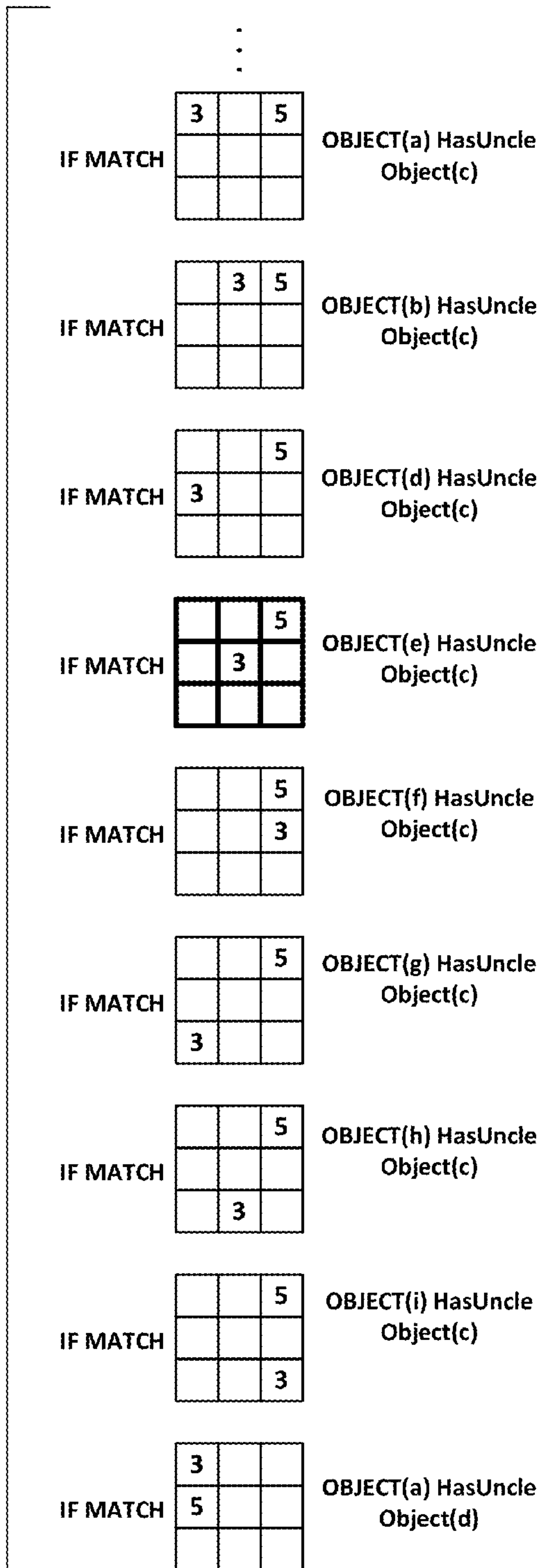
FIG. 26 – PREDICATE TEMPLATES
