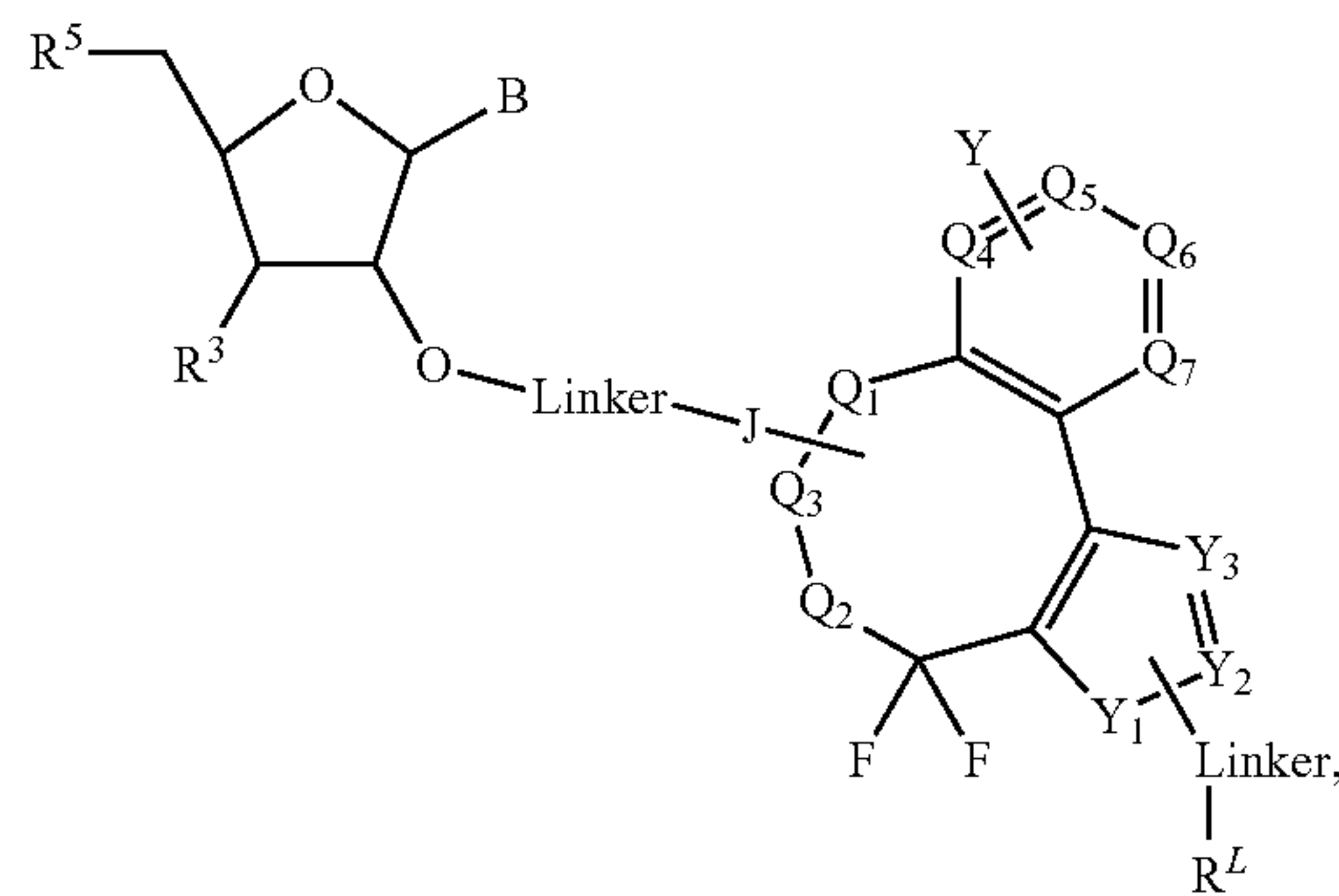
Formula (Va)
