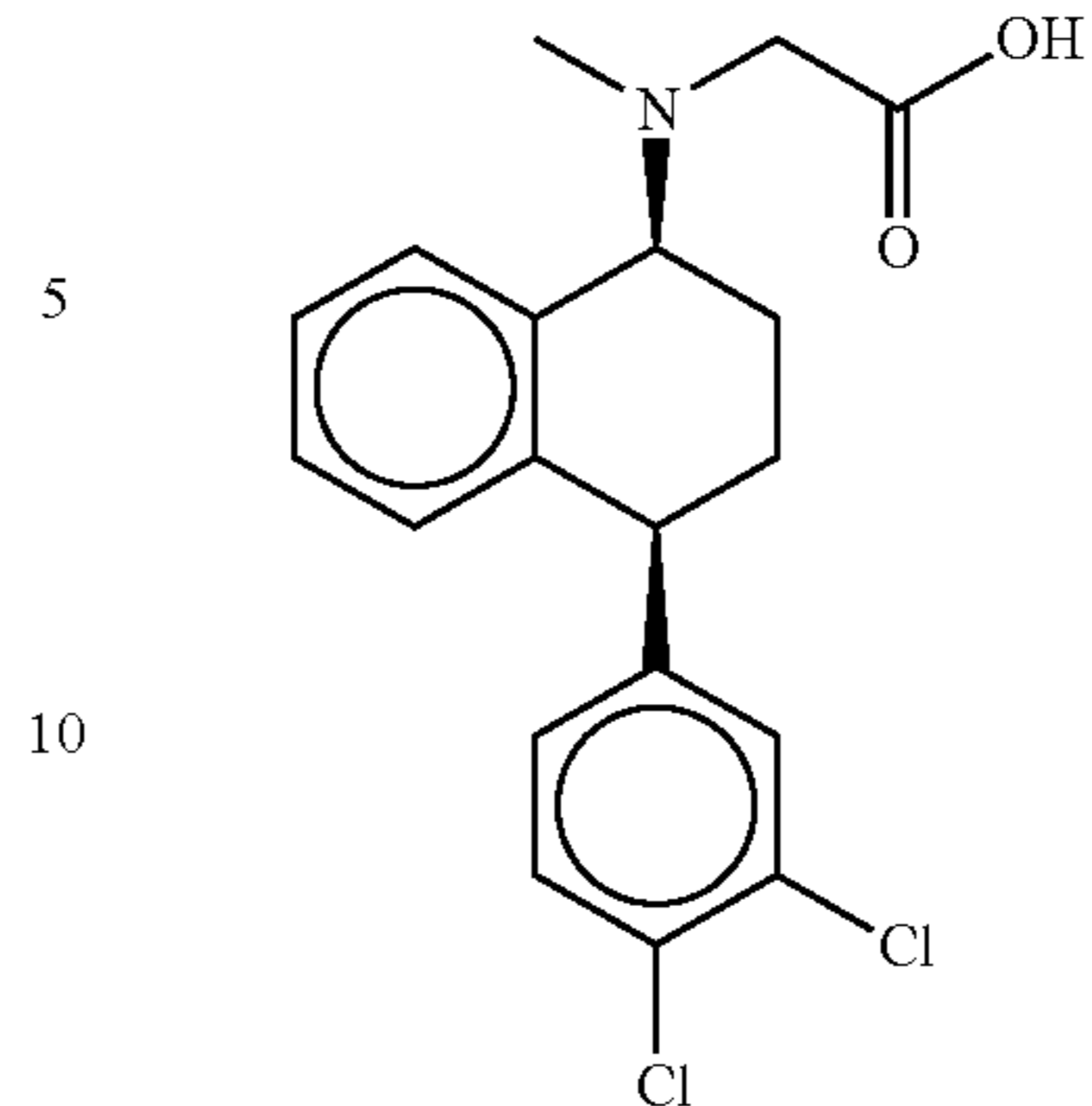
Sertraline-CME
